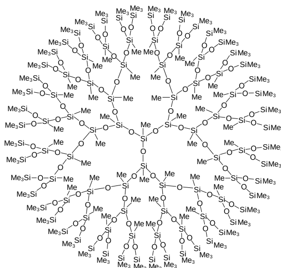
Рис.1. полиметилсилсесквиоксановый дендример 4-ой генерации
