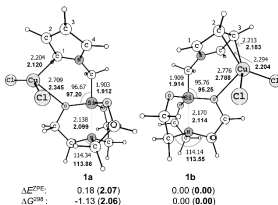
Рис. 1. UPBE0/6-311+G(d,p) оптимизированная геометрия и относительная энергетика изомеров a и b комплекса 1\cdot\text{CuCl}_2 в газовой фазе и растворе ДМСО (жирный шрифт, С-РСМ модель). Связевые расстояния приведены в Å, углы в град., энергии в ккал/моль
