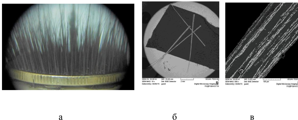
Рис. 1. Оптическое (а) и СЭМ (б, в) изображение пучка (а) и срезанных (б, в) игл.
