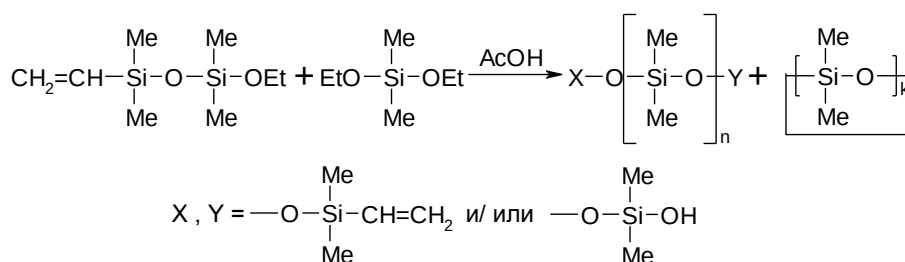
Рис. 1. Схема поликонденсации этоксивинилтетраметилдисилогана и диметилдиэтоксисилана в условиях активной среды.
