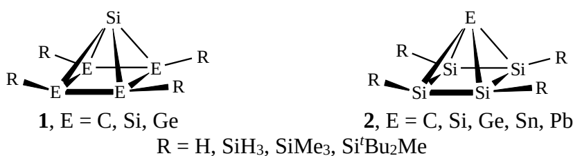
Схема 1. Кремнийсодержащие пирамиданы.
