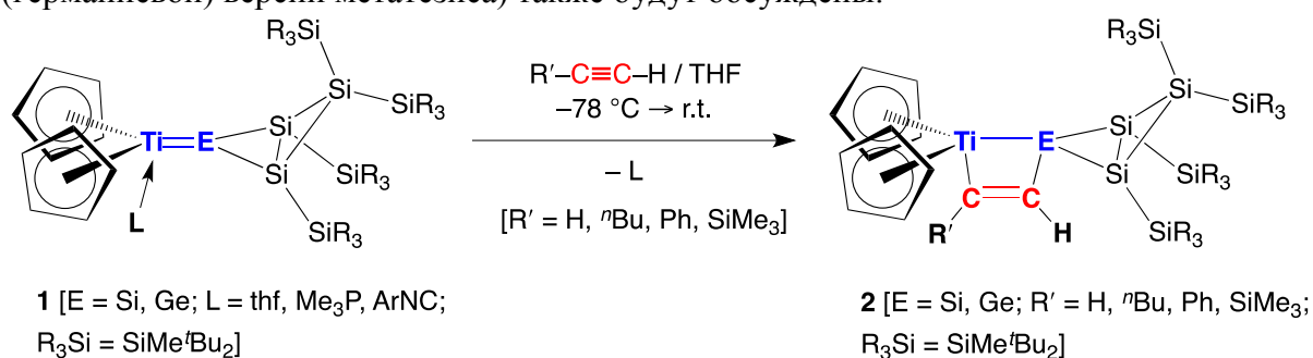
Рис. 1. Получение сила(герма)титанациклбутенов 2 из Шроковских силилиденовых(гермилиденовых) комплексов титана 1 .
