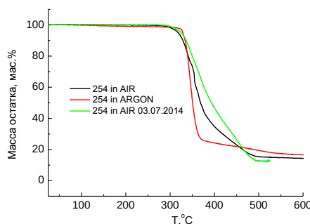
Рис.1 Термогравиметрические кривые полимера Ф-39.
