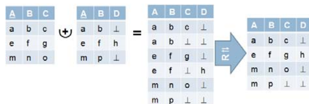
Рис. 3. Пример операции Complementation Union
