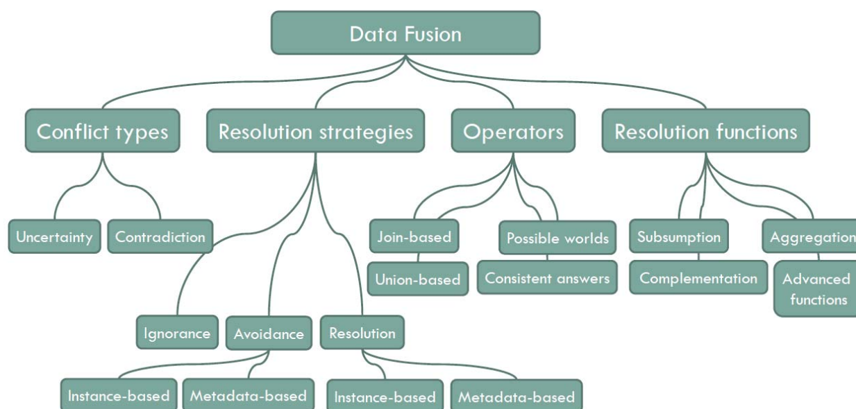
Рис. 1. Различные аспекты проблемы слияния данных
