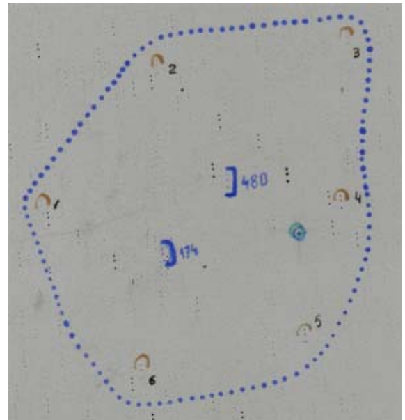
Рис. 2. Фрагмент фотопластинки астрографа с изображениями астероидов
