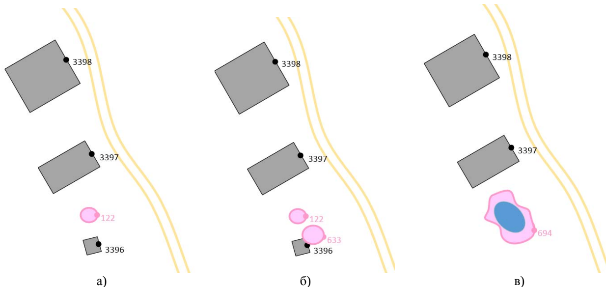
Рис. 1. Пример эволюции карстовых форм на карте: а – одна карстовая форма; б – появление второй карстовой формы с частичным разрушением объекта; в – объединение карстовых форм в одну с частичным заполнением водой
