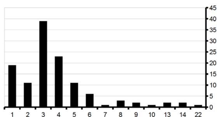
Рисунок 6. Гистограмма распределения числа провинций по кланам
