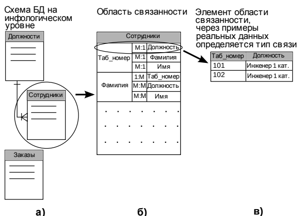
Рис. 2. Определение связи между атрибутами Таб_Номер и Должность через использование двухстрочного отношения: а) схема БД на инфологическом уровне; б) детализирована область связности Сотрудники ; в) детализирован элемент связности Таб_Номер – Должность области связности Сотрудники , связь между атрибутами которого определяется через использование двухстрочного отношения, заполненного реальными данными
