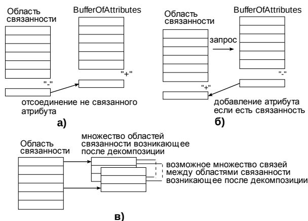
Рис. 3 Операции, производимые над областями связности: а) DeleteAttributeOperation, б) AddAttributeOperation, в) DecompositionOperation
