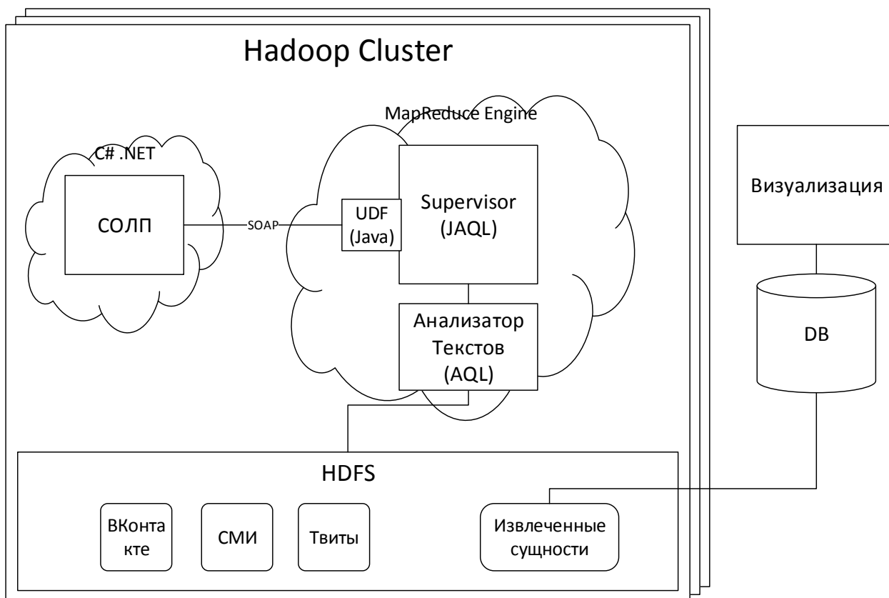
Рис. 2. Архитектура средств извлечения и анализа сущностей в среде Hadoop
