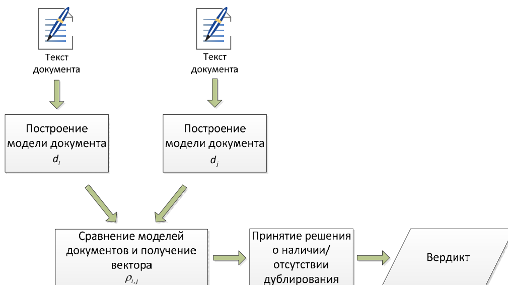
Рис. 2. Этапы обнаружения дубликатов
