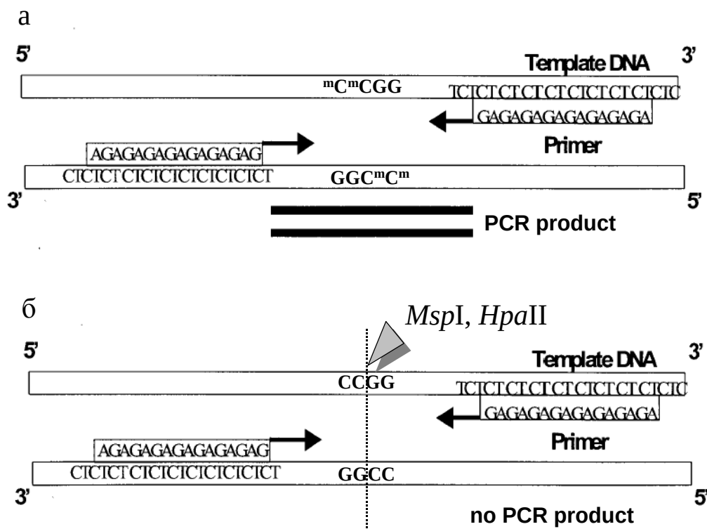
Рис. 1. Принцип MS-ISSR (methylation-sensitive ISSR). Альтернативные варианты ISSR–ПЦР при использовании в качестве матрицы ДНК, предварительно инкубированной с MspI или HpaII : а – метилированный сайт рестрикции 5'- m C m CGG не разрезается MspI или HpaII , ПЦР-фрагмент амплифицируется, б – деметилированный сайт 5'-CCGG служит мишенью для MspI или HpaII , ДНК-матрица разрезается, ПЦР-фрагмент не амплифицируется. Схема ISSR по Pradeep Reddy et al. (2002).
