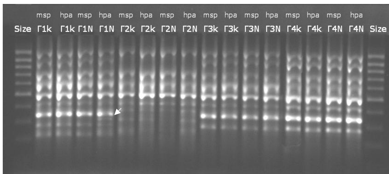
Рис.3. Электрофореграмма ПЦР-фрагментов, полученных методом MS-ISSR для сортов груши (Г1–Г4, табл. 3): k – контроль, N – после криоконсервации; msp – ДНК перед проведением ПЦР обработана Msp I, hpa – Hpa II. Белой стрелкой обозначен выявленный случай метилирования ДНК у сорта Нежность (Г1): ПЦР-фрагмент не амплифицируется до замораживания образца, но присутствует после (М–Н–/М–Н+).
