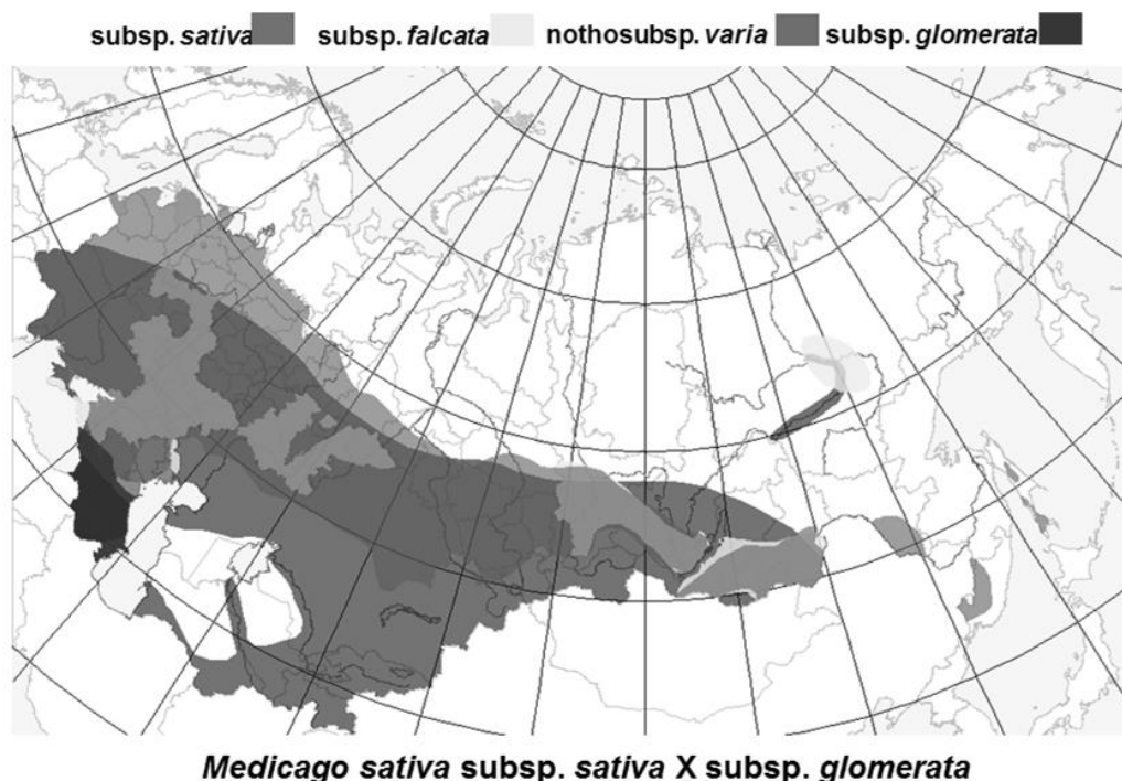
Рис. 10. Использование GAP анализа в мобилизации и сохранении ГРП
