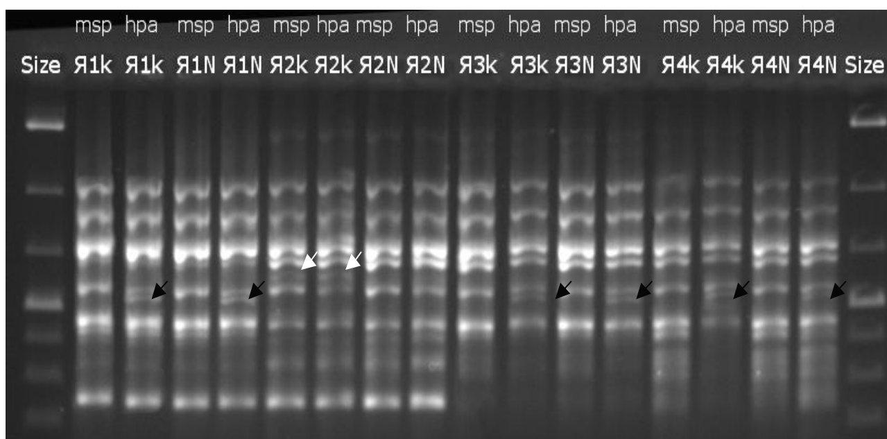
Рис. 2. Электрофореграмма ПЦР-фрагментов, полученных методом MS-ISSR для сортов яблони (Я1–Я4, табл. 3): к – контроль, N – после криоконсервации; msp – ДНК перед проведением ПЦР обработана MspI , hpa – HpaII . Белой стрелкой обозначен выявленный случай деметилирования ДНК у сорта Я2: ПЦР-фрагмент амплифицируется до замораживания образца, но отсутствует после (М+Н+/М–Н–). Черными стрелками обозначен выявленный профиль метилирования ДНК (М–Н+/М–Н+) у сортов яблони Я1, Я3, Я4, не изменяющийся при криоконсервации.
