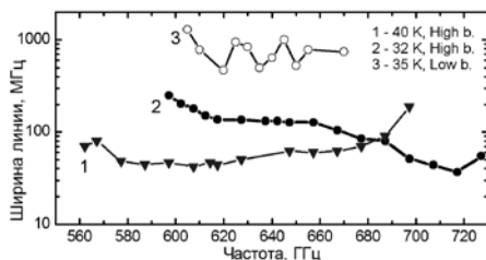
Рис. 1. Зависимость ширины линии излучения генератора от частоты при различных температурах и в различных режимах:
