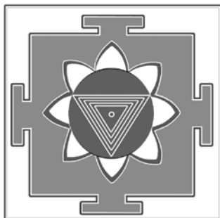
Рисунок 71. Мандала, янтра.
