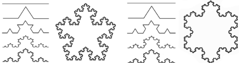
Рисунок 66. Фрактал «Снежинка Коха».
