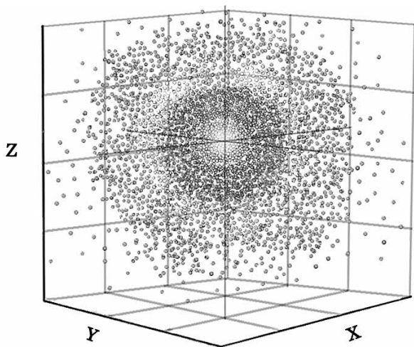
Рисунок 2. Электронное облако атома водорода: часть трёхмерного пространства вокруг ядра атома, где сохраняется наибольшая вероятность местонахождения электрона.
