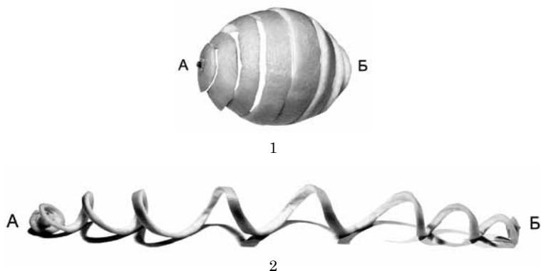
Рисунок 4. Образный пример преобразования электрона из частицы в волну:
