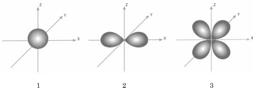
Рисунок 3. Различные формы электронного облака («геометрия» квантовой химии):
