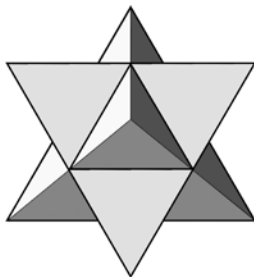
Рисунок 61. Звёздчатый октаэдр Леонардо да Винчи.
