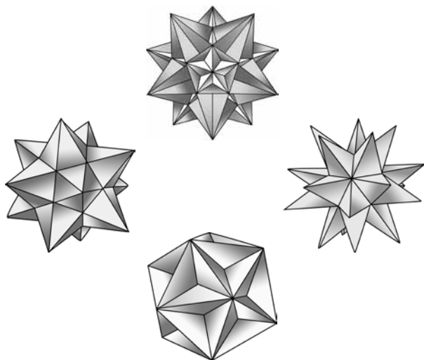
Рисунок 62. Звёздчатые многогранники: тела Кеплера-Пуансо.
