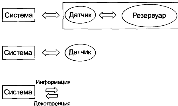
Рис. А.2. Обратимая (в середине) и необратимая (вверху) декогеренция. Необратимость возникает в случае, если окружение системы, вызывающее ее декогеренцию, содержит макроскопическую часть (резервуар), так как огромное число степеней свободы резервуара невозможно контролировать так, чтобы обратить процесс. Декогеренция зависит от информации о системе, которая уходит в окружение, что феноменологически описывается операцией редукции (нижняя часть рисунка).
