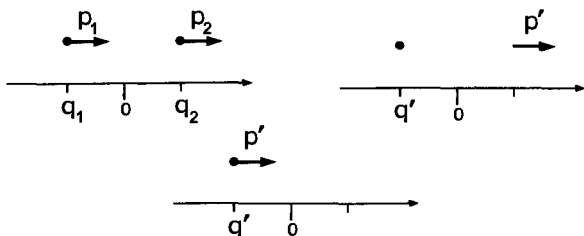
Рис. 1.7. Парадокс Эйнштейна–Подольского–Розена. Перед измерением q_2 = -q_1 , p_2 = p_1 ; измерение дает q_1 = q' , p_2 = p' . В результате координата и импульс первой частицы точно известны: q_1 = q' , p_1 = p' . Но это невозможно в силу принципа неопределенностей.
