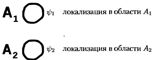
Рис. 4.1. Измерение, различающее между двумя альтернативными свойствами (например, «находиться в области A_1 » и «находиться в области A_2 »). Перед измерением квантовой системы могло не существовать ни одного из этих свойств (если система находилась в состоянии c_1\psi_1 + c_2\psi_2 ).
