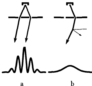
Рис. А.4. Двухщелевой эксперимент и эксперимент типа Который Путь. При пролете электрона через две щели в непрозрачном экране возникает интерференционная картина. Она исчезает, если на пути электрона имеется устройство, дающее информацию о том, через какую щель он пролетел.
