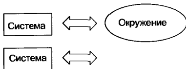
Рис. А.1. Разные способы описания взаимодействия: взаимодействие измеряемой системы с прибором, или окружением, (вверху) или редукция состояния измеряемой системы (внизу). В последнем случае влияние прибора (окружения) учитывается неявно, феноменологически.
