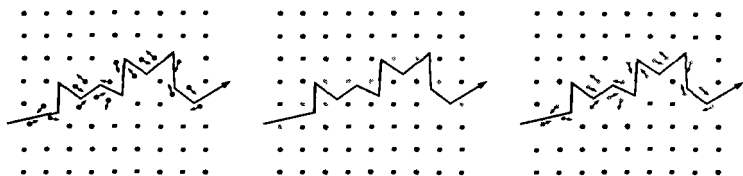
Рис. А.3. Квантовая диффузия. Частица, пролетая через среду, состоящую из атомов, оставляет в ней свой след: ближайшие к ней атомы смещаются (на рисунке слева), или переходят в возбужденное состояние (в середине), или возникают оба эффекта (справа).
