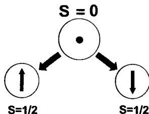
Рис. В.1. ЭПР эффект. Две частицы спина 1/2 возникают при распаде частицы спина 0 . Вследствие этого проекции спинов двух частиц коррелированы, в том числе проекции на одну и ту же ось противоположны.
