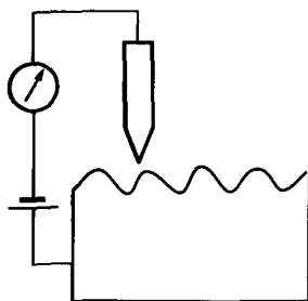
Рис. 2.2. Схема работы сканирующего микроскопа. Острый электрод помещается над определенной точкой образца, и на электрод подается постоянное напряжение. Туннельный ток между этим электродом и образцом зависит от расстояния между электродом и ближайшей к нему точкой образца. Изменение положения электрода (сканирование поверхности образца) и измерение тока позволяет определить форму поверхности с точностью до размера атома.
