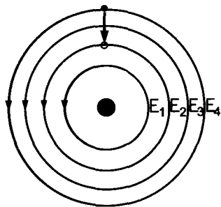
Рис. 1.3. Модель атома, предложенная Бором. Электрон сколь угодно долго может находиться на любой из стационарных орбит, соответствующих определенным уровням энергии E_n . При переходе между двумя уровнями E' и E'' испускается квант света, энергия которого h\nu равна разности энергий этих уровней E' - E'' . На рисунке — переход между уровнями E_4 и E_2 , соответствующий второй линии серии Бальмера.
