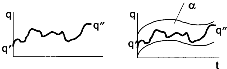
Рис. А.5. Описание непрерывного измерения ограниченным интегралом по путям. Эволюция системы вдоль определенного пути представляется амплитудой, зависящей от этого пути. Эволюция изолированной системы представляется суммой таких амплитуд, то есть интегралом по всем путям (слева). Эволюция непрерывно измеряемой системы представляется интегралом по путям, лежащим в определенном коридоре \alpha . Этот коридор представляет результат непрерывного измерения, например, слежения (с конечной точностью) за координатой системы.
