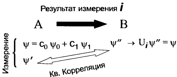
Рис. 2.4. Квантовая телепортация. В точке A имеется два кубита: основной в произвольном (и неизвестном) состоянии \psi и вспомогательный, который коррелирован с кубитом в точке B . Задача — перевести кубит в точке B в состояние \psi . Для этого производится измерение пары кубитов в точке A . Результат измерения i пересылается в точку B , где над имеющимся там кубитом производится преобразование U_i , зависящее от этого результата. Тогда этот кубит оказывается в состоянии \psi .
