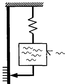
Рис. 1.6. Мысленный эксперимент Эйнштейна, якобы опровергающий соотношение неопределенности \Delta E \Delta T > h . Фотоны, находящиеся в ящике, взвешиваются, затем открывается дверца и один фотон выпускается, после чего взвешивание повторяется. По разности полученных масс энергия одного фотона находится с помощью формулы E = mc^2 .
