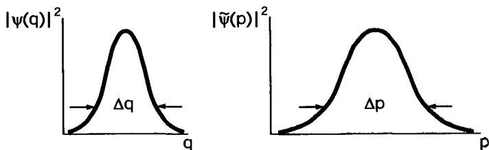
Рис. 1.5. Вероятностная интерпретация волновой функции. В координатном представлении: |\psi(q)|^2 — плотность вероятности нахождения частицы в точке q . С большой вероятностью частица находится в области размером \Delta q (неопределенность координаты). В импульсном представлении: |\tilde{\psi}(p)|^2 — плотность вероятности того, что частица имеет импульс p . С большой вероятностью импульс частицы принадлежит области размером \Delta p (неопределенность импульса).
