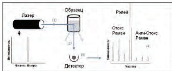
Рис. 1. Релейные и рамановские спектры.
