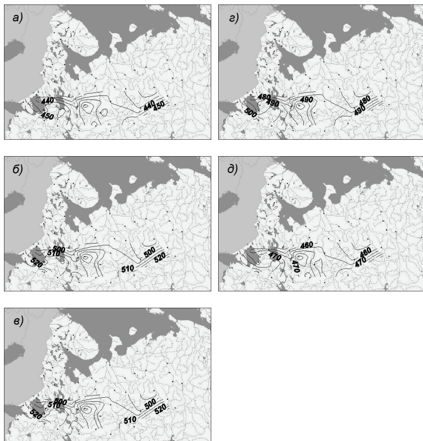
Рис. 4.22. Испарение с ельника III класса бонитета (а – 20 лет, б – 40 лет, в – 60 лет, г – 80 лет, д – 100 лет)
