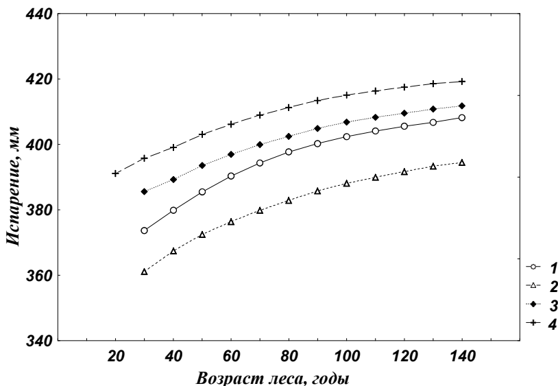
Рис. 4.14. Испарение с сосняка сфагнового (Va класс бонитета) при среднегодовой температуре воздуха 2.4 °C (1), 1.4 °C (2), 3.4 °C (3), 4.4 °C (4)
