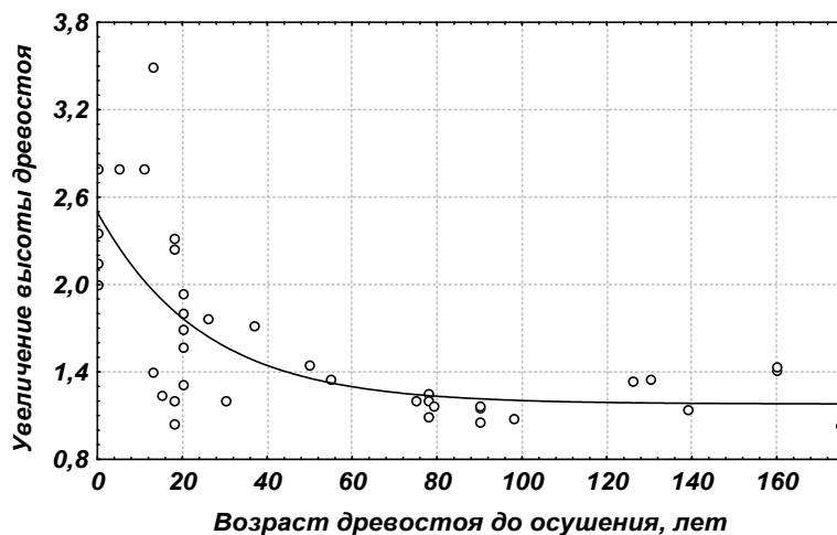
Рис. 1.3. Зависимость прироста древостоя в высоту в результате мелиорации (отношение измеренной высоты древостоя после мелиорации к его высоте в естественных условиях) от возраста до осушения
