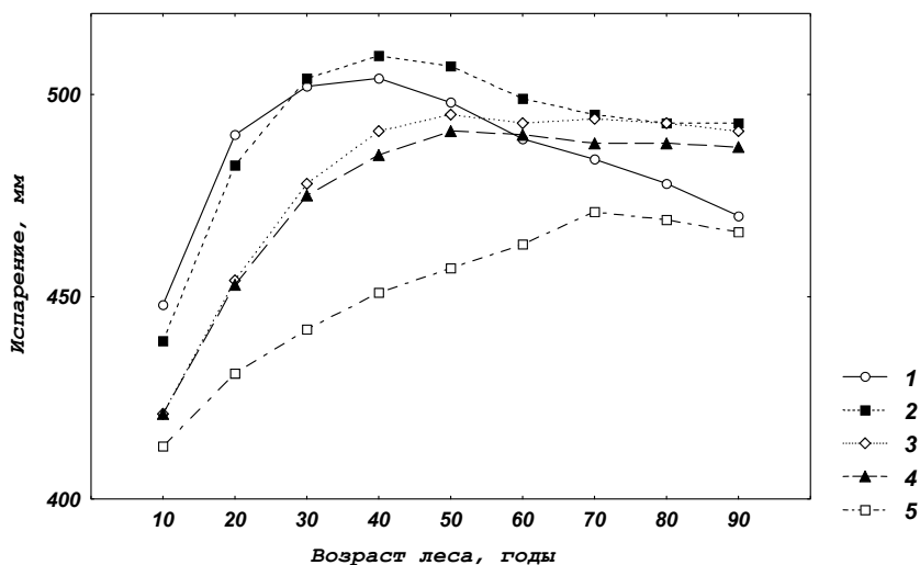
Рис. 4.6. Среднее многолетнее годовое испарение с березняков южной подзоны тайги (1 – кисличный I кл. бонитета, 2 – черничный II кл. бонитета, 3 – черничный III кл. бонитета, 4 – долгомошно-черничный III кл. бонитета, 5 – травяно-сфагновый IV кл. бонитета)
