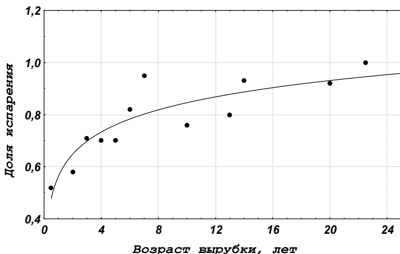
Рис. 2.1. Зависимость относительной величины испарения (относительно спелого леса) от возраста вырубki
