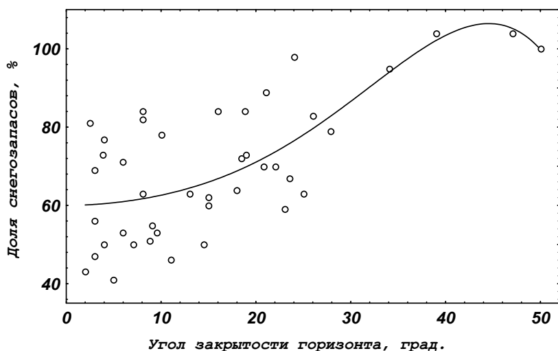
Рис. 4.26. Зависимость снегозапасов на поляне от угла закрытости горизонта
