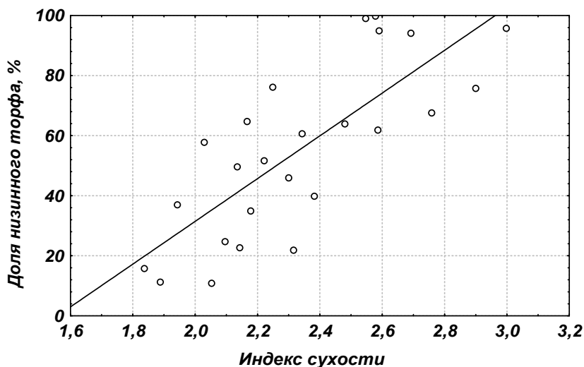
Рис. 1.2. Зависимость доли низинного торфа в регионе от климатического фактора
