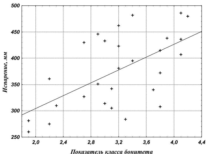
Рис. 4.3. Зависимость суммарного испарения с лесного водосбора от продуктивности леса
