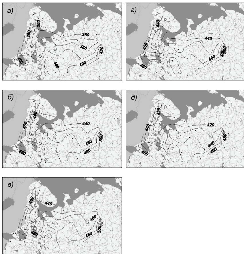
Рис. 4.23. Испарение с ельника IV класса бонитета (а – 20 лет, б – 40 лет, в – 60 лет, з – 80 лет, д – 100 лет)
