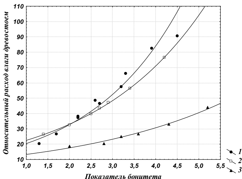
Рис. 3.3. Зависимость относительного расхода воды (отношение удельного расхода воды для прироста к удельному расходу воды для поддержания жизнедеятельности) для прироста единицы фитомассы от показателя бонитета (1 – сосна, 2 – ель, 3 – береза)
