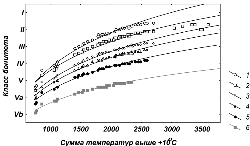
Рис. 1.5. Зависимость производительности сосняков черничного (1), брусничного (2), верескового (3), долгомошного (4), багульникового (5) и сфагнового (6) от суммы температур выше +10^{\circ}\text{C}
