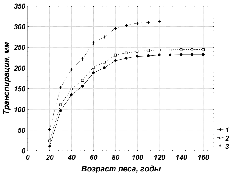
Рис. 4.10. Транспирация сосняка (1), ельника (2) и березняка (3) V класса бонитета
