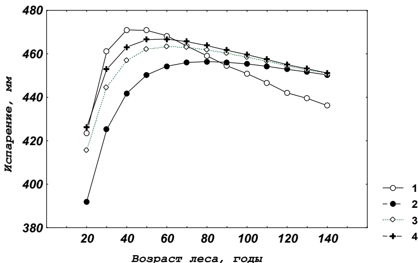
Рис. 4.15. Испарение с сосняка брусничного (III класс бонитета) при среднегодовой температуре воздуха 2.4 °C (1), 1.4 °C (2), 3.4 °C (3), 4.4 °C (4)
