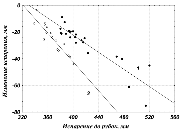
Рис. 4.17. Изменение испарения с леса после рубок ухода в зависимости от начального испарения (1 – сосновый лес, 2 – еловый лес)
