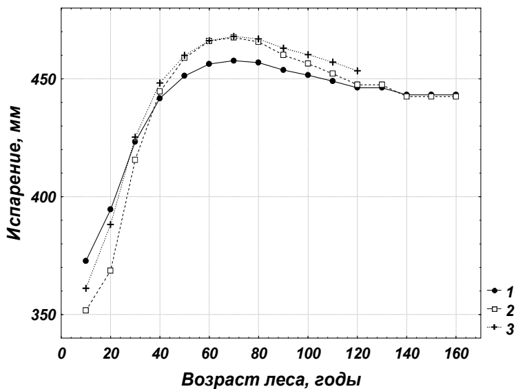
Рис. 4.12. Суммарное испарение с сосняка (1), ельника (2) и березняка (3) III класса бонитета
