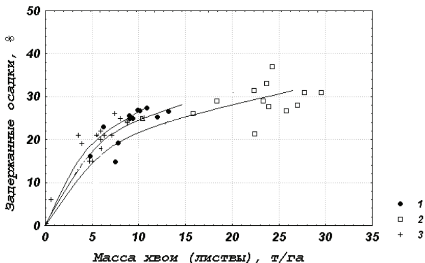
Рис. 3.5. Зависимость относительной величины испарения (относительно выпавших осадков) задержанных пологом леса жидких осадков от массы хвои (листвы) (1 — сосновым лесом, 2 — еловым лесом и 3 — березовым лесом)
