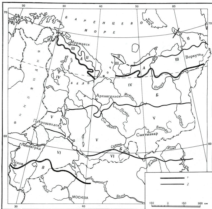
Рис. 1.1. Физико-географическое районирование ЕСР (по [96])
