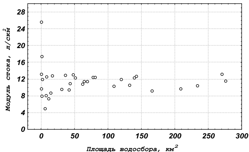
Рис. 2.2. Зависимость модуля стока рек Карелии от площади водосбора
