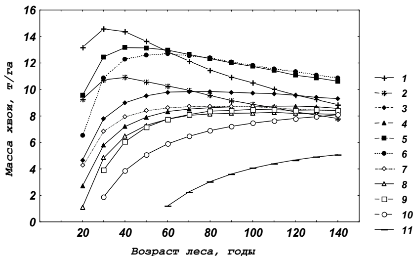
Рис. 4.1. Динамика массы хвои в различных типах сосняков (1 – черничный II класса бонитета, 2 – черничный III класса бонитета, 3 – черничный IV класса бонитета, 4 – черничный V класса бонитета, 5 – брусничный III класса бонитета, 6 – брусничный IV класса бонитета, 7 – брусничный V класса бонитета, 8 – лишайниковый V класса бонитета, 9 – сфагновый V класса бонитета, 10 – сфагновый Va класса бонитета, 11 – сфагновый Vб класса бонитета)
