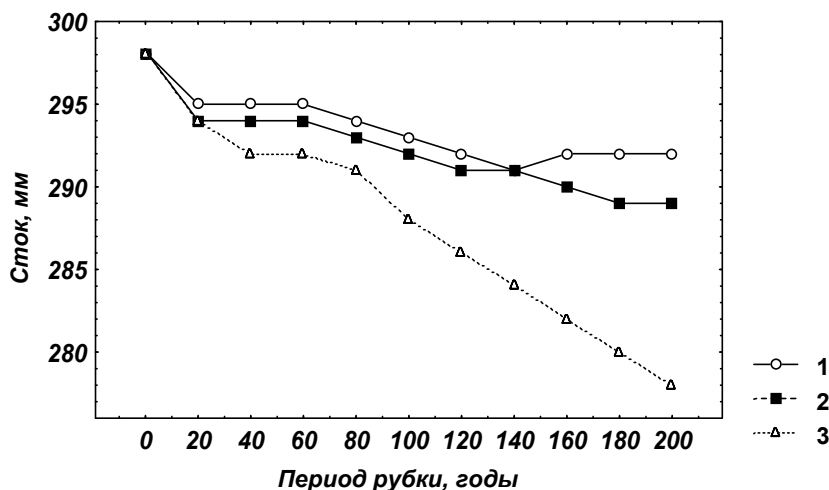
Рис. 6.2. Сток с модельного водосбора: 1 – вырубка леса III–V бонитета в размере расчетной лесосеки, 2 – вырубка леса всех бонитетов в размере расчетной лесосеки, 3 – то же при использовании лесосеки на 66% [17]
