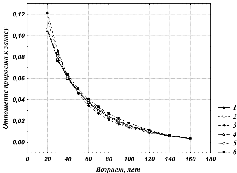
Рис. 1.4. Зависимость относительной величины текущего прироста к запасу от возраста для различных типов ельников (1 – брусничный, 2 – черничный свежий, 3 – кисличный, 4 – черничный влажный, 5 – болотно-травяной, 6 – долгомошный)
