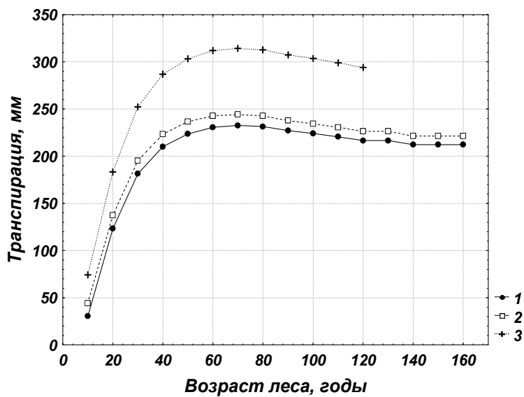
Рис. 4.9. Транспирация сосняка (1), ельника (2) и березняка (3) III класса бонитета
