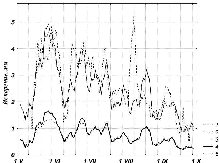
Рис. 3.4. Временной ход суммарного испарения с леса (1, 3), транспирации (2, 4) и испарения с открытой водной поверхности (5) (скользящее осреднение с шагом 5 суток) при g_s = f(d) (1, 2) и g_s = \text{const} (3, 4)
