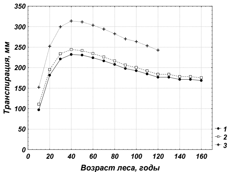
Рис. 4.8. Транспирация сосняка (1), ельника (2) и березняка (3) I класса бонитета
