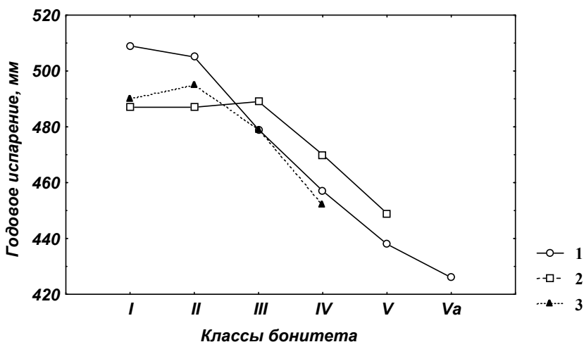
Рис. 4.7. Зависимость испарения от классов бонитета для различных пород древостоя (1 – сосна, 2 – ель, 3 – береза)
