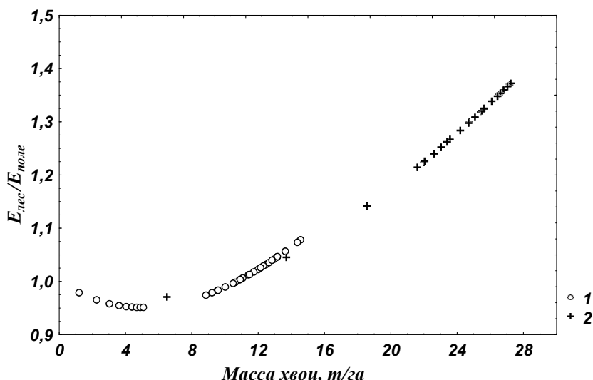
Рис. 4.27. Зависимость соотношений испарения с хвойного леса и поля от массы хвои (1 – сосновый лес, 2 – еловый лес)
