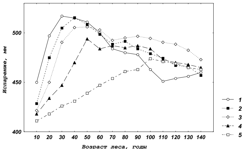
Рис. 4.5. Среднее многолетнее годовое испарение с ельников южной подзоны тайги (1 – кисличный I кл. бонитета, 2 – черничный II кл. бонитета, 3 – черничный III кл. бонитета, 4 – сфагново-черничный IV кл. бонитета, 5 – травяно-сфагновый V кл. бонитета)
