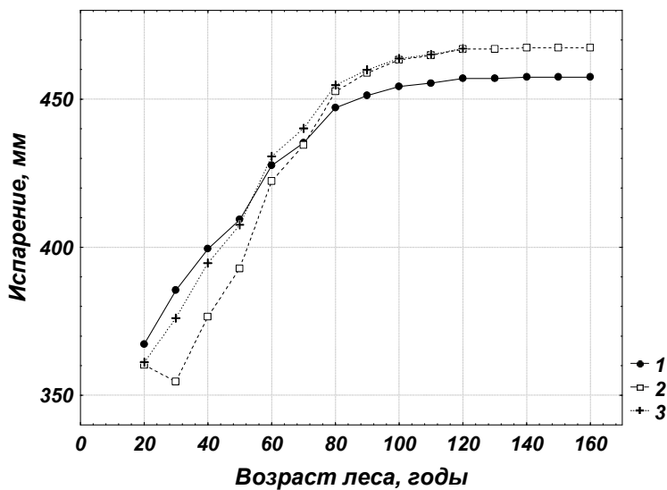
Рис. 4.13. Суммарное испарение с сосняка (1), ельника (2) и березняка (3) V класса бонитета
