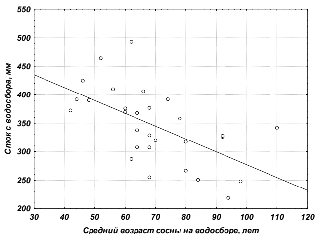
Рис. 6.1. Зависимость стока от среднего возраста сосны на водосборе
