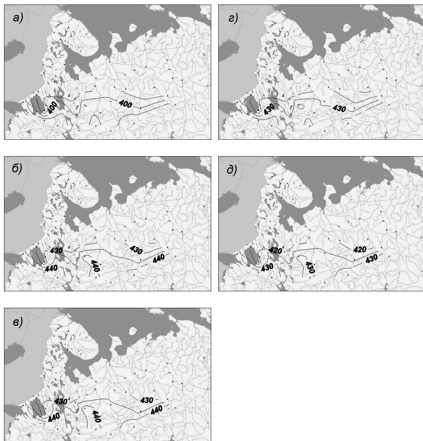
Рис. 4.25. Испарение с березняка II–III класса бонитета (а – 20 лет, б – 40 лет, в – 60 лет, г – 80 лет, д – 100 лет)
