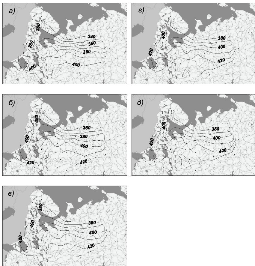
Рис. 4.21. Испарение с сосняка V класса бонитета (а – 20 лет, б – 40 лет, в – 60 лет, г – 80 лет, д – 100 лет)
