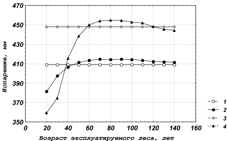
Рис. 4.18. Возрастные изменения суммарного испарения с эксплуатируемых сосняка брусничного (2) и ельника черничного (4) (для сравнения показано испарение с коренных сосняка брусничного (1) и ельника черничного (3))
