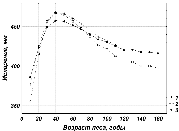
Рис. 4.11. Суммарное испарение с сосняка (1), ельника (2) и березняка (3) I класса бонитета
