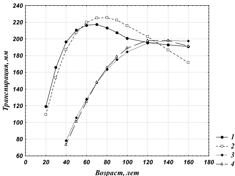
Рис. 3.1. Транспирация сосняком чернично-кисличным (1, 2) и сосняком сфагновым (3, 4), рассчитанная по методу транспирационных коэффициентов (1, 3) и по Хильми (2, 4)
