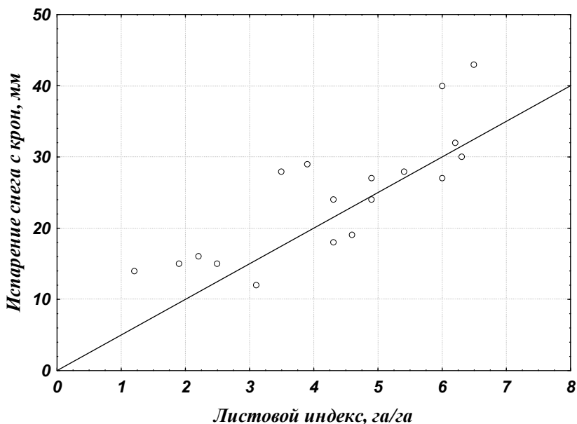
Рис. 3.6. Зависимость испарения снега с крон хвойных деревьев от листового индекса
