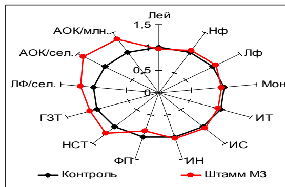
Рис. 2. Влияние штамма M3 Bacillus sp. на структурно-функциональные параметры иммунной системы.
