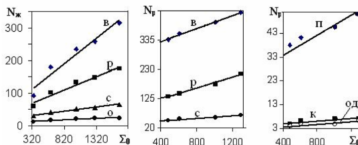
Рис. 4. Графики зависимости N_{ж} и N_{р} в от \Sigma_0 для разных таксонов (буквенные обозначения таксонов – по табл.1-2).
