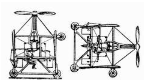
Проект вертолета Николы Теслы.
