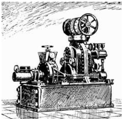
Паровая турбина Теслы мощностью в 1000 лошадиных сил.
