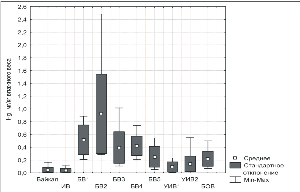
Рис. 7.1.14. Изменение концентраций ртути в мышечной ткани речного окуня в водоемах Байкало-Ангарской водной системы с различной степенью техногенной нагрузки ИВ – Иркутское водохранилище; Братское водохранилище: БВ1 – г. Усолье-Сибирское, БВ2 – о. Конный, БВ3 – Балаганское расширение, БВ4 – средняя часть вдхр., БВ5 – нижняя часть вдхр.; Усть-Илимское водохранилище: УИВ1 – верхняя часть вдхр., УИВ2 – нижняя часть вдхр.; БОВ – район планируемого Богучанского водохранилища. ПДК Hg для хищных рыб – 0,6 мг/кг влажного веса.
