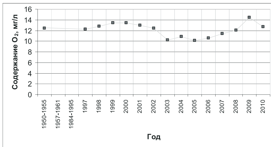
Рис. 7.1.9. Изменение содержания кислорода в воде истока реки Ангары за период 1950-2010 гг.
