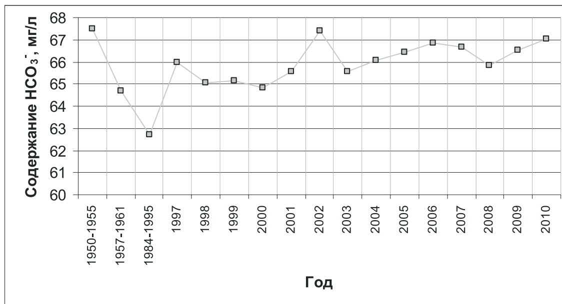
Рис. 7.1.5. Изменение содержания \text{НСО}_3^- в воде истока реки Ангары за период 1950-2010 гг.
