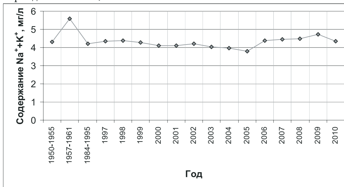
Рис. 7.1.7. Сумма ионов \text{K}^+ и \text{Na}^+ в воде истока реки Ангары за период 1950-2010 гг.
