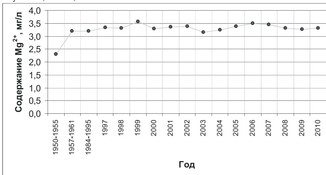
Рис. 7.1.4. Среднее содержание \text{Mg}^{2+} в воде истока реки Ангары
