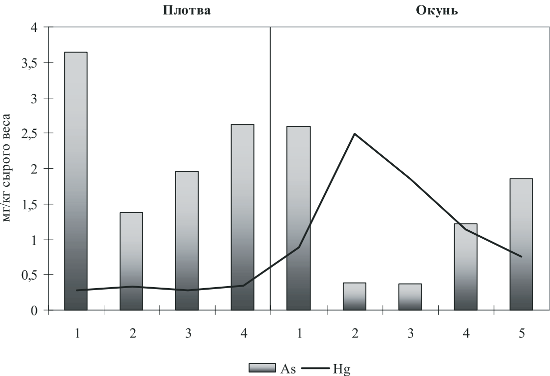
Рис. 7.1.15. Соотношение накопления Hg и As в мышечной ткани плотвы и окуня верхней части Братского водохранилища.
