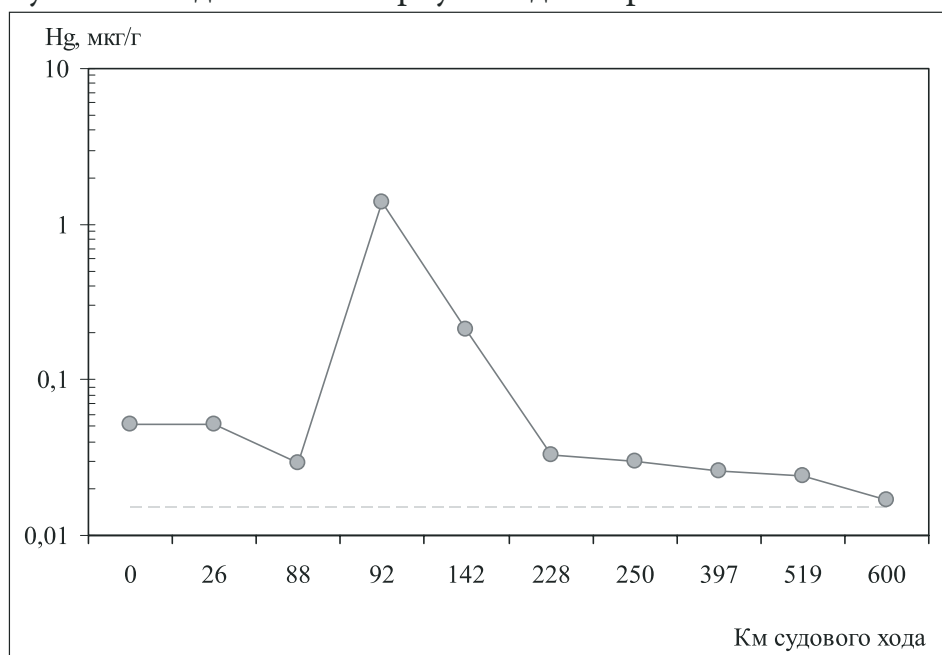
Рис. 7.1.12. Изменение концентраций ртути в рдесте гребенчатом по судовому ходу вниз по течению от г. Иркутска до г. Братск в 2009 г. 92 км судового хода – район выпусков сточных вод УХП.
