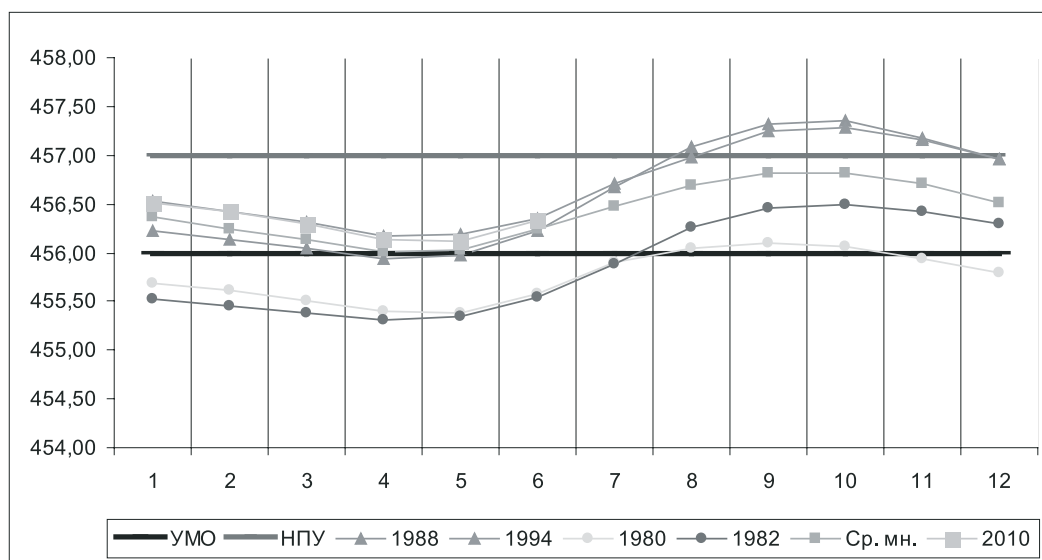
Рис. 4.7.1. Уровни озера Байкал 2010 г. в сравнении с максимальным (1988, 1994), минимальным (1980, 1982), среднемноголетним.
