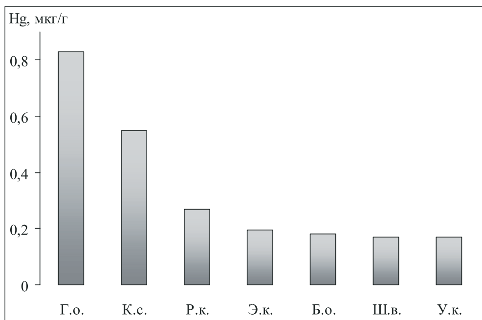
Рис. 7.1.13. Содержание ртути в водных растениях различных экобиоморфологических групп по 2008 г. (45 км ниже выпусков «Усольехимпром»). Г.о. – гигрогипнум охристый, К.с. – кладофора скученная, Р.к. – рдест курчавый, Э.к. – элодея канадская, Б.о. – болотник обоеполый, Ш.в. – шелковник волосистый, У.к. – уруть колосистая.
