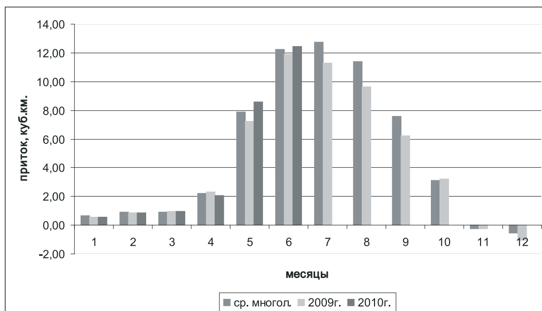
Рис. 4.7.2. Полезный приток в озеро Байкал за 2010 год в сравнении с 2009 г. и среднемноголетним
