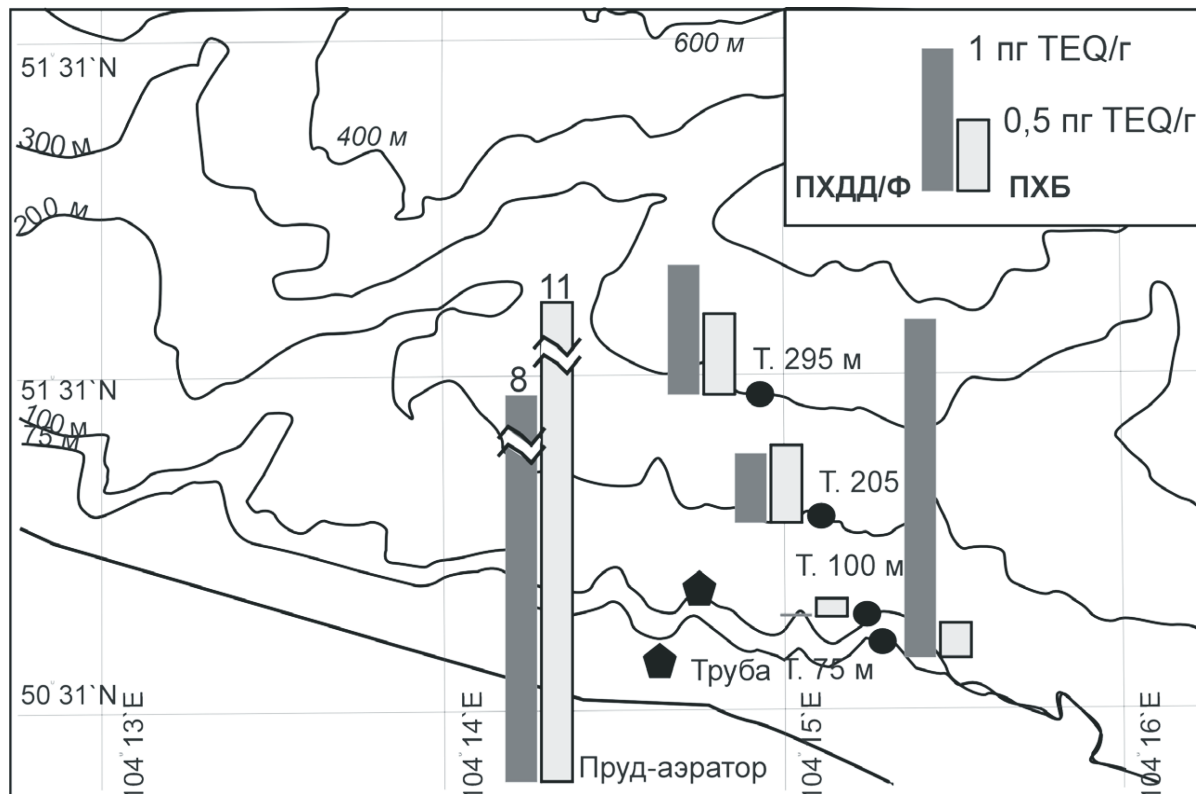
Рис. 7.1.21. Распределение токсического эквивалента (TEQ) ПХДД/Ф и ПХБ в донных отложениях Байкала (pg TEQ-WHO/g сухого веса).
