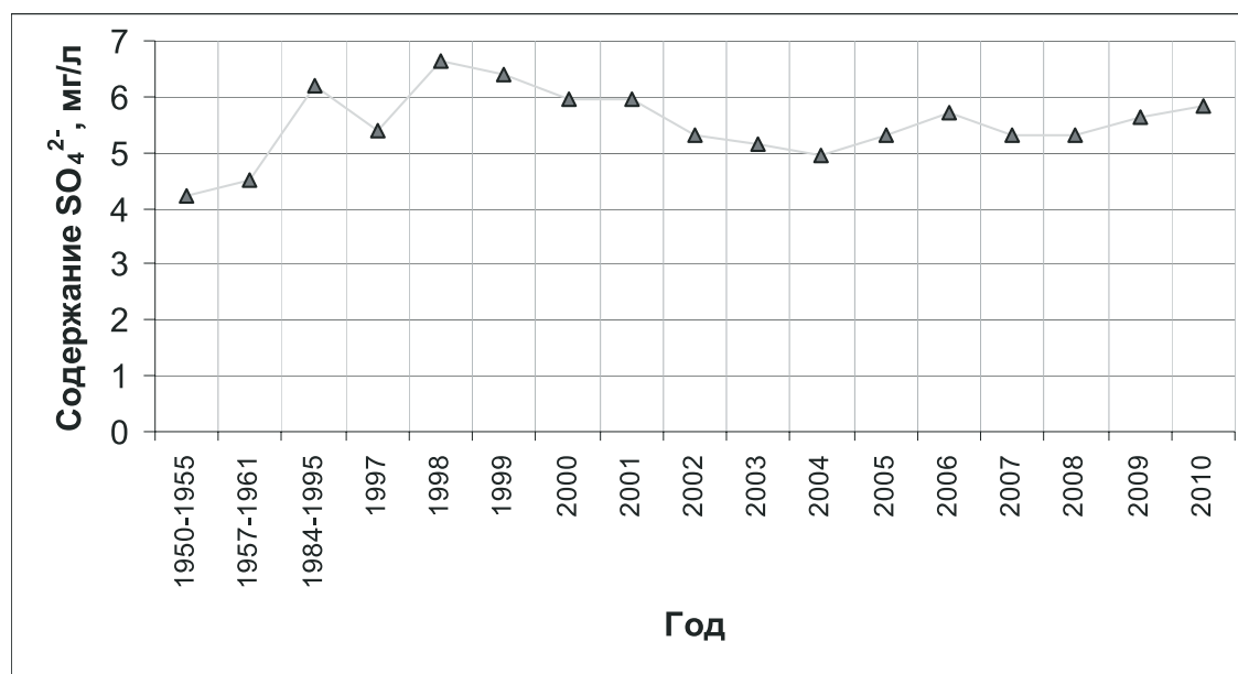
Рис. 7.1.8. Изменение содержания сульфат-иона в воде истока реки Ангары за период 1950-2010 гг.
