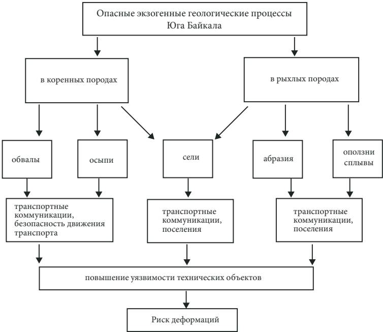
Рис. 7.2.5. Схема экзогеодинамической опасности для территории юга озера Байкал.
