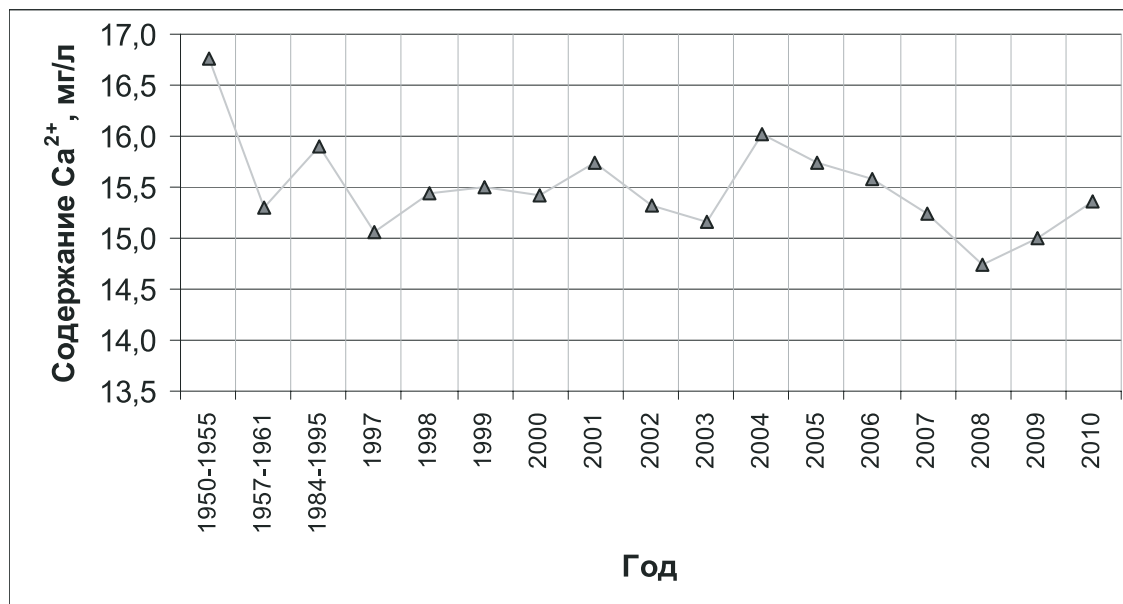
Рис. 7.1.3. Изменение содержания \text{Ca}^{2+} в воде истока реки Ангары за период 1950-2010 гг.
