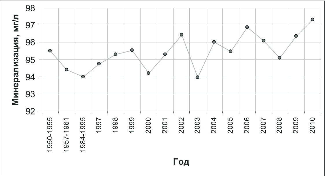
Рис. 7.1.2. Межгодовое изменение минерализации в воде истока реки Ангары за период 1950-2010 гг.
