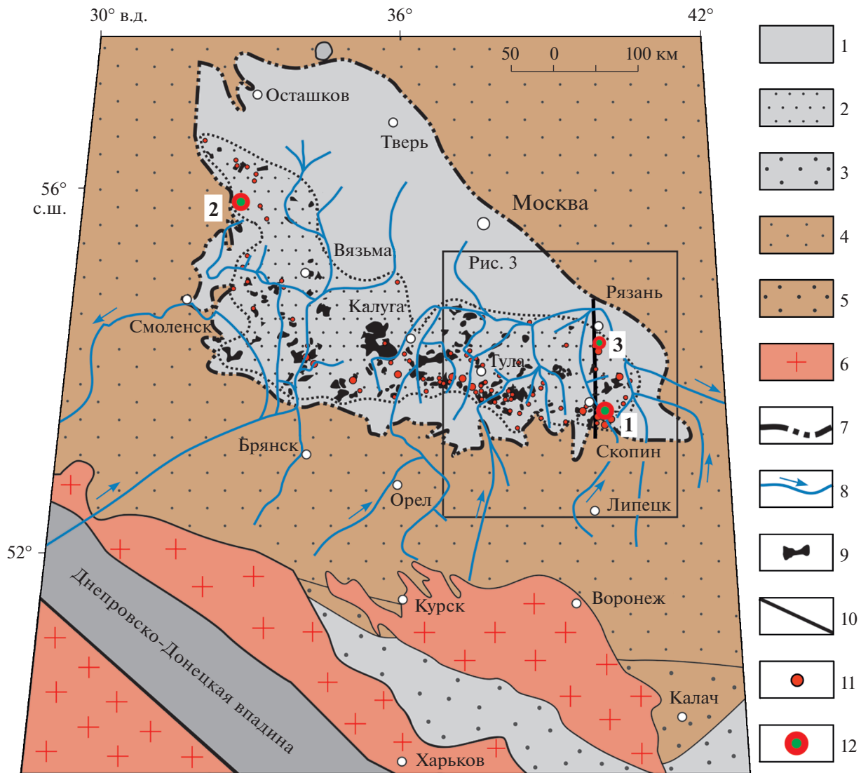
Рис. 2. Палеогеографическая реконструкция центральной части Восточно-Европейской платформы для ранне-средневизейского времени, по [Палеогеоморфологический ..., 1983; Махлина, 1993; Карась и др., 2017] с изменениями. 1–3 – нижне-средневизейские отложения: 1 – преимущественно глинистые (озерные и мелководно-морские фации), 2 – преимущественно песчаные (дельтовые фации бобринских палеорек), 3 – песчаные (фации аллювия); 4 – верхнедевонско-нижнекаменноугольные карбонатно-терригенные отложения в области размыва; 5 – верхнедевонские терригенные отложения (прибрежно-морские фации) в области размыва; 6 – выступы докембрийского кристаллического фундамента в области размыва; 7 – граница визейского Подмосковского буроугольного бассейна; 8 – русла палеорек с направлением течения; 9 – болота (залежи бурого угля); 10 – долгоживущий Двуреченско-Липецкий разлом; 11 – проявления урана; 12 – месторождения с установленной рениевой минерализацией (1 – Брикетно-Желтухинское, 2 – Бельское, 3 – Алексеевское урановорудное проявление).
