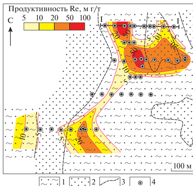
Рис. 4. Изолинии продуктивности рениевого оруденения в бобриковской свите Брикетно-Желтухинского месторождения на литолого-фациальной схеме, с линией разреза I—I', по [Карась и др., 2016, 2017] с изменениями.
