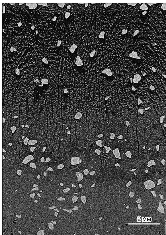
Рис. 4. Вертикальный срез модельной смеси 90 % каолинита и 10 % песка в мерзлом состоянии после однократного промерзания.
