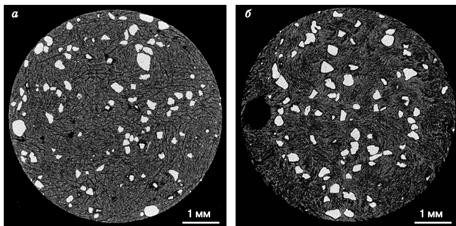
Рис. 5. Распределение песчаных частиц в образце модельной смеси каолинита и песка:
