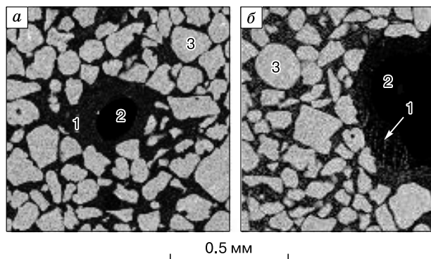
Рис. 2. Микростроение образца кварца с неполным заполнением пор (а) и игольчатый лед-цемент в образце кварца с неполным заполнением пор (б).
