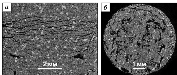
Рис. 3. Криогенные текстуры в образце суглинка.
