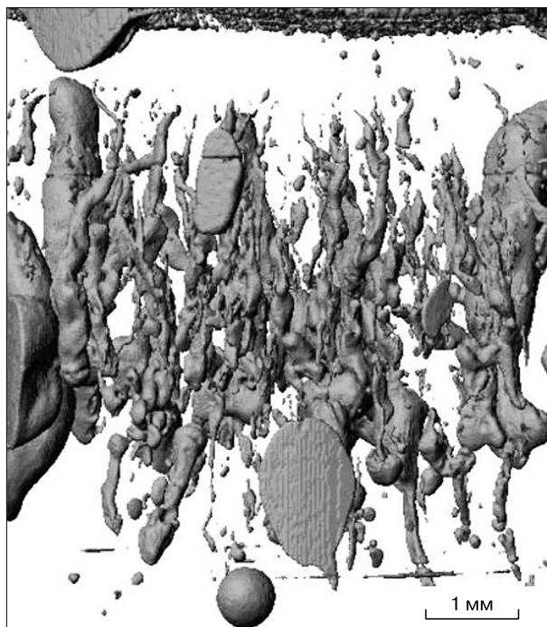
Рис. 1. Распределение пор (серые фигуры) в образце льда.
