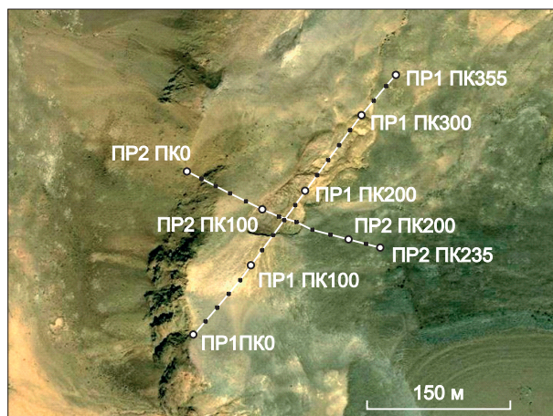
Рис. 5. Схема расположения профилей электротомографии (источник космоснимка – http://www.bing.com/mapspreview ).
