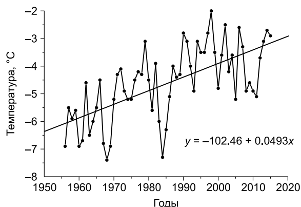
Рис. 11. Среднегодовые температуры воздуха за последние 60 лет и линейная аппроксимация зависимости.
