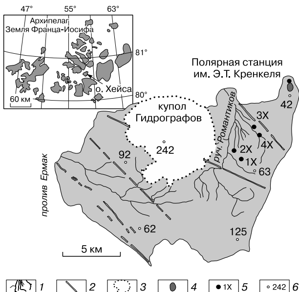
Рис. 1. Схема района исследований.
