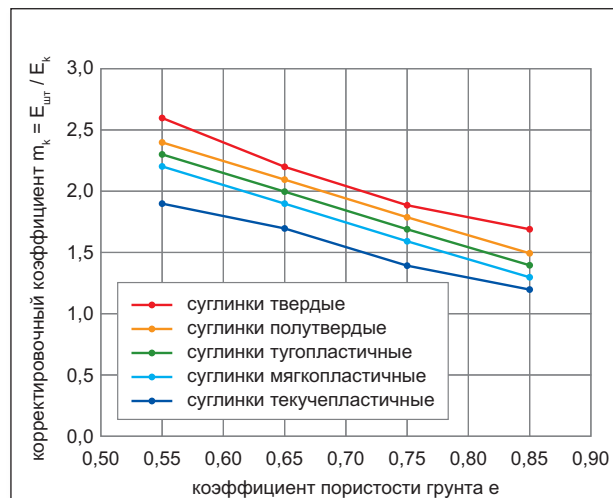
Рис. 4. Графики зависимости корректировочного коэффициента m_k от коэффициента пористости грунта e для суглинков
