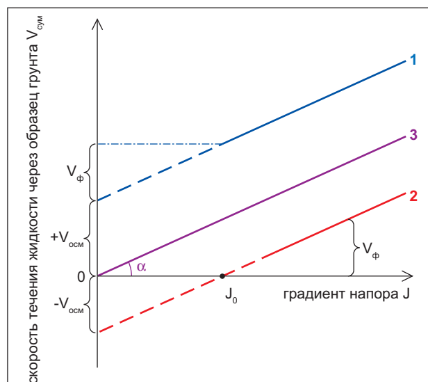
Рис. 2. Графический способ нахождения поправки на скорость и направления осмотического потока в глине при расчете коэффициента фильтрации: 1 — одинаковые направления фильтрационного и осмотического потоков; 2 — встречные направления фильтрационного и осмотического потоков; 3 — зависимость V_{\text{ф}}(J) (объяснения в тексте)
