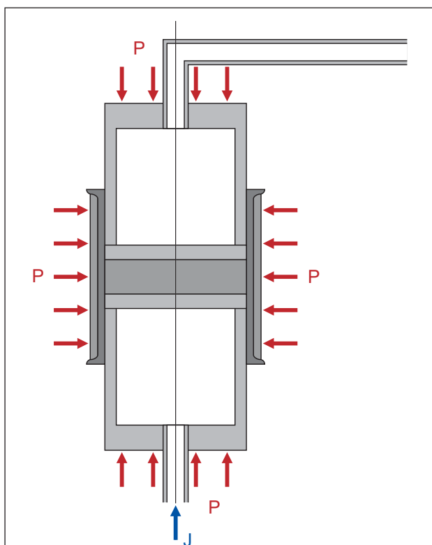
Рис. 1. Схема модернизированного узла с образцом испытываемого грунта в фильтрационном приборе УИПК-1М для одновременного измерения скоростей фильтрационного и капиллярно-осмотического потоков в глинистых грунтах (объяснения в тексте)
