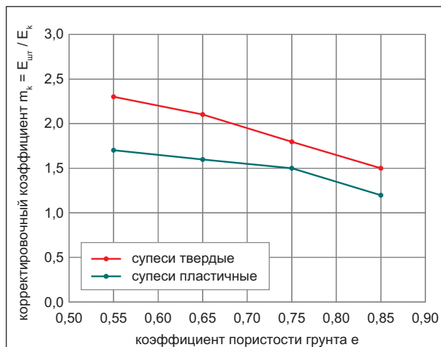
Рис. 3. Графики зависимости корректировочного коэффициента m_k от коэффициента пористости грунта e для супесей
