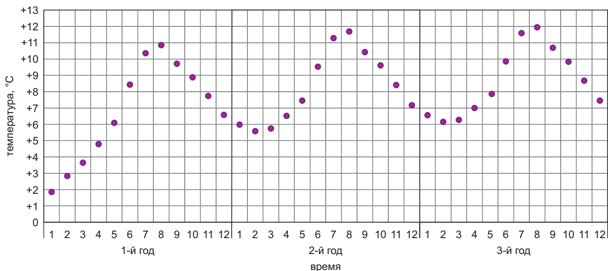
Рис. 5. График сезонного хода температур в пределах дрены (блока 17/8) при температуре внутри сооружения +20°C
