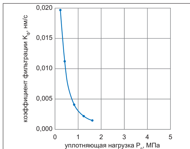
Рис. 3. Зависимость коэффициента фильтрации Са-монтмориллонита K_f от давления предварительного уплотнения P_n
