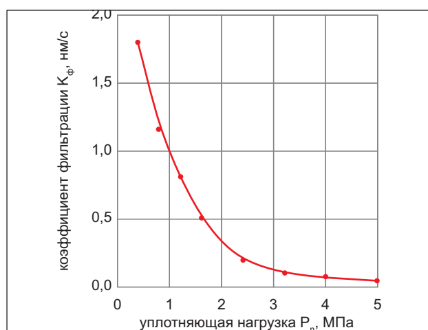
Рис. 4. Зависимость коэффициента фильтрации На-каолинита K_f от давления предварительного уплотнения P_n
