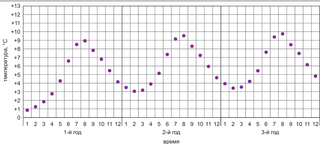
Рис. 4. Графики сезонного хода температур в пределах дрены А при температуре внутри сооружения +15°C
