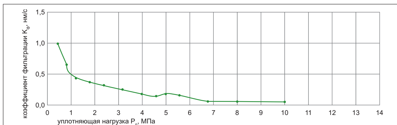
Рис. 5. Зависимость коэффициента фильтрации Са-гидрослюды K_f от давления предварительного уплотнения P_n
