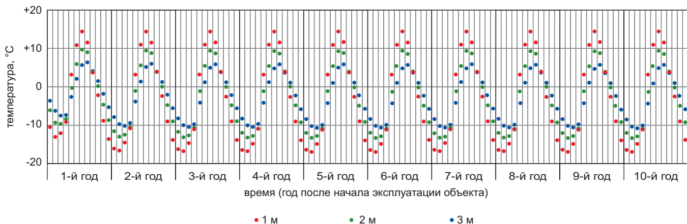
Рис. 10. График сезонного хода температуры на разных глубинах (при наличии снежного покрова в зимний период)
