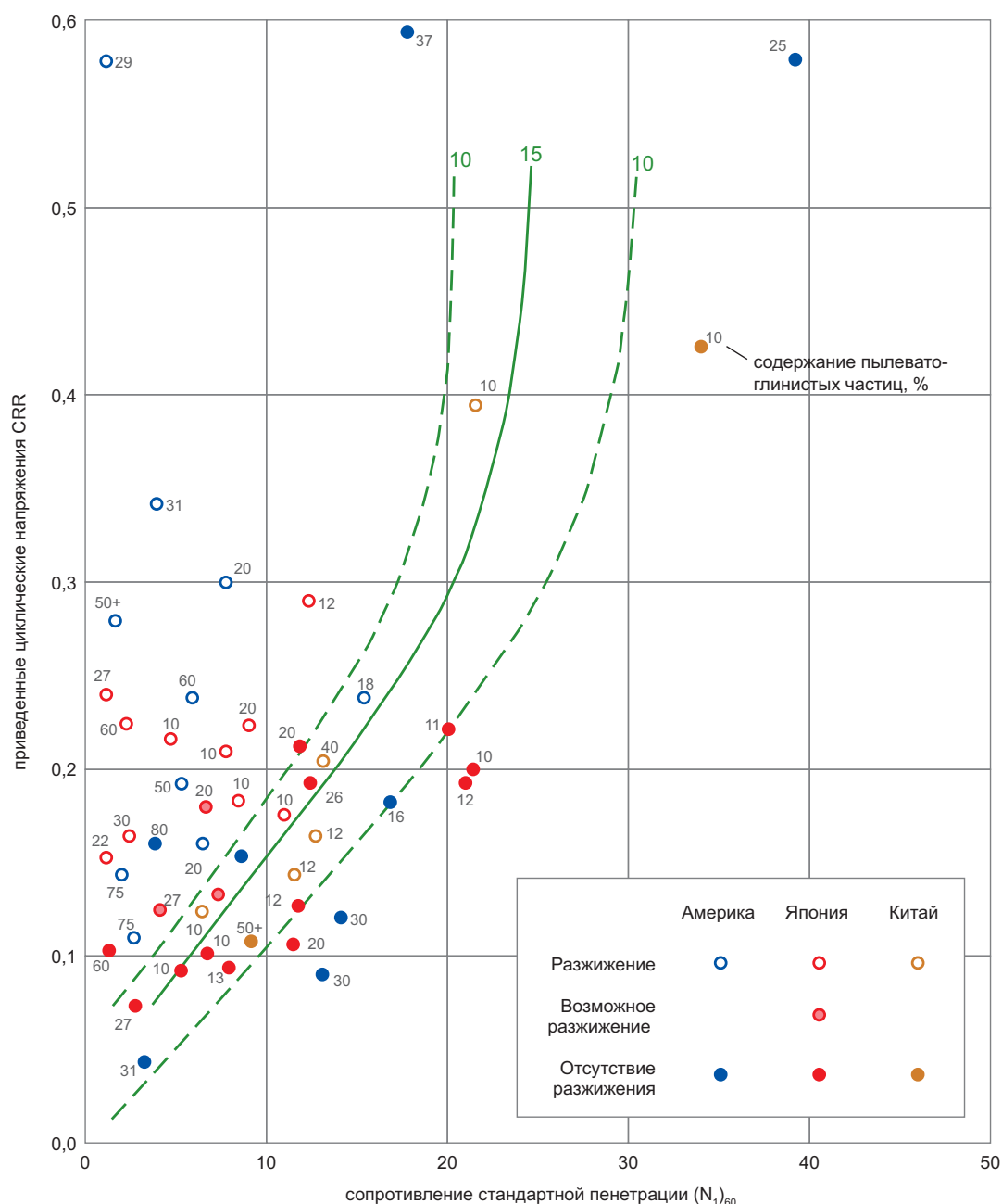
Рис. 1. Зависимость между приведенными циклическими напряжениями, вызывающими разжижение, и сопротивлением стандартной пенетрации для чистых и пылеватых песков при землетрясениях с магнитудой 7,5 [24]. Цифрами над верхними концами кривых указаны соответствующие им величины содержания пылевато-глинистых частиц FC, %
