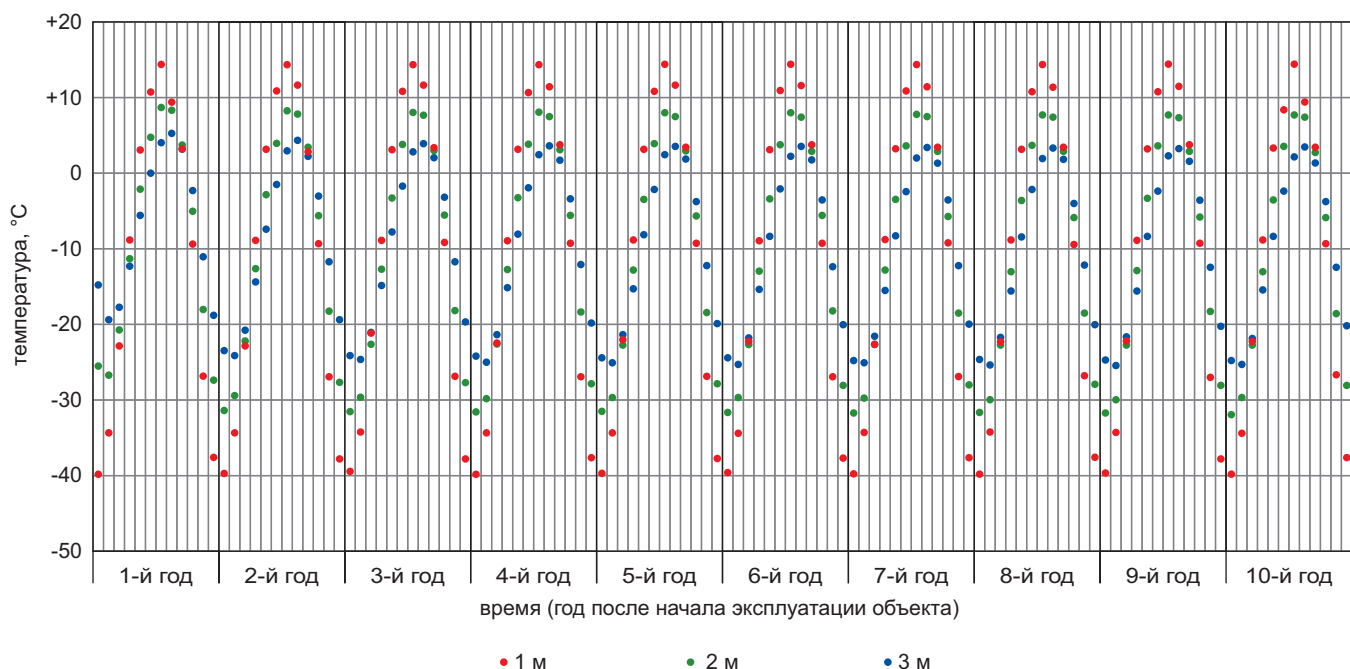
Рис. 11. График сезонного хода температуры на разных глубинах (при расчистке снега в зимний период)
