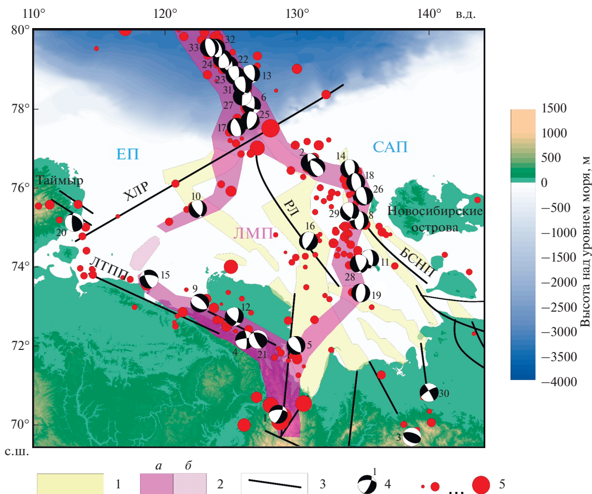
Рис. 2. Схема сейсмотектоники Лаптевоморского региона, по [Аветисов, 2000; Сейсмотектоника ..., 2017] с изменениями и дополнениями.
