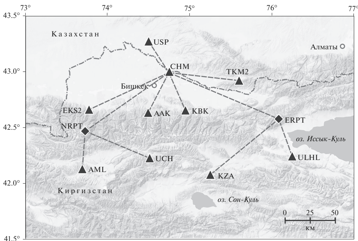
Рис. 1. Положение станций киргизской сейсмологической сети KNET. Треугольники — сеймостанции; пунктирные прямые линии — телеметрическая радиосвязь между станциями и ретрансляторами (четырёхугольники) для управления и передачи данных.
