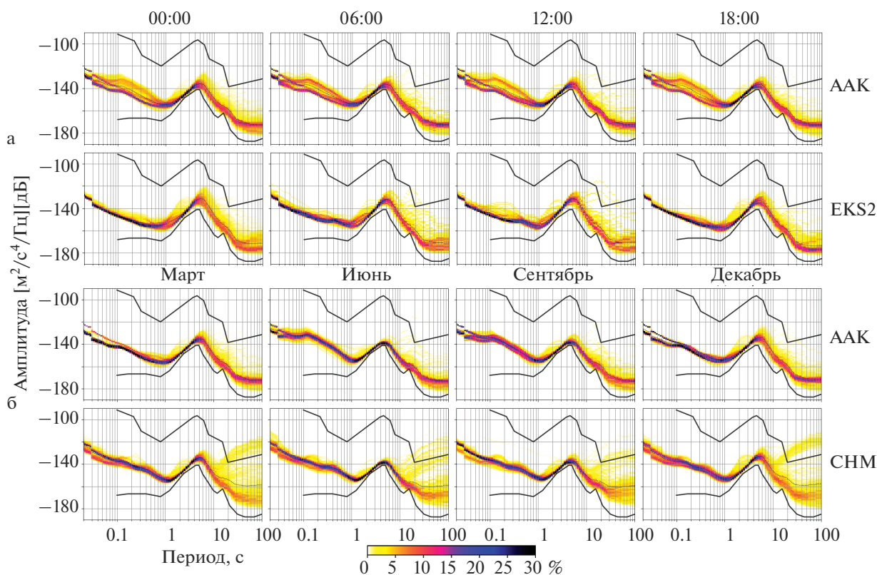
Рис. 6. ВСПМ сейсмического шума (канал Z): а — по временам суток (станции AAK и EKS2); б — по временам года (AAK и CHM).
