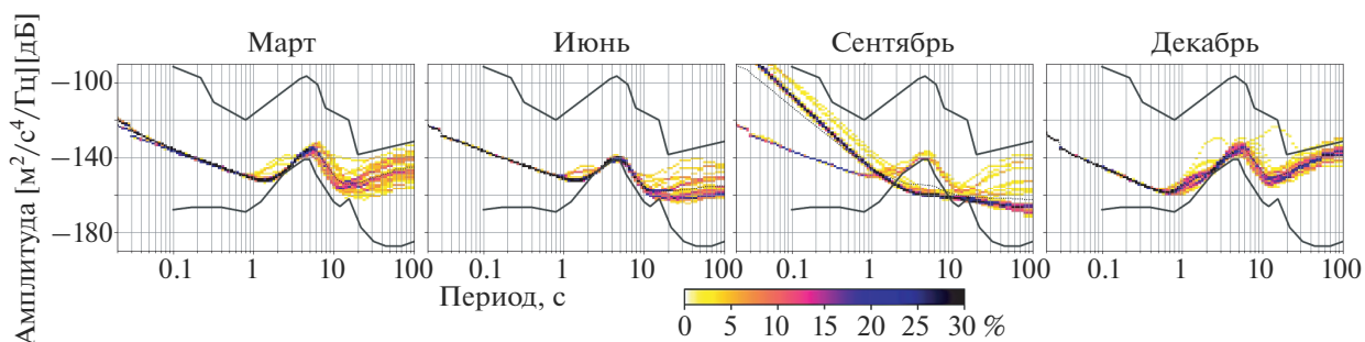
Рис. 11. ВСПМ станции UCH по каналу E для 2009 г.
