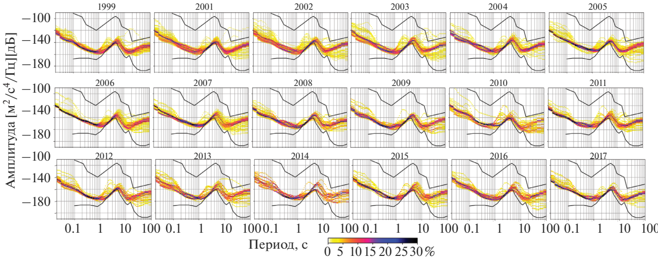
Рис. 9. ВСПМ для станции TKM2 по годам исследования для N канала.
