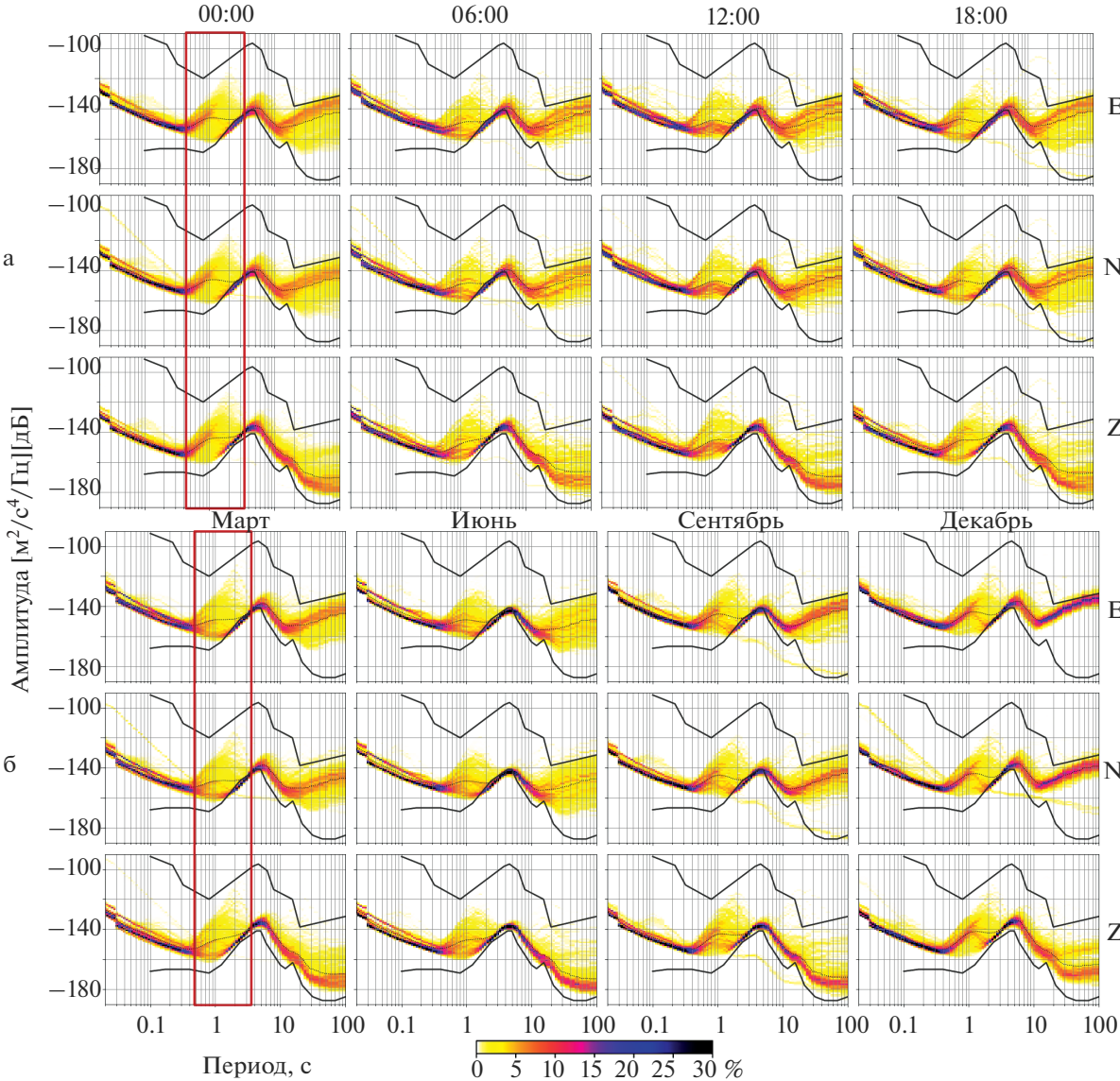
Рис. 8. ВСПМ для станции ULHL по временам суток (а) и временам года (б) по всем каналам.
