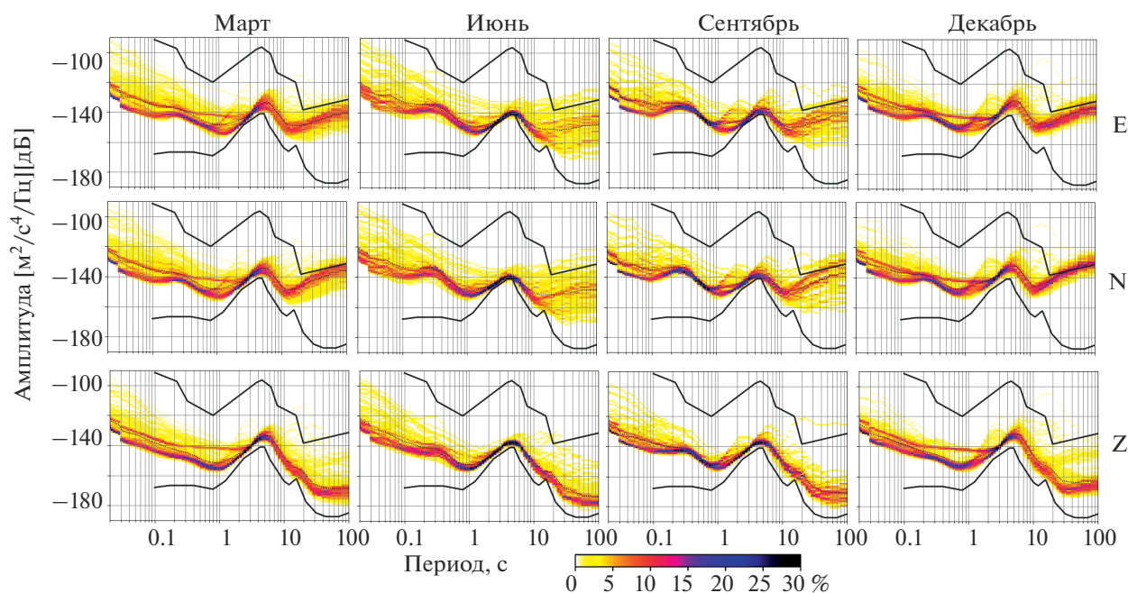
Рис. 7. ВСПМ станции KBK по всем каналам за март, июнь, сентябрь, декабрь.
