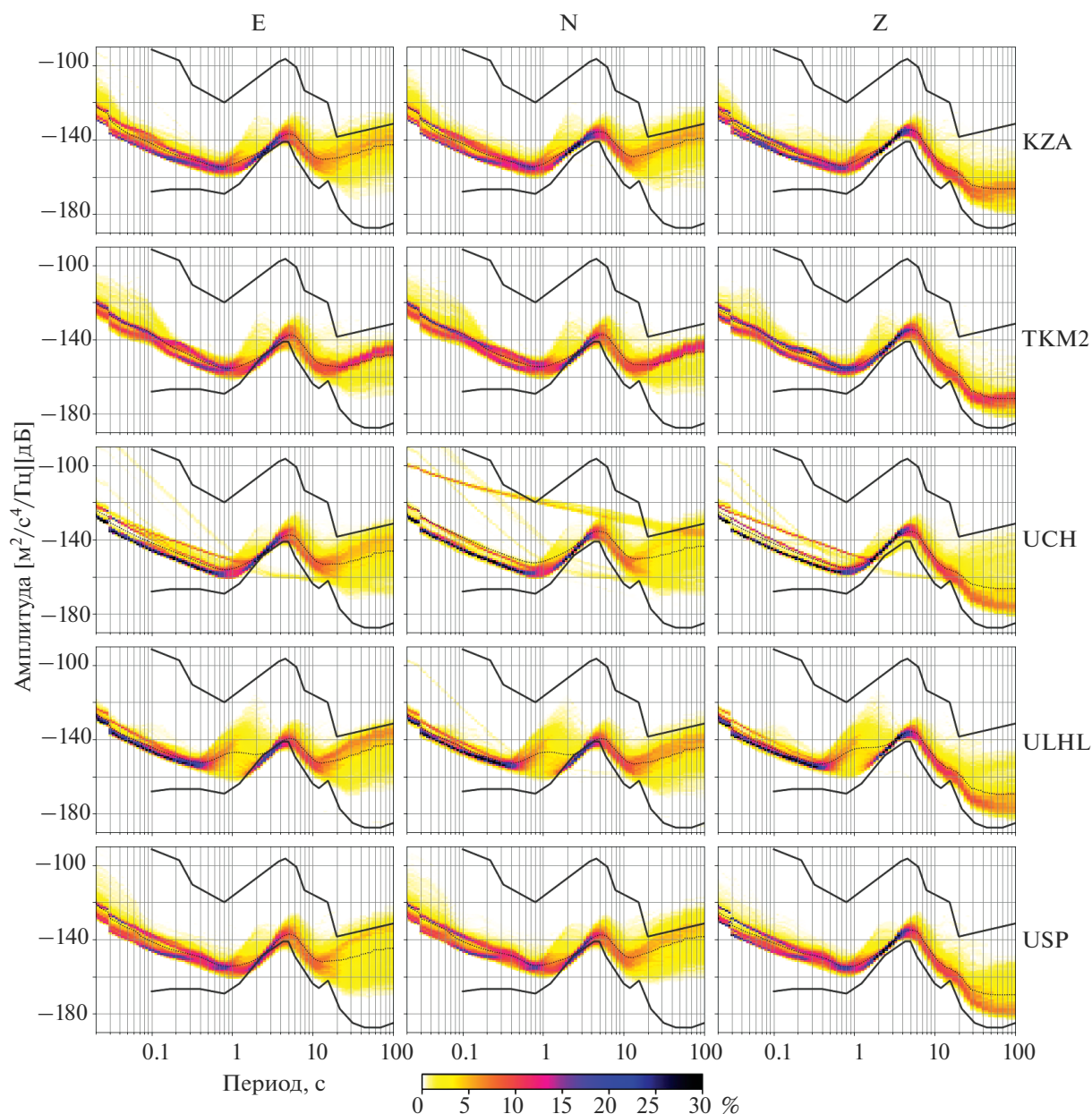
Рис. 5. ВСПМ сейсмического шума по всем каналам станций KZA, TKM2, UCH, ULHL и USP, построенные по всему набору данных.
