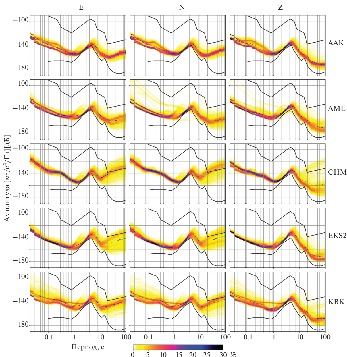
Рис. 4. ВСПМ сейсмического шума по всем каналам станций AAK, AML, CHM, EKS2 и KBK, построенные по всему набору данных. Тонкой черной пунктирной линией на этом и всех последующих рисунках ВСПМ показана кривая зависимости среднего значения ВСПМ от частоты.
