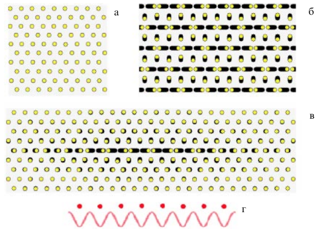
Рис. 8. (а) Двумерный кристалл Морса, атомы которого расположены в узлах треугольной решётки. (б) Стробоскопическая картина движения атомов для коротковолновой фононной моды в нелинейном режиме. (в) Стробоскопическая картина движения атомов в окрестности ДБ, полученная наложением колоколообразных функций на коротковолновую фононную моду, изображённую на рис. б. Перемещения атомов на рис. б и в увеличены для наглядности в семь раз. (г) Схема одномерной модели для качественного изучения ДБ, изображённого на рис. в. Цепочка атомов испытывает действие периодического локального потенциала, созданного атомами, окружающими плотноупакованный атомный ряд, в котором возбуждён ДБ.
