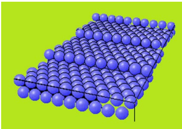
Рис. 12. Вициальная поверхность кристалла. Край террасы представляет собой одномерную периодическую структуру, на которой могут существовать ДБ. Атомно-гладкая поверхность — это двумерная периодическая структура, которая также может поддерживать ДБ.
