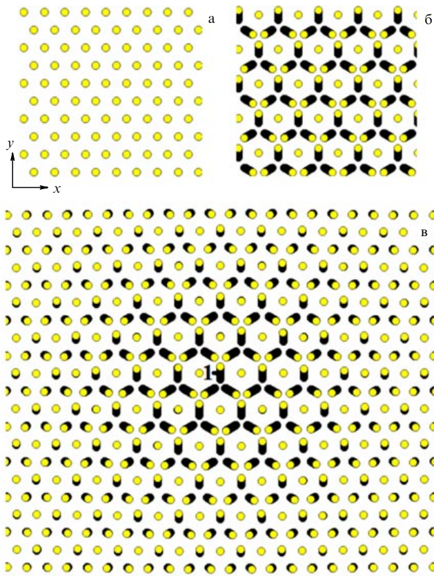
Рис. 9. (а) Двумерный кристалл Морса, атомы которого расположены в узлах треугольной решётки. (б) Стробоскопическая картина движения атомов для высокосимметричной фононной моды с волновым вектором на границе зоны Бриллюэна в нелинейном режиме. (в) Стробоскопическая картина движения атомов в окрестности ДБ, полученного наложением колоколообразной функции с радиальной симметрией на коротковолновую фононную моду в нелинейном режиме. На рисунках б, в перемещения атомов для наглядности увеличены в семь раз.
