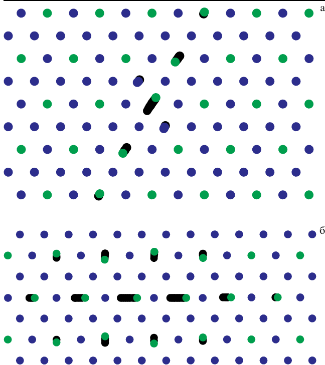
Рис. 3. Стробоскопическая картина движения атомов вблизи ДБ в кристалле Pt_3Al (по результатам работы [80]). Тяжёлые атомы Pt изображены более тёмным цветом, чем лёгкие атомы Al. (а) Щелевой ДБ, локализованный преимущественно на одном лёгком атоме, совершающем колебания в противофазе с соседними лёгкими атомами в плотноупакованном атомном ряду. (б) ДБ с частотой выше частот фононного спектра, локализованный преимущественно на четырёх-пяти атомах Al, расположенных в одном плотноупакованном ряду. Данные атомы совершают синфазные колебания. Этот ДБ, в отличие от щелевого, может двигаться вдоль плотноупакованного ряда.
