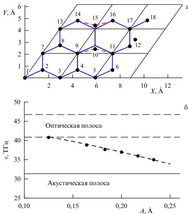
Рис. 15. (а) Расчётная ячейка с периодическими граничными условиями для моделирования из первых принципов ДБ в графене, подвергнутом одноосному растяжению вдоль оси X [220]. ДБ возбуждался посредством начального отклонения атомов 10 и 15 вдоль оси Y в противоположных направлениях. (б) Зависимость частоты \nu ДБ в графене от его амплитуды A .
