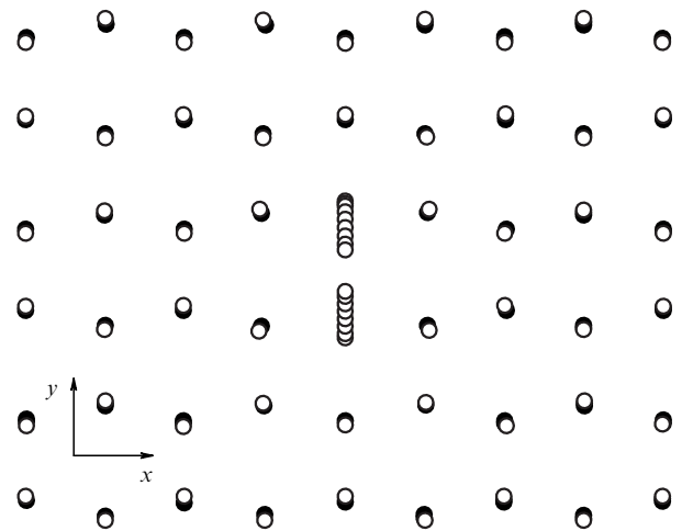
Рис. 4. Стробоскопическая картина движения атомов вблизи ДБ в однородно деформированном графене (по результатам работы [68]). Изучены также кластеры таких ДБ [69]. Частота ДБ лежит в щели фононного спектра графена, появившейся в результате приложения однородной деформации.
