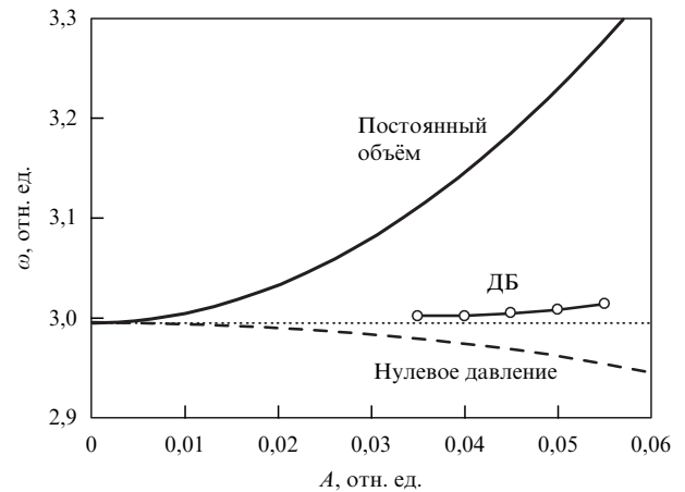
Рис. 10. Зависимость частоты фононной моды, представленной на рис. 9б, от амплитуды в нелинейном режиме: сплошная кривая — при неизменных размерах расчётной ячейки, штриховая кривая — при нулевом давлении. Горизонтальная пунктирная линия показывает верхнюю границу фононного спектра, \omega_{\max} = 2,995 . Кружки, соединённые линией, представляют зависимость частоты ДБ, показанного на рис. 9в, от амплитуды колебания его центральных атомов.
