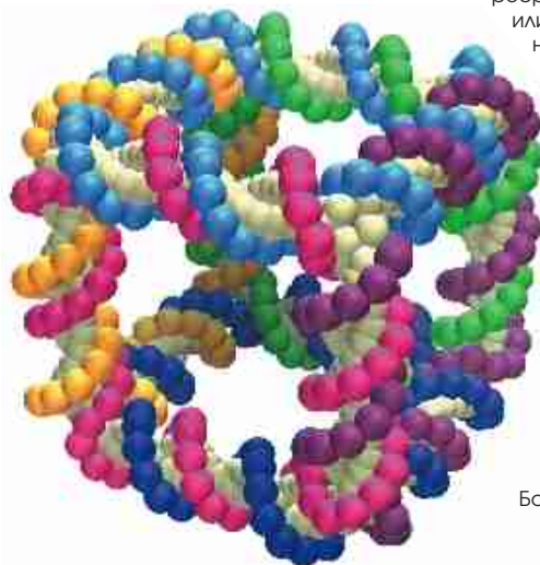
Куб из стержней (внизу слева), составленный из шести петель ДНК, показывает, что из ДНК можно строить трехмерные структуры. Основа каждой цепи ДНК изображена цветными сферами (для каждой цепи взята другой цвет), а основания обозначены как белые сферы. Каждое ребро куба содержит 20 пар нуклеотидов, или примерно два полных оборота двойной спирали. Каждый угол – узел с тремя ветвями. Упрощенная схема (внизу справа) показывает, как связаны цепи ДНК, но опускает их спиральное закручивание.
