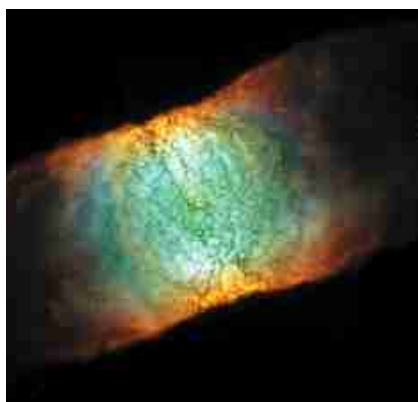
Планетарная туманность Сетчатка Глаза (IC 4406),
