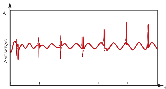
Рис. 10. Первичный Фурье-анализ отраженного ультразвукового сигнала.
