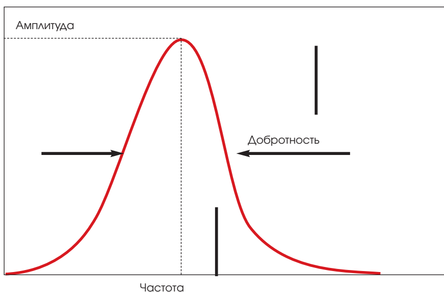
Рис. 9. Локальный анализ резонансных кривых.
