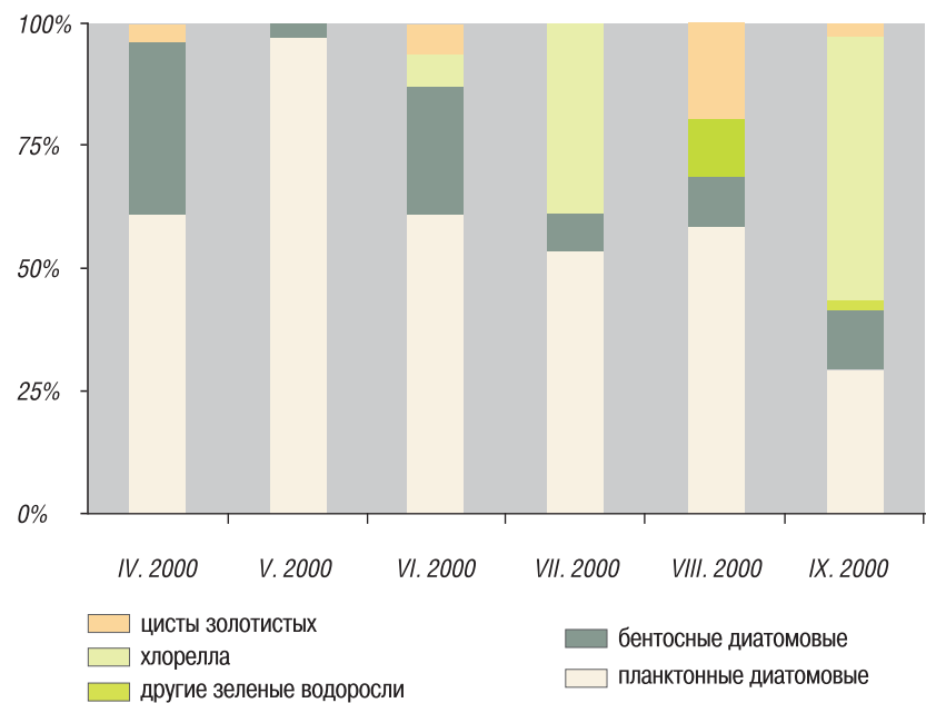
Пример сезонной динамики компонентов пищевого комка у байкалийд. Вид Liobaicalia stiedae , населяющая песчаную литораль у пос. Култук (по Roepstorf, Sitnikova, 2003)
