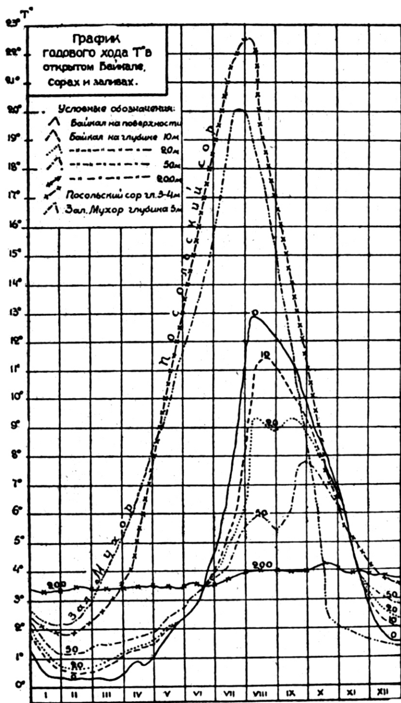
Рис. 3. График годового хода темпе- ратуры воды в открытом Бай- кале, сорах и заливах (по Кожову)
