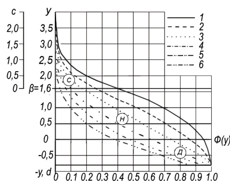
Рис. 1 – Обобщенная водохозяйственная характеристика (ОВХ) 1-6 – варианты \lambda ; C – холостые сбросы; H – наполнения; D – дефициты
