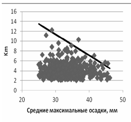
Рис. 1 – Зависимость коэффициента Km от среднееголетнего максимума суточных осадков для ЕТР и её верхняя огибающая
