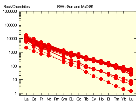
Fig. 8. REE pattern Khibina apatite.
