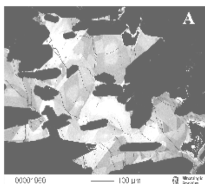
Fig. 5. Interstitial eudialyte.
