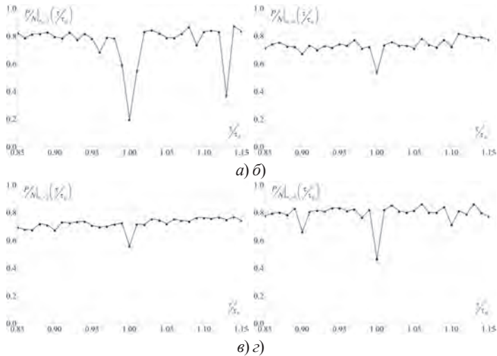
Рис. 1 – Графики значений отношений ложных ближайших соседей к длине ряда P/N для пространства вложения m_c = 2 (при переходе в m_c = 3 ) в виде зависимостей от \tau / \tau_0 для следующих систем: а) ИСН - 1 б) ИСН - 2 в) ИСН - 3 г) 2 - ИСН - 1
