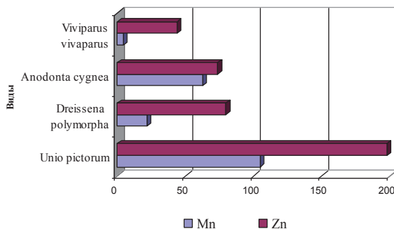
Рис. 2. Содержание марганца и цинка в мягких тканях моллюсков (мг / кг сух. массы)
