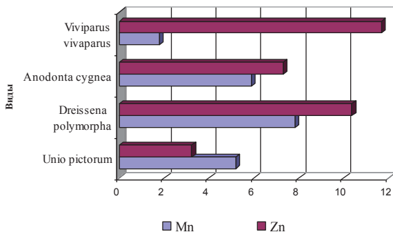
Рис. 1. Содержание марганца и цинка в раковинах моллюсков (мг / кг сух. массы)
