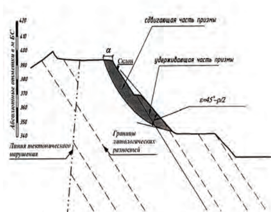
Рисунок 1 – Механизм формирования призмы обрушения по склону
