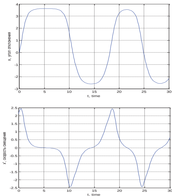
Рисунок 4 – Колебательный процесс при \dot{x}(0) = 2,1176
