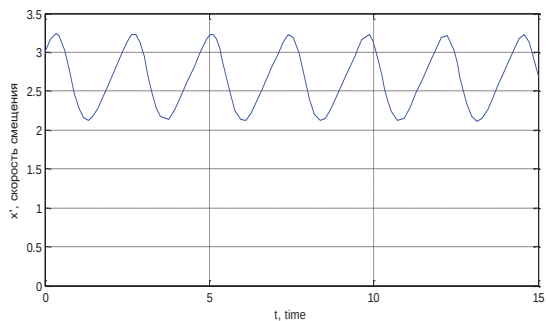
Рисунок 2 – Колебательный процесс при \dot{x}(0) = 3
