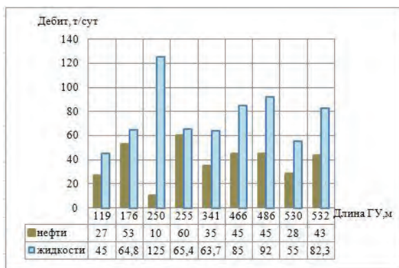
Рисунок 2 Продуктивность горизонтальных скважин
