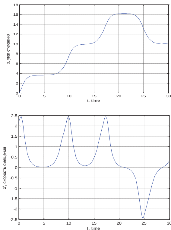
Рисунок 5 – Колебательный процесс при \dot{x}(0) = 2,1177
