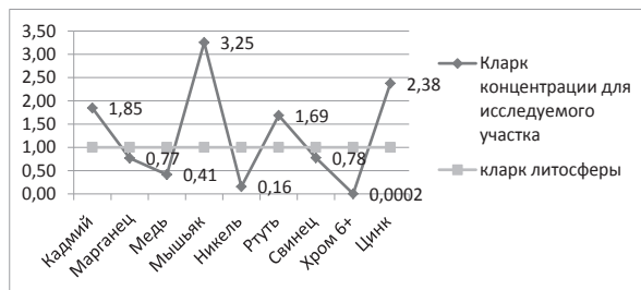
Рисунок 1. Геохимический спектр донных отложений пруда Коммунар реки Миасс Челябинской области, рассчитанный по литосферным кларкам
