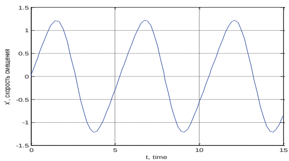
Рисунок 1 – Колебательный процесс при \dot{x}(0) = 0
