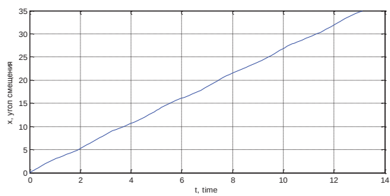
Рисунок 1 – Колебательный процесс при \dot{x}(0) = 0
