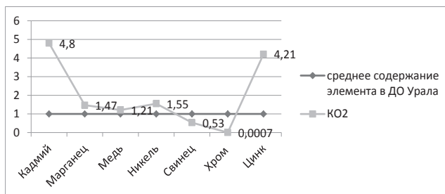
Рисунок 2. Геохимический спектр донных отложений пруда Коммунар реки Миасс Челябинской области, рассчитанный по среднему содержанию элементов в ДО Урала
