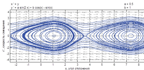
Рисунок 3 – Фазовый портрет модели
