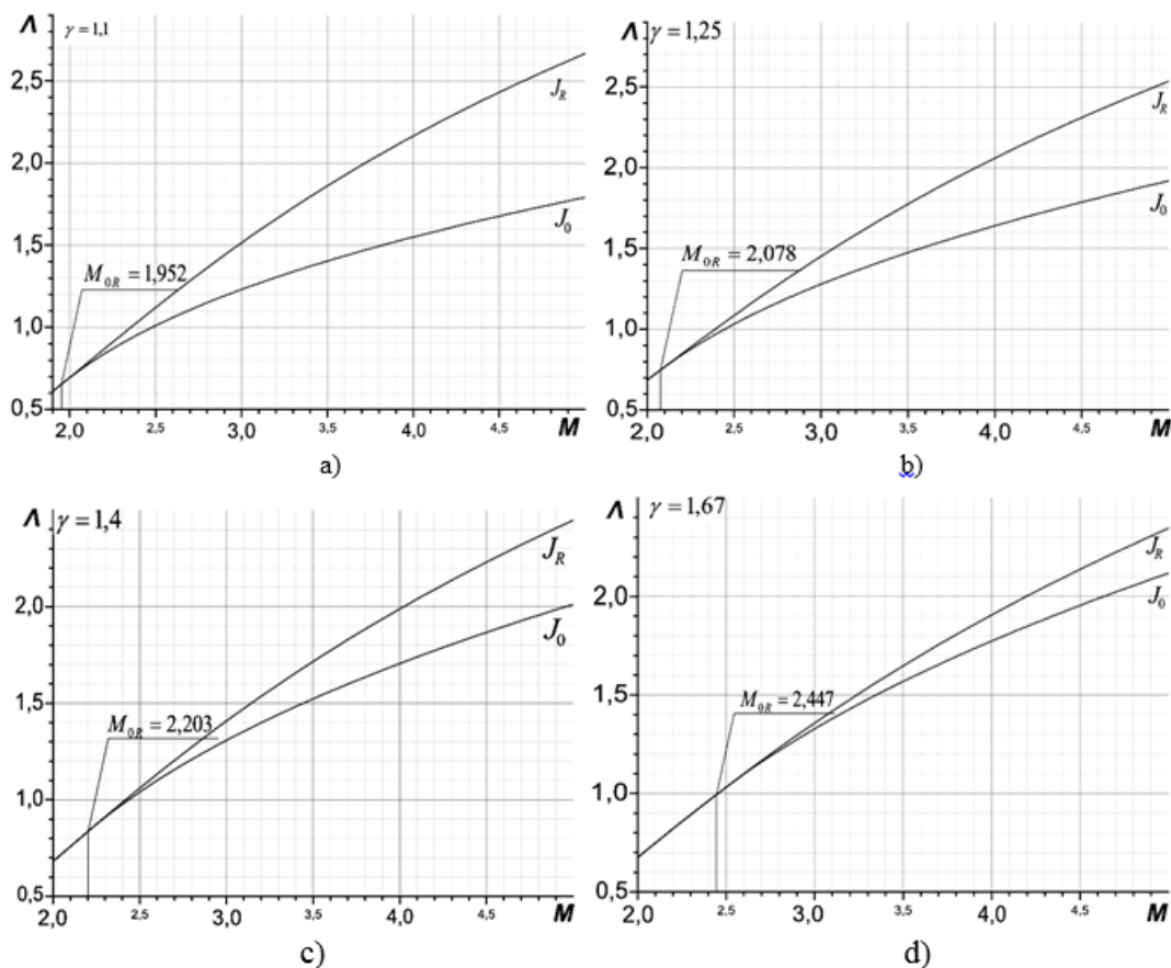
Рис. 5. Область неоднозначности, в которой возможно как РО так и МО скачка от стенки
