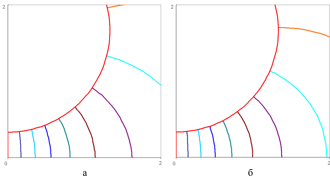
Рис. 6. Линии тока в МЭП: а – для зависимости (7); б – для эквипотенциального анода
