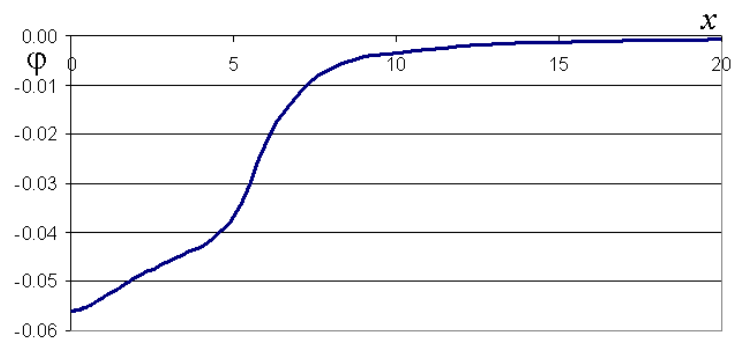
Рис. 3. Распределение потенциала по поверхности анода
