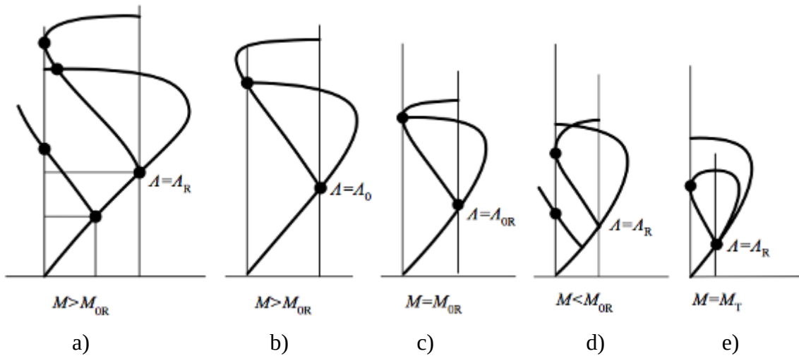
Рис. 2. Переход от регулярного отражения к маховскому
