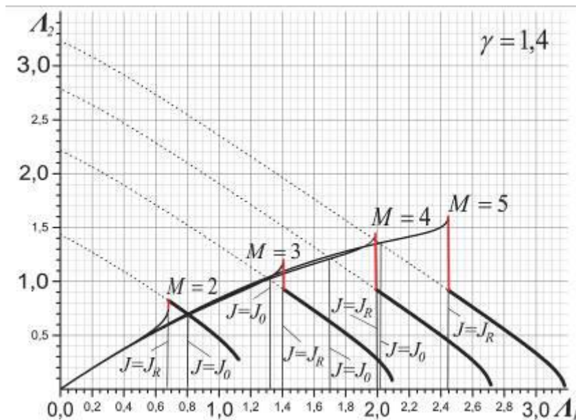
Рис. 4. Зависимость интенсивности отраженного скачка от интенсивности приходящего скачка
