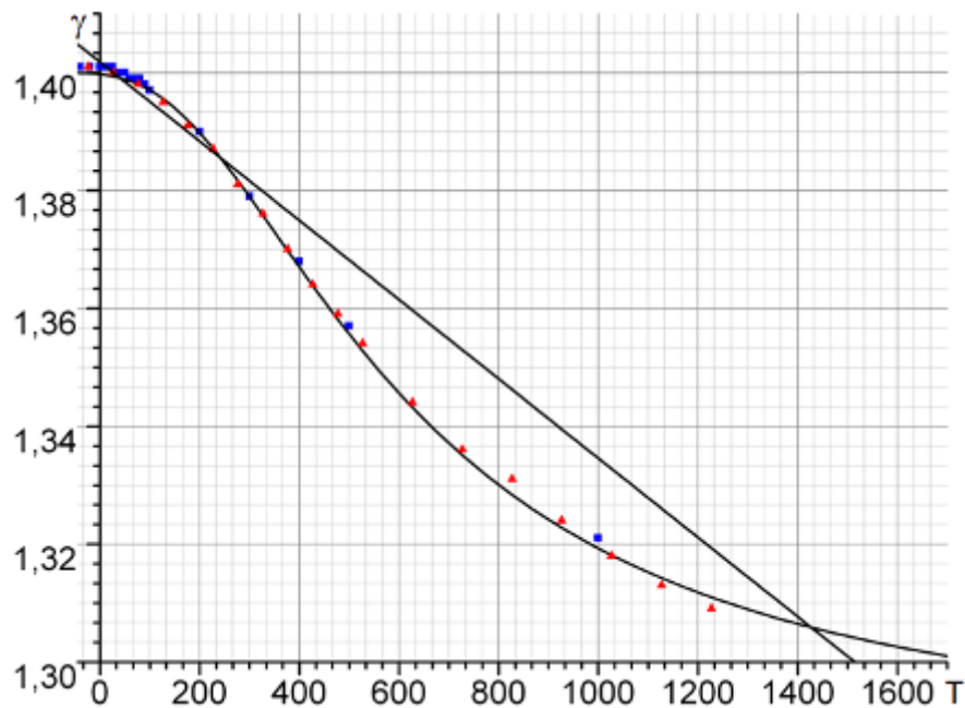
Рис. 6. Сравнение зависимости показателя адиабаты от температуры (°C) с линейным приближением и экспериментальными данными (красные треугольники – [20], синие квадраты – [21])
