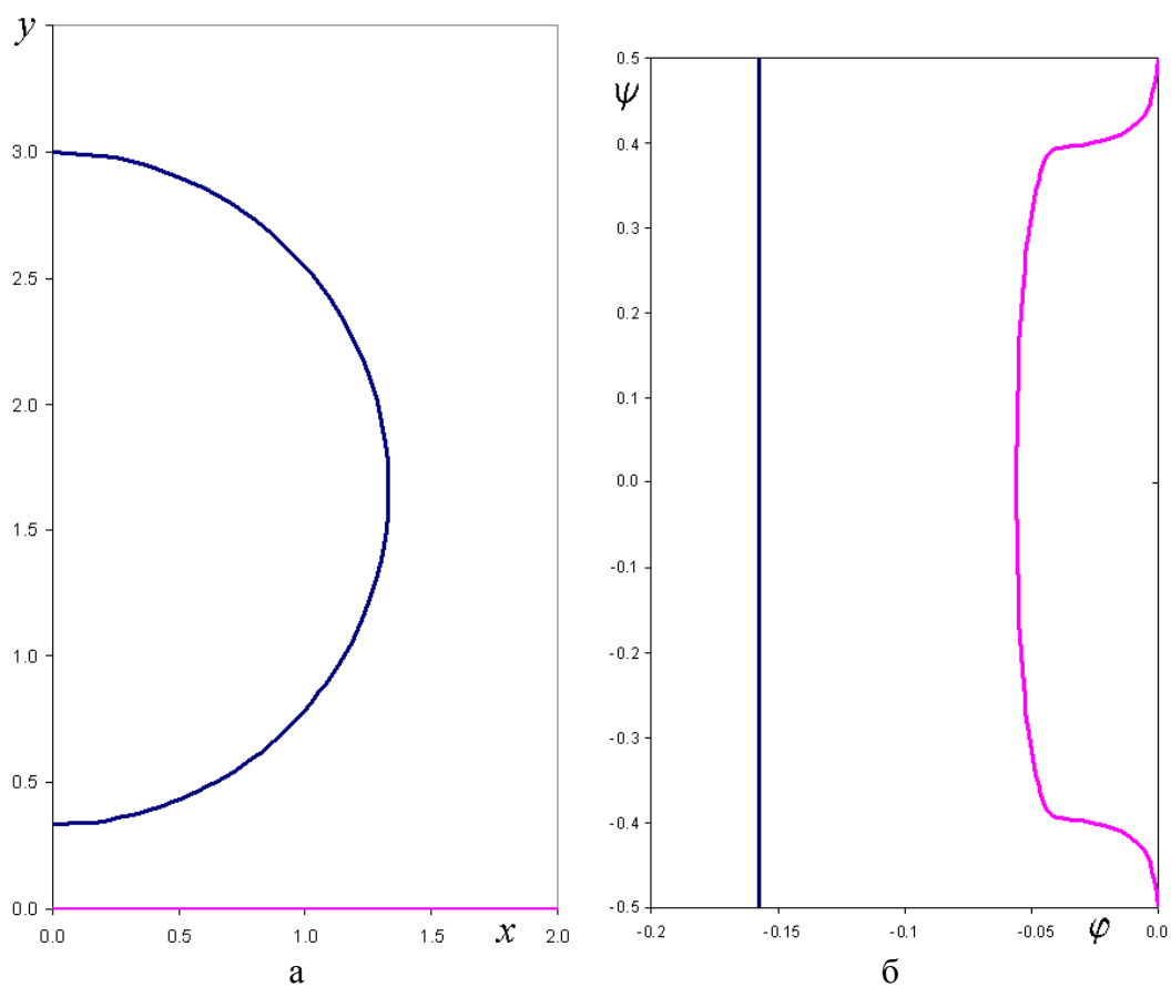
Рис. 2'. Формы области на плоскостях: а – физической z ; б – комплексного потенциала w
