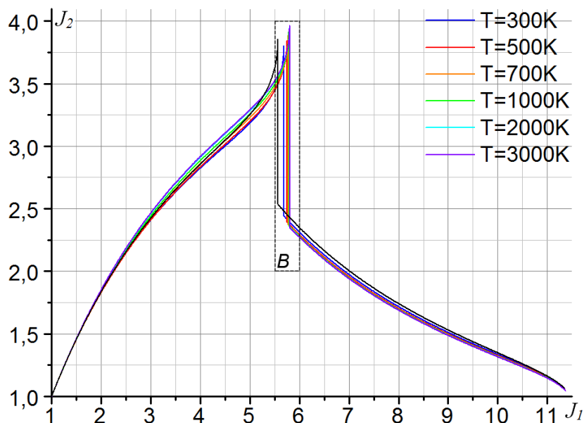
Рис. 7. Зависимость интенсивности отраженного скачка от интенсивности приходящего скачка при числе Маха M=3.5 и \gamma_i=1,4 для различной температуры окружающей среды
