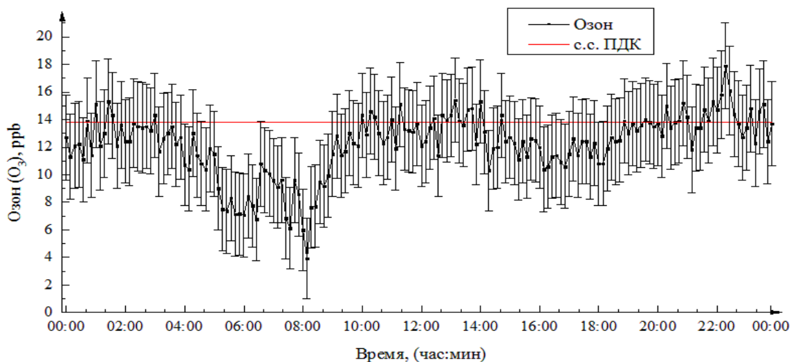
Рис. 1. Суточный ход значений концентраций озона ( O_3 )
