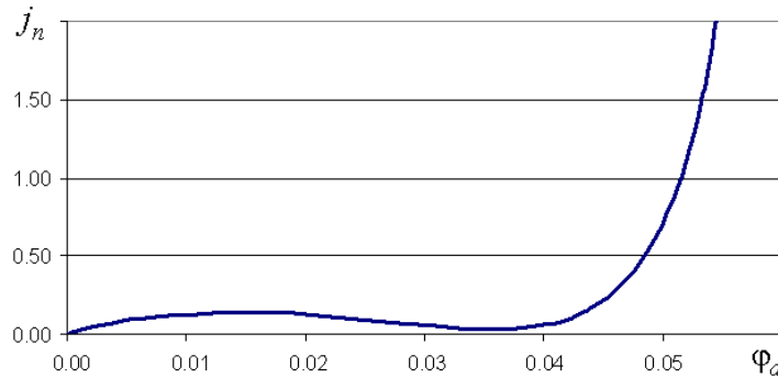
Рис. 2. График аппроксимирующей зависимости (7) для k=50
