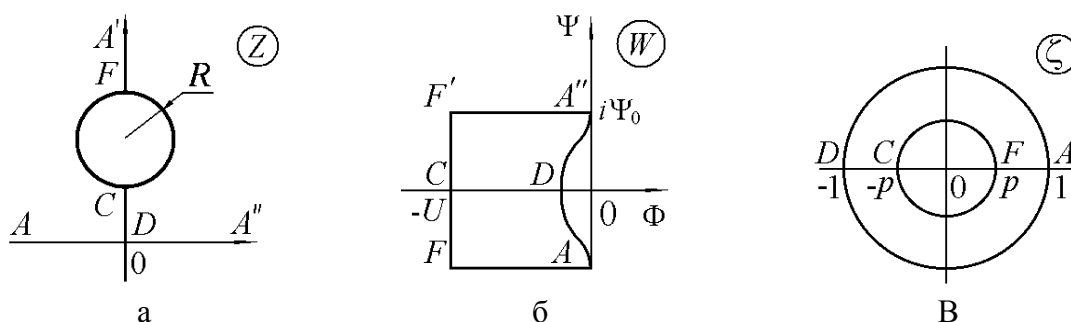
Рис. 1. Формы области на плоскостях: а – физической; б – комплексного потенциала; в – параметрической плоскости
