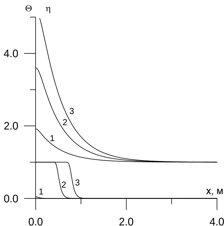
Рис. Распределение температуры и концентрации конечного продукта
