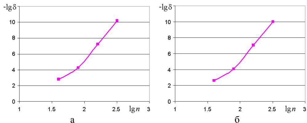
Рис. 7. Оценка погрешности параметров в точке D: а – потенциала; б – плотности тока
