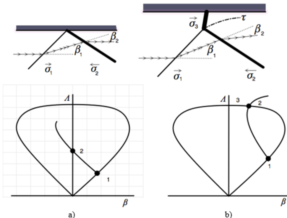
Рис. 1. Регулярное (а) и нерегулярное (б) отражение косоугольного скачка \sigma_1 от стенки
