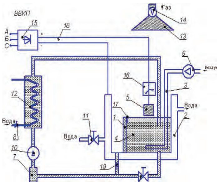
Рисунок. 1. - Функциональная схема экспериментальной установки
