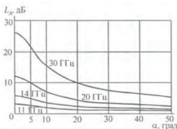
Рисунок 1. Ослабление радиосигнала в дожде при I = 6 \text{ мм / ч}
