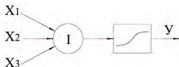
Рис. 2. Структурная модель искусственного нейрона
