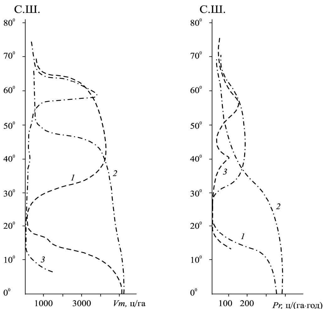
Рис. 6.2. Зональное распределение фитомассы Vm и фитопродукции Pr Секторы: 1-приатлантический, 2-притихоокеанский, 3-континентальный.
