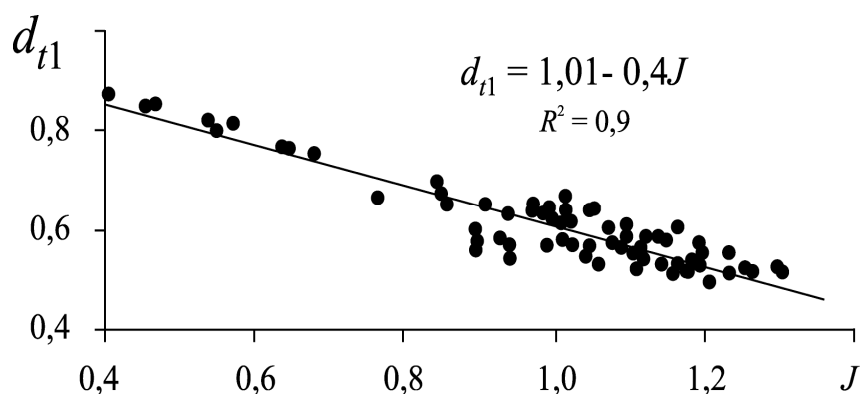
Рис. 5.4. Связь J и d_{t1}
