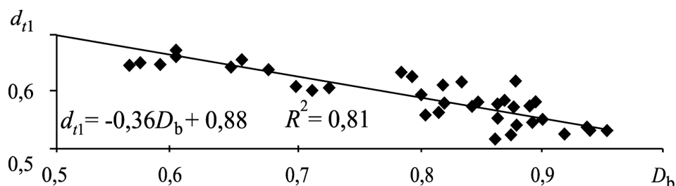
Рис. 7.5. Связь D_b и d_{t1}
