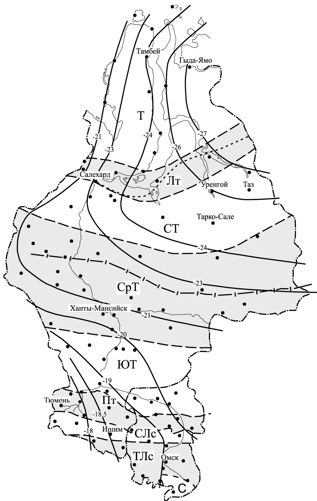
Рис. 5.13. Изолинии t_1 (остальные обозначения по рис. 5.11)
