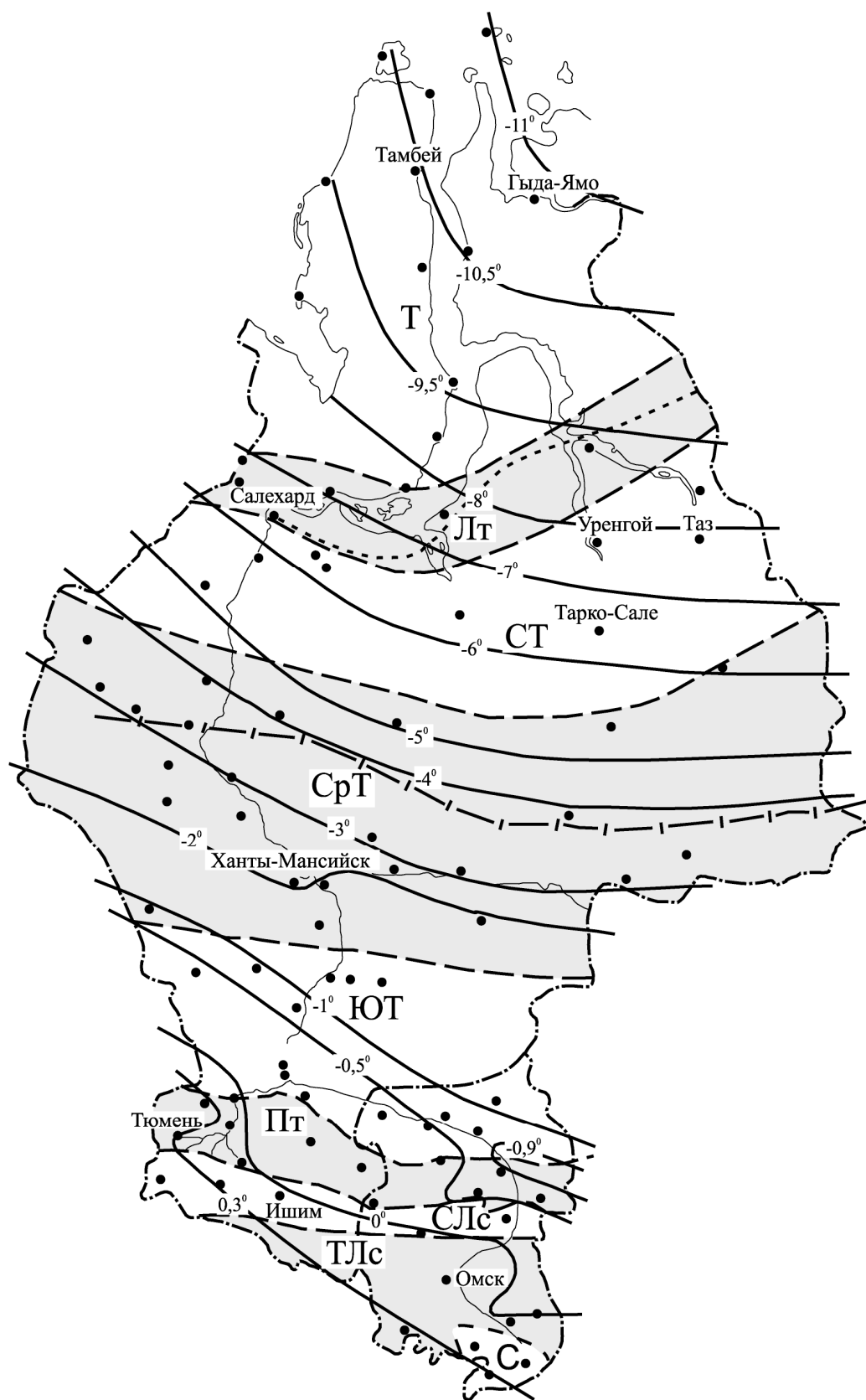
Рис. 5.14 Изолинии t_c (остальные обозначения по рис. 5.11)
