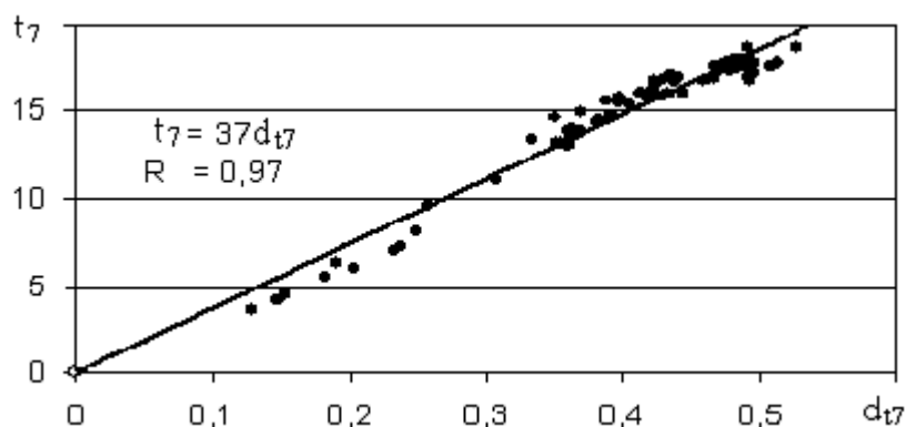
Рис. 5.7. Зависимость t_7 от d_{t7}
