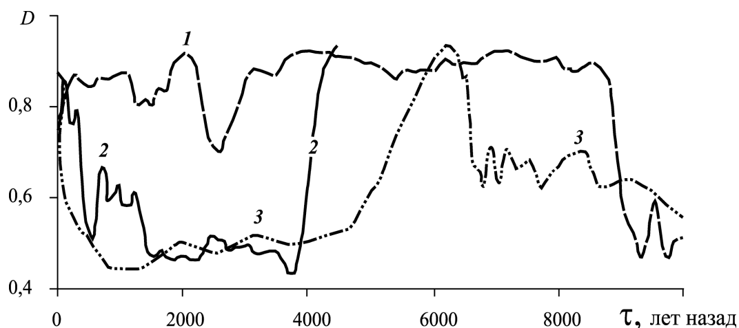
Рис. 4.5. Ход доминанты фоссильных палиноспектров в Западной Сибири и Северном Казахстане (1 - Янтарный, 2- Сладково, 3 - Озерки )
