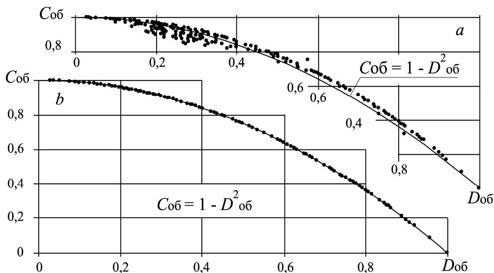
Рис. 4.4. Зависимость C_{об} от D_{об}
