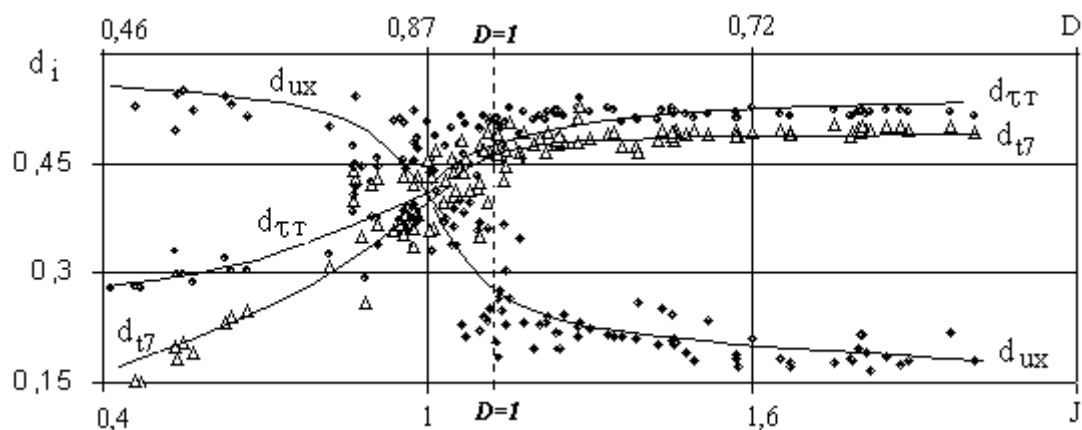
Рис. 5.2. Связь d_{t7} , d_{ux} и d_{\tau\tau} с J и D
