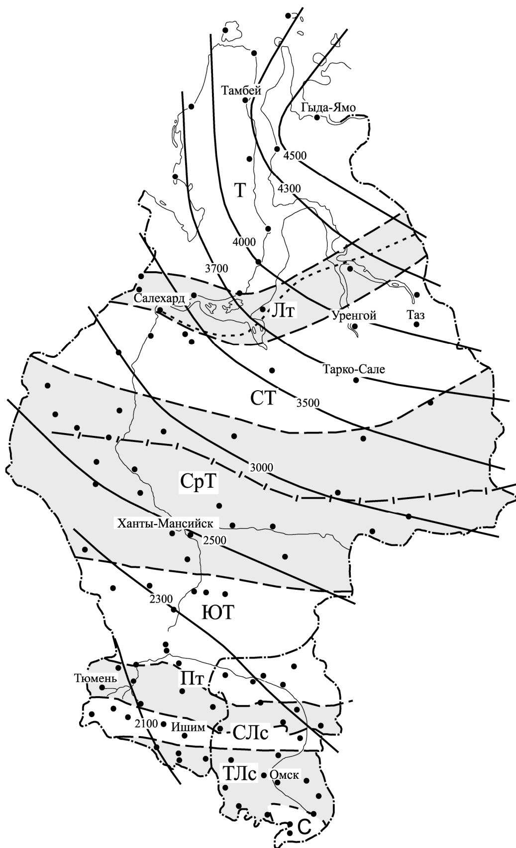
Рис. 5.19. Изолинии \Sigma_0 (остальные обозначения по рис. 5.11)
