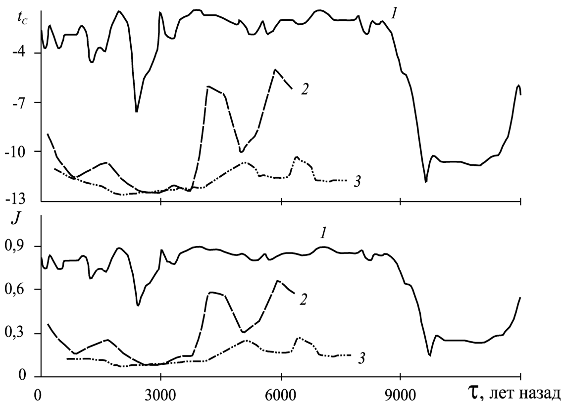
Рис. 8.2. Ход во времени среднегодовой температуры воздуха ( t_c ) и индекса сухости ( J )
