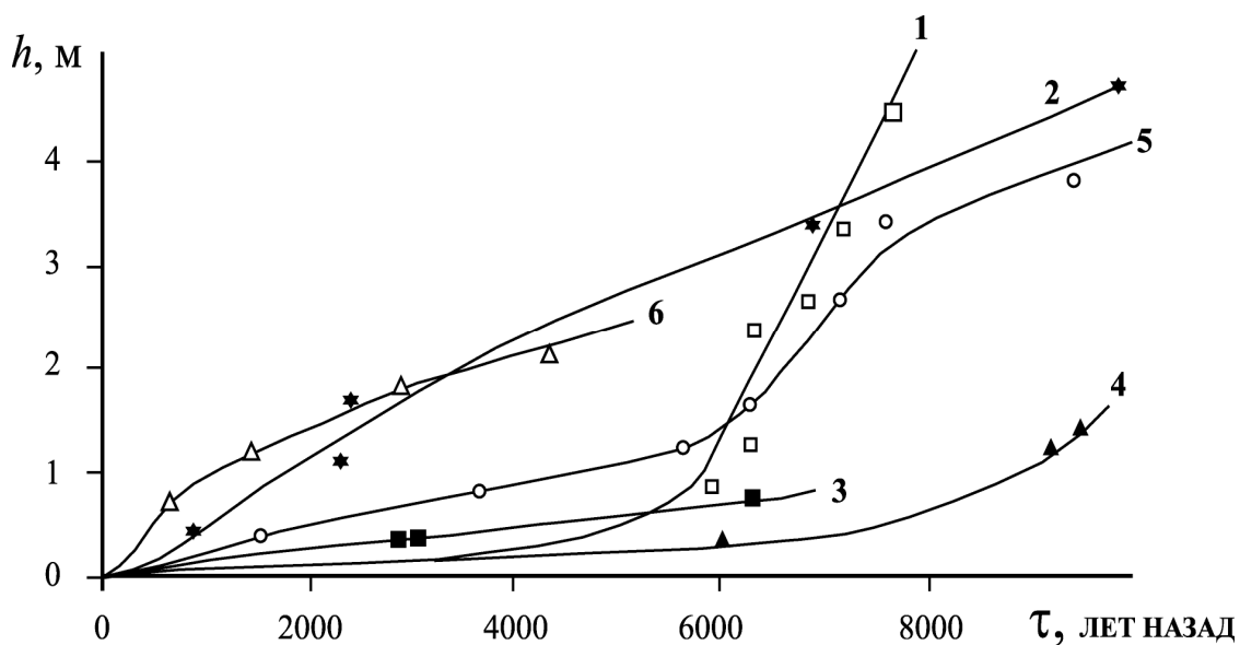
Рис. 2.6. Примеры хода осадконакопления в голоцене в разных районах 1- Ямбура, 2- разрез Янтарный, 3- Салехард, 4- Игарка, 5 Семипалатинск, 6- Сладково
