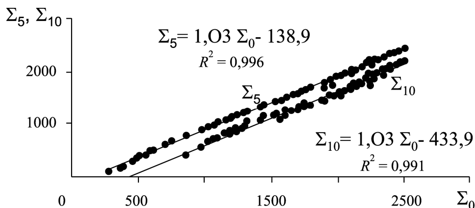
Рис. 5.5. Связь \Sigma_0 , \Sigma_5 и \Sigma_{10}
