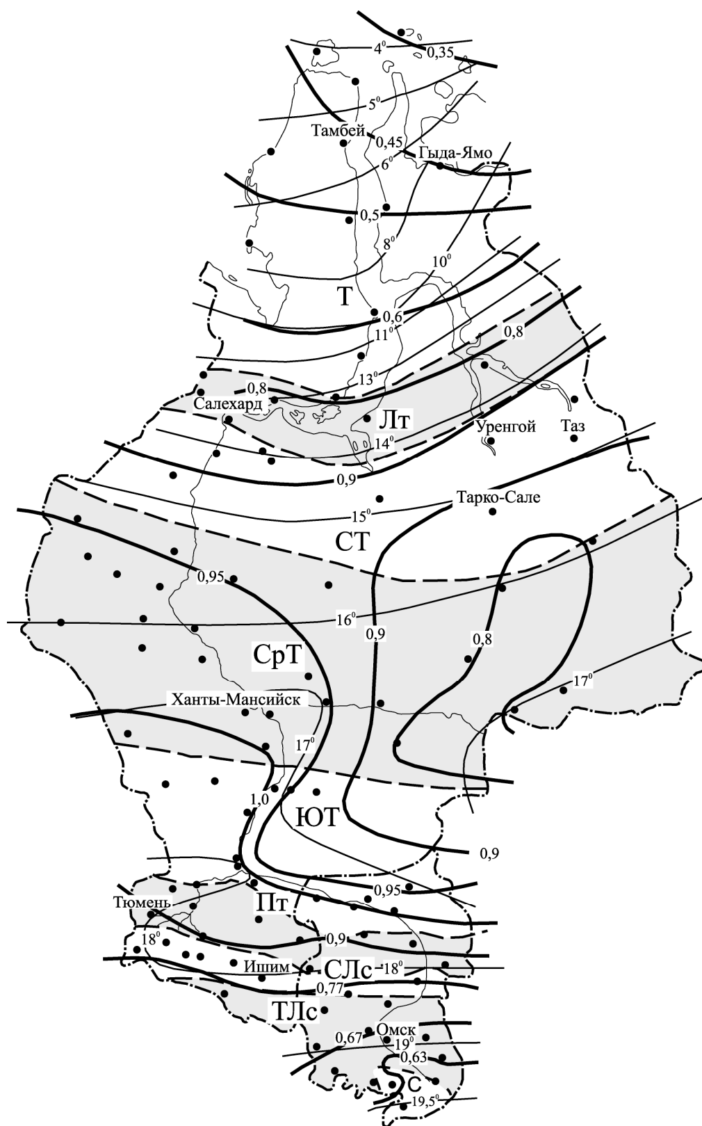
Рис. 7.3. Изолинии D (жирная линия) и t_7 (тонкая линия) (другие обозначения по рис.5.11)
