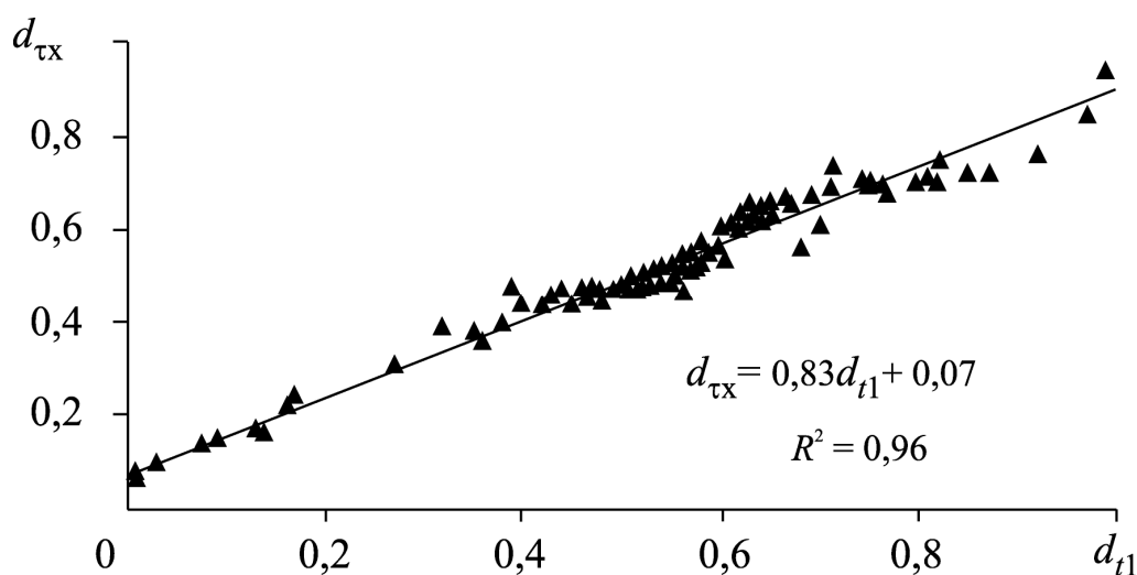
Рис. 5.6. Связь d_{tx} и d_{t1}
