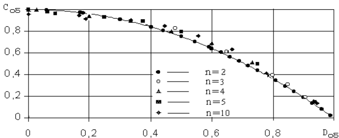
Рис. 3.2. Зависимость C_{об} от D_{об} и n
