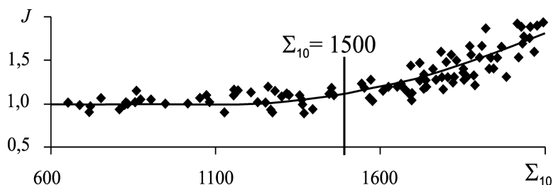
Рис. 5.9. Связь J и \Sigma_{10}
