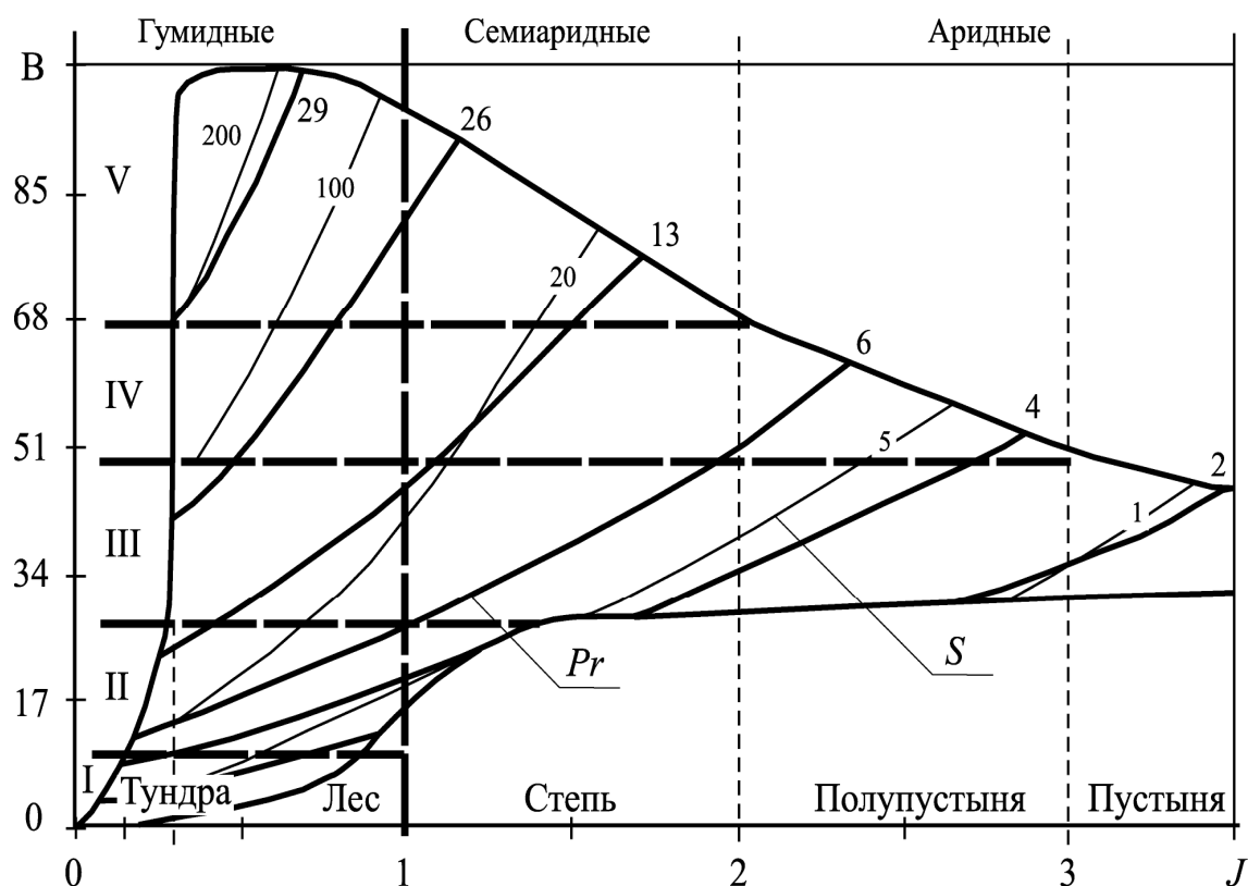
Рис. 2.5. Фитопродукция Pr и сток S в координатах B, J I...V – термические пояса (по рис.2.4)
