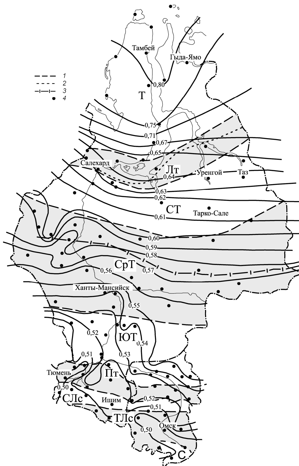
Рис. 5.11. Изолинии d_{11}
