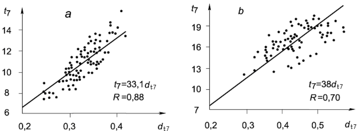
Рис. 5.8. Зависимость t_7 от d_{t7} в Салехарде - a и в Сургуте - b
