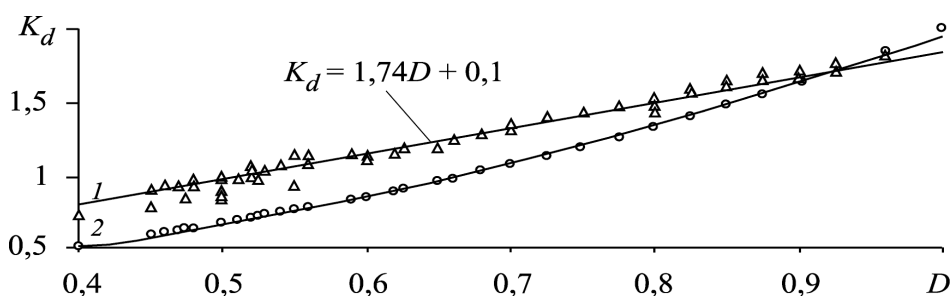
Рис. 7.4. Зависимость коэффициента K_d от D
