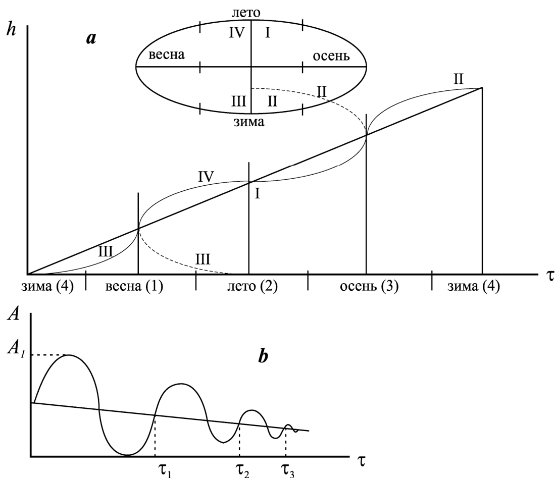
Рис. 2.1. Схематический вид траекторий развития
