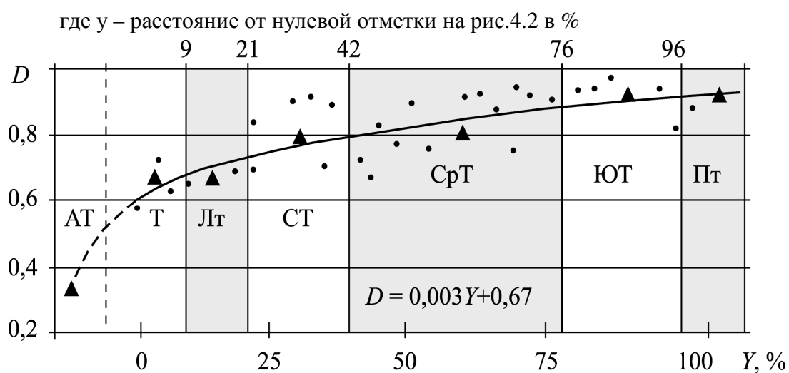
Рис. 4.3. Распределение D по маршруту Новый Порт-Тюмень
