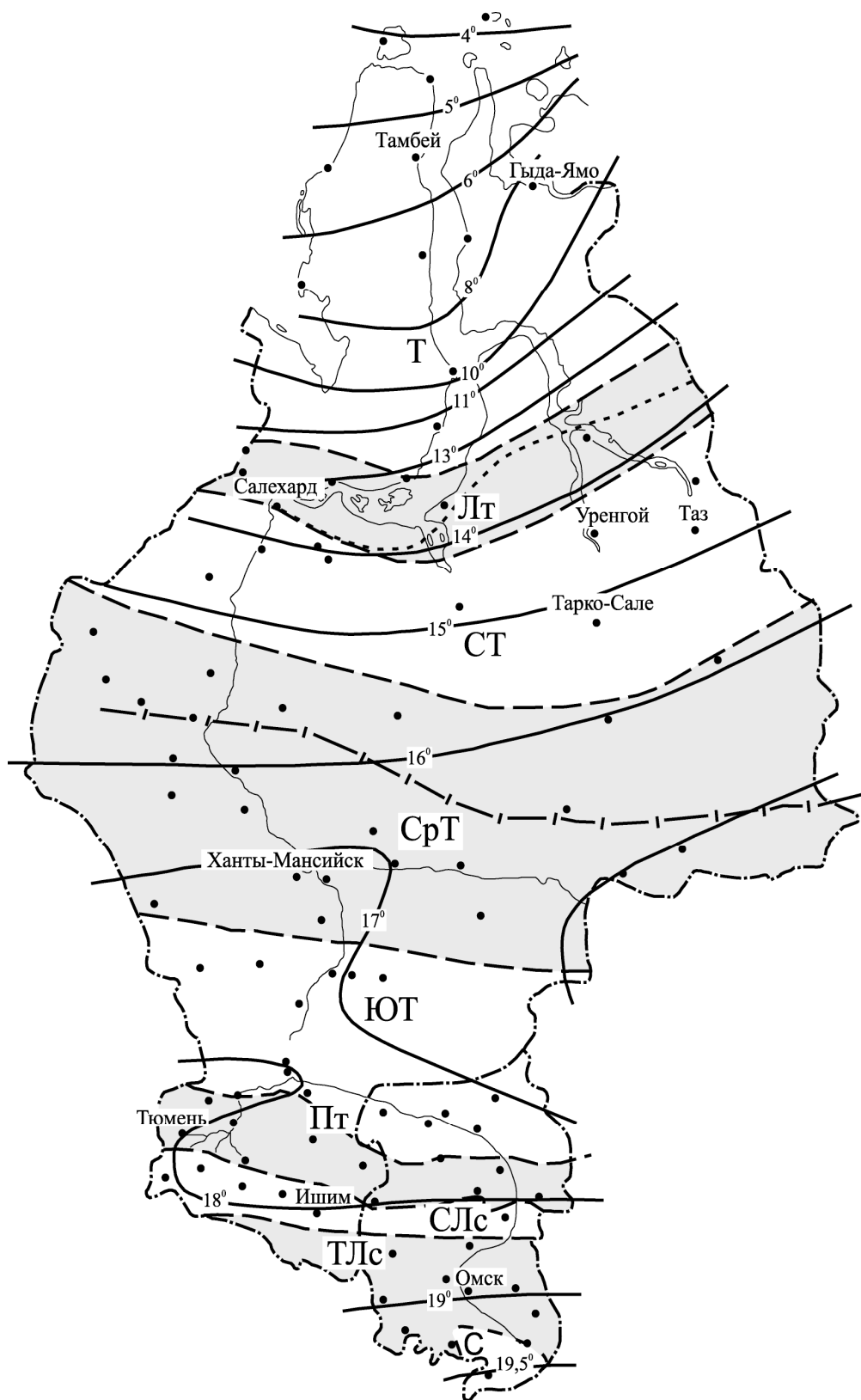
Рис. 5.12. Изолинии t_7 (остальные обозначения по рис. 5.11)
