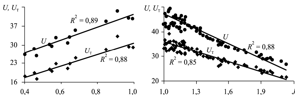
Рис. 5.10. Зависимость сумм осадков U и U_T от индекса сухости J
