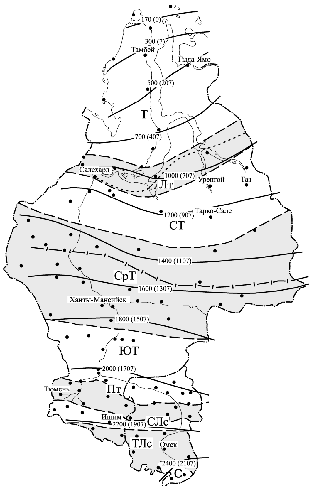
Рис . 5.18. Изолинии \Sigma_5 и \Sigma_{10} ( \Sigma_{10} – в скобках, остальные обозначения по рис. 5.11)
