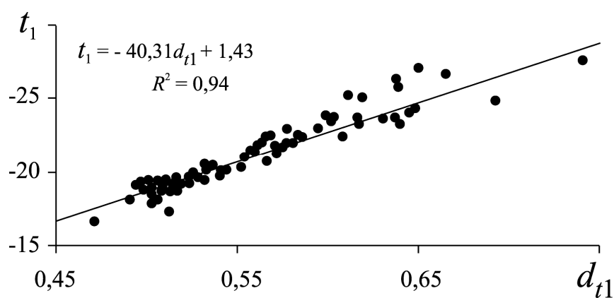
Рис. 5.3. Связь t_1 и d_{t1}
