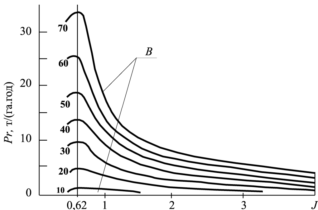
Рис. 6.1. Зависимость P_r от J и B .
