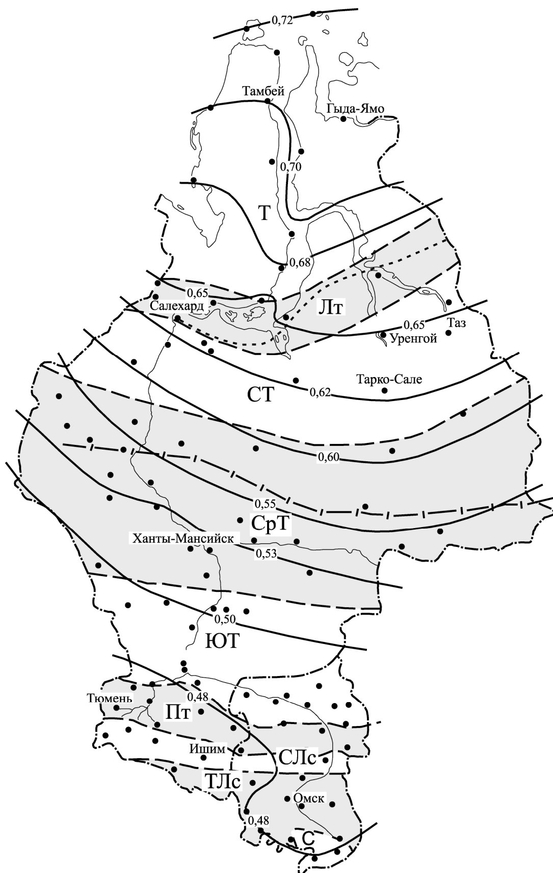
Рис. 5.17. Изолинии d_{tx} (остальные обозначения по рис. 5.11)
