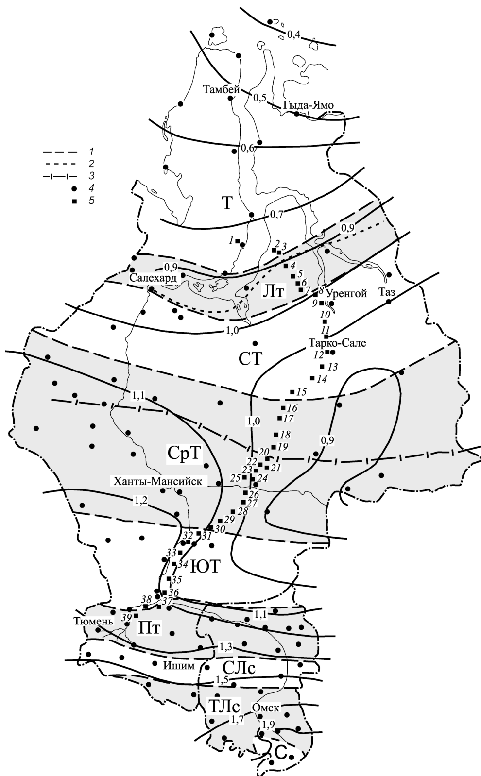
Рис. 4.1. Изолинии J
