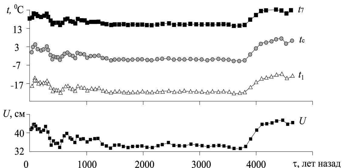
Рис. 8.1. Ход характерных температур воздуха и осадков в Сладково.
