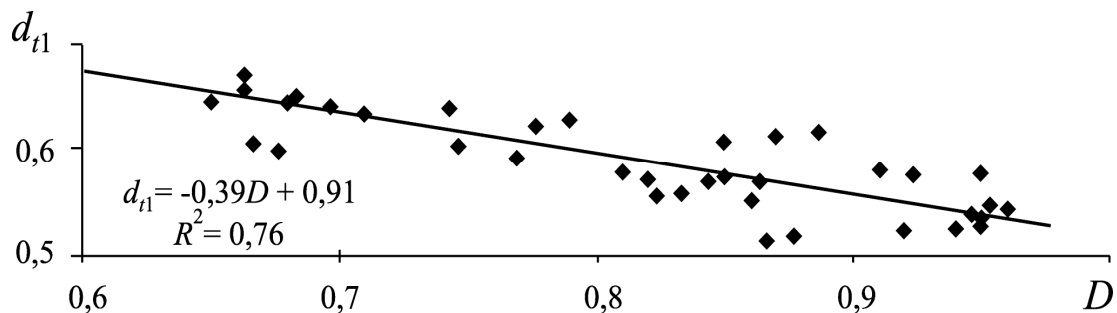
Рис. 7.2. Связь D и d_{t1}
