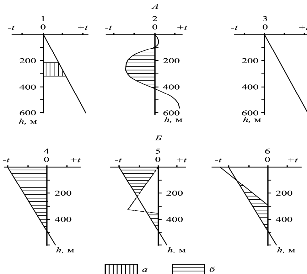
Рис. 5.20. Принципиальная схема образования многоярусного криогенного строения горных пород при разложении газгидратов (А) и в разных условиях засоленности (Б).
