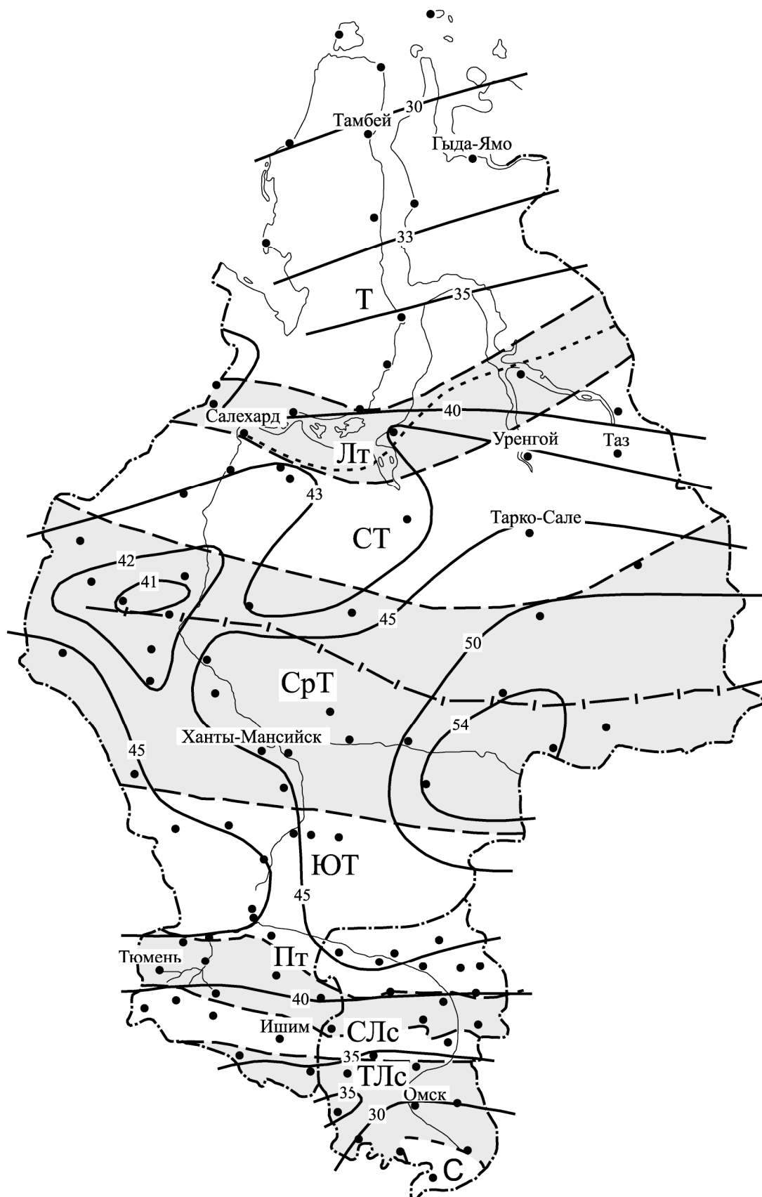
Рис. 5.15. Изолинии U (остальные обозначения по рис. 5.11)
