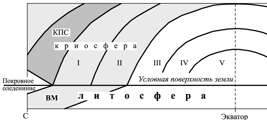
Рис. 2.4. Схематический меридиональный разрез биосферы:
