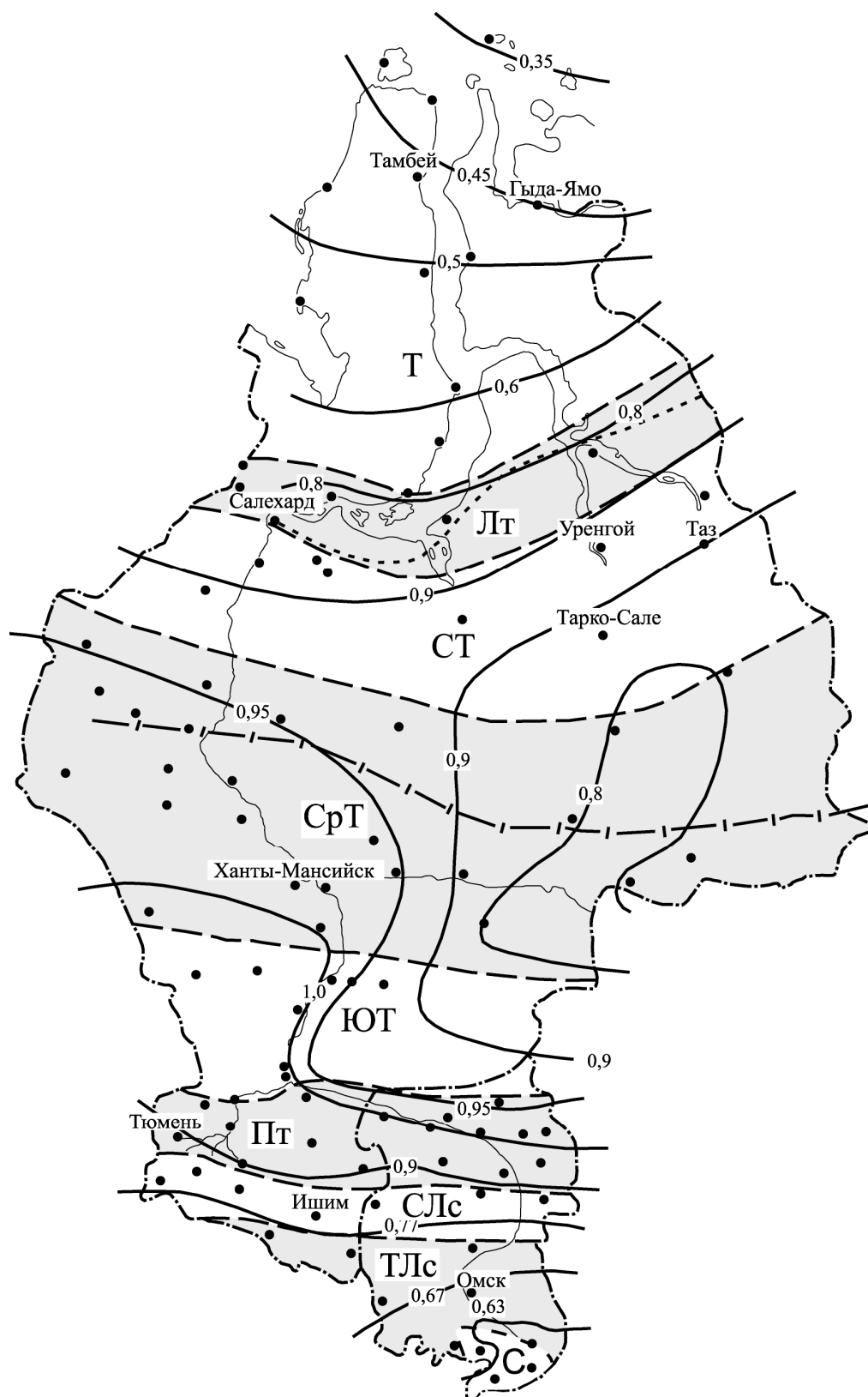
Рис. 4.2. Изолинии расчетной величины D (обозначения по рис. 4.1)
