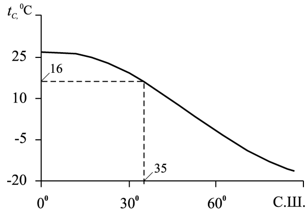
Рис. 3.1. Распределение среднеширотной температуры воздуха t_c , °C.
