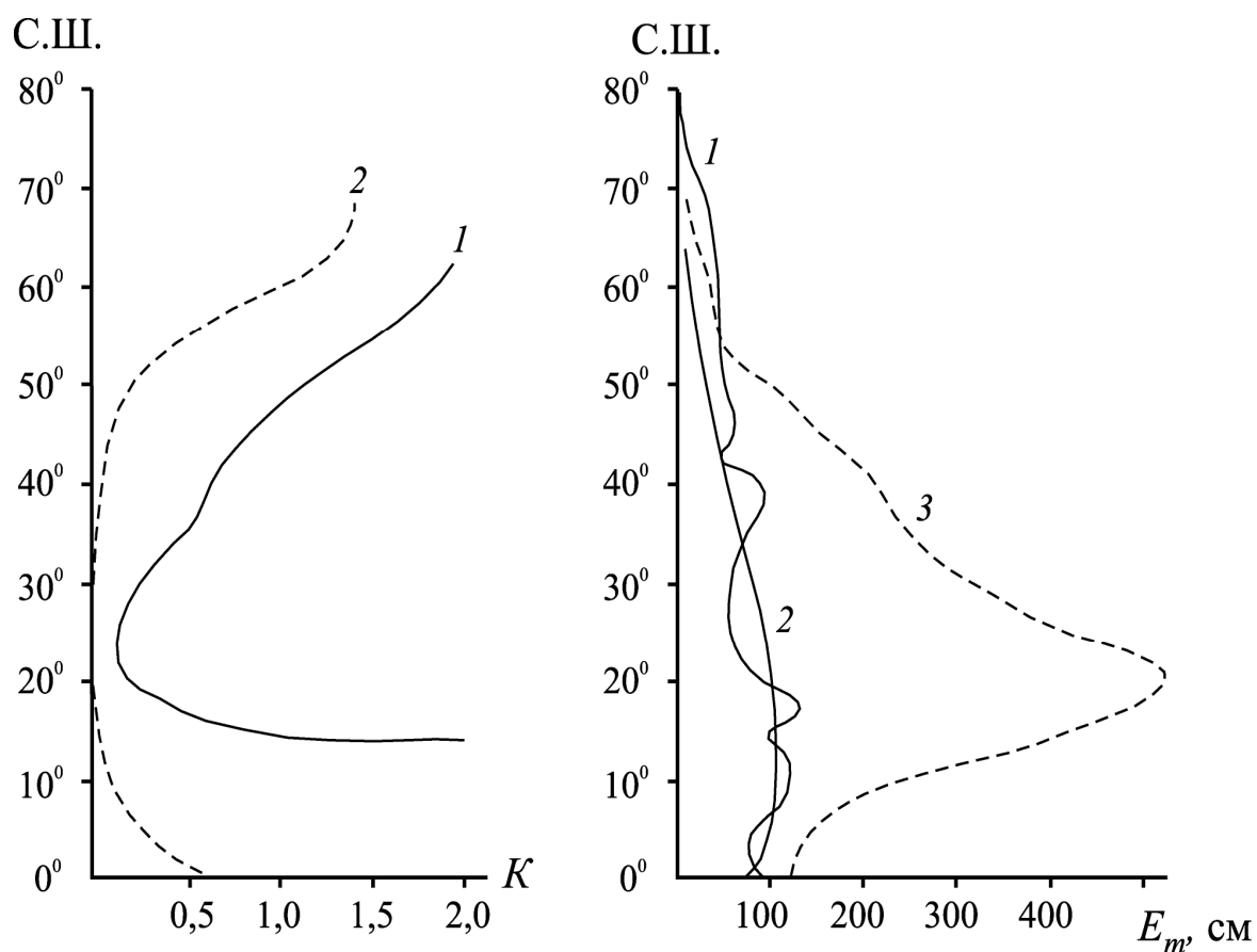
Рис. 2.3. Зональное распределение годовых величин K и E_m Секторы: 1-приатлантический, 2-притихоокеанский, 3-континентальный.
