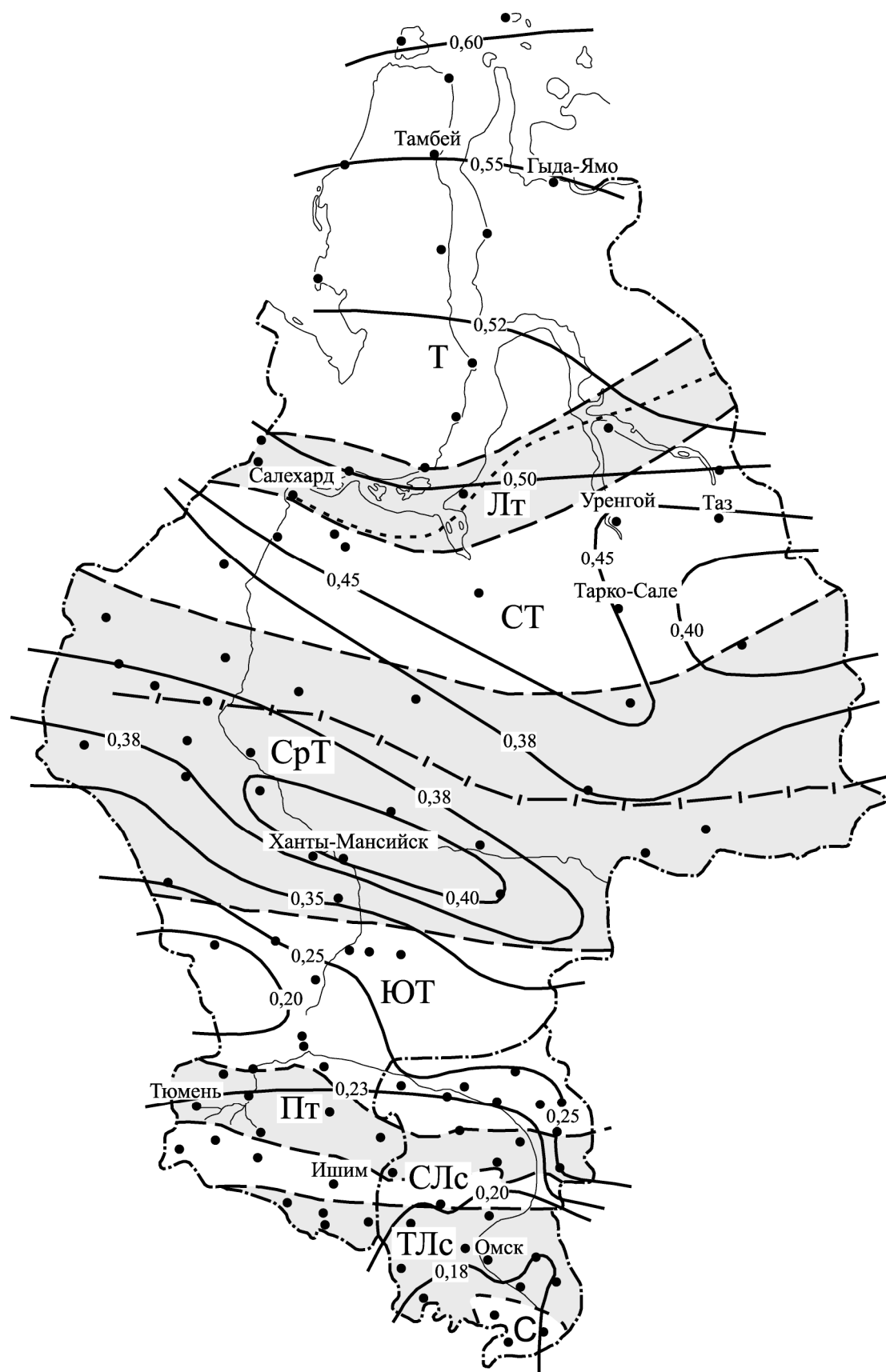
Рис. 5.16. Изолинии d_{ux} (остальные обозначения по рис. 5.11)
