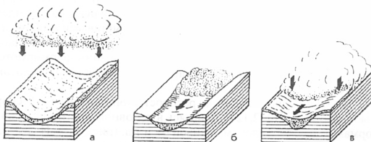
Рис. 11. Схематические представления о механизмах образования пирокластических отложений: а: пеплы облаков пирокластических потоков отлагаются слоем равной мощности на потоках и вокруг них; б: отложения пирокластических потоков залегают согласно рельефу - в долинах; в: отложения пирокластических волн имеют разные мощности на возвышенностях и в долинах - формируются из приземного пирокластического облака, испытывающего гравитационное воздействие.
