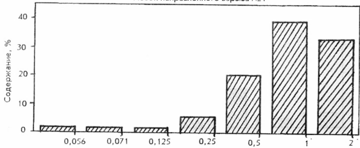
Песок направленного взрыва №2
