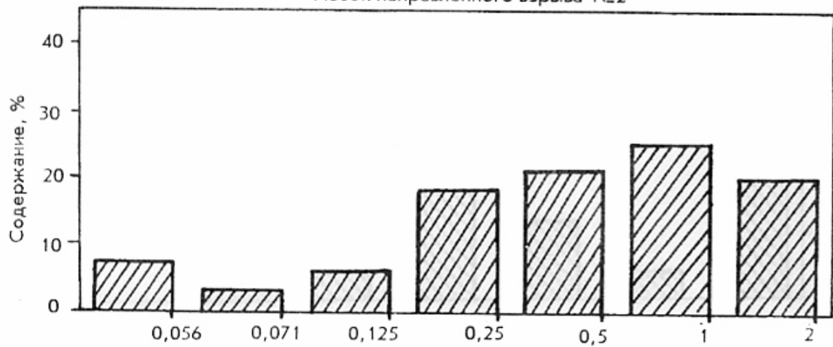
Агломерат направленного взрыва
