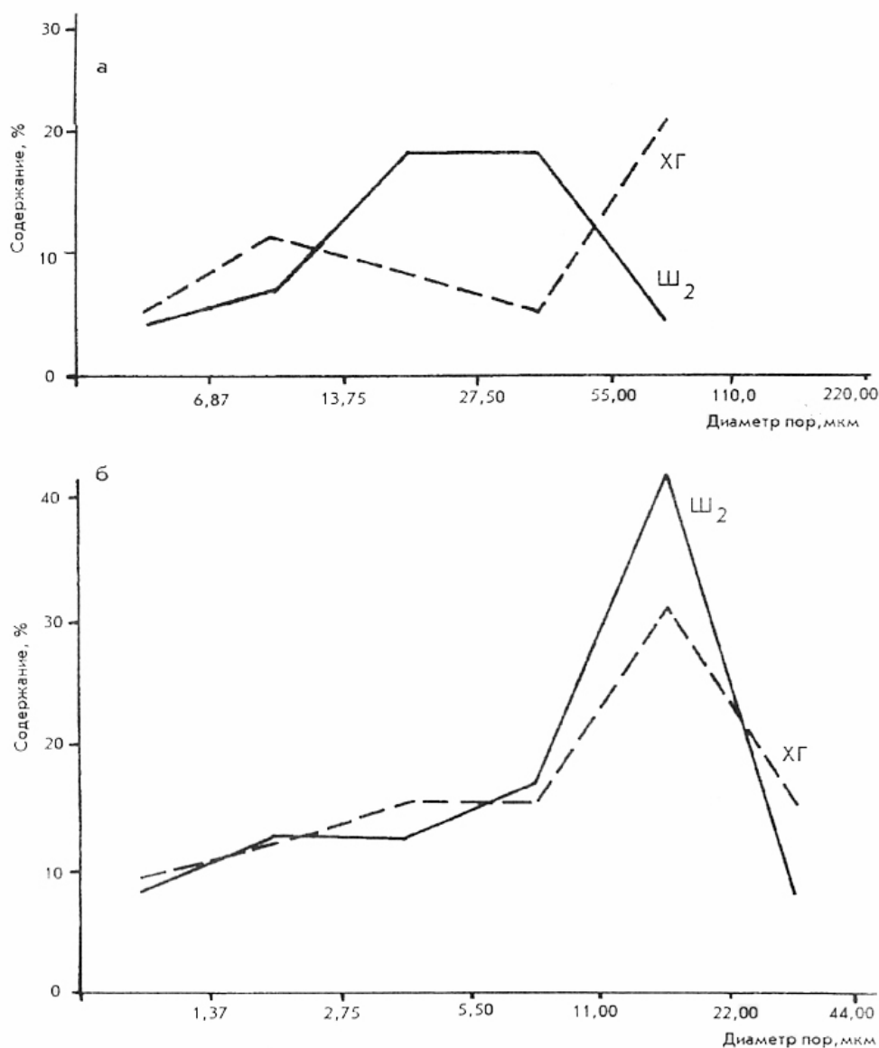
Рис. 9. Кривые распределения пор разного диаметра в образцах ненарушенного строения тефры вулканов Шивелуч (Ш 2 ) и Хангар (ХГ) при увеличениях 200 (а) и 1000 (б).
