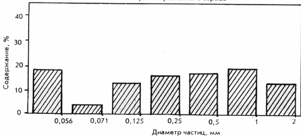
Агломерат направленного взрыва
