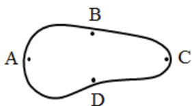
Рис.1.Схема расположения контактов при измерении методом Ван-дер-пау.
