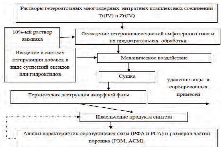
Рис. 2 – Технологическая схема получения продукта по М – 2
