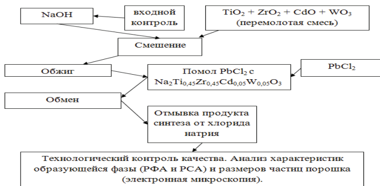
Рис. 1 – Принципиальная технологическая схема синтеза целевой фазы по М – 1
