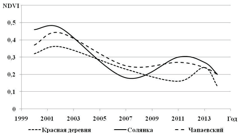
Рисунок 1 - Динамика NDVI на тестовых полигонах
