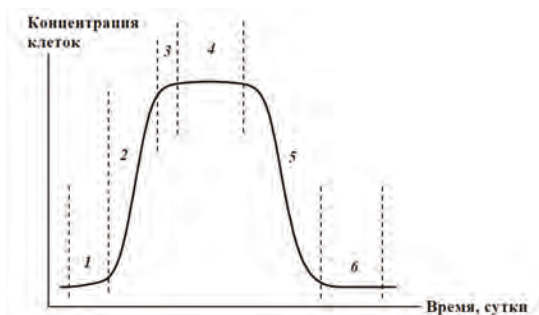
Рисунок 2. Кривая роста микроорганизмов: 1 – латентная фаза (лаг - фаза); 2 – фаза роста с постоянной скоростью (экспоненциальная фаза); 3 – фаза замедления скорости роста; 4 – фаза стационарного равновесия; 5 – фаза отмирания; 6 – фаза уменьшения скорости отмирания
