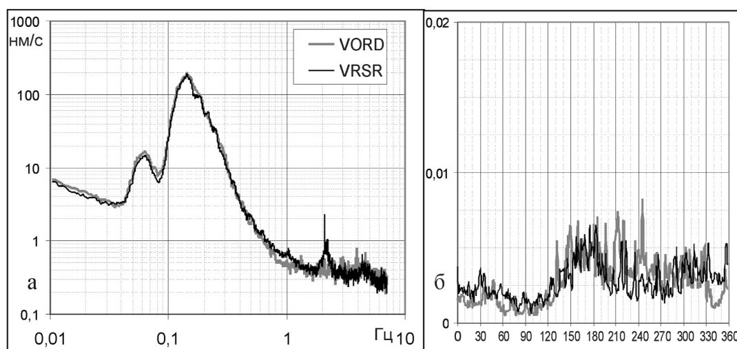
Рис. 4.5. Спектральный состав Z-компоненты микросейсмического процесса во время сейсмической бури и распределение частот азимутов преимущественных колебаний его на станциях «Дивногорье» (VORD) и «Сторожевое» (VRSR) в один и тот же момент времени
