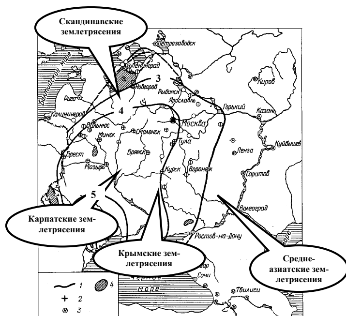
Рис. 2.1. Карта изосейст (равных сотрясений) глубокофокусно-го Карпатского землетрясения 4 марта 1977 г. (по Ананьину): 1 — изосейсты, баллы; 2 — эпицентр землетрясения; 3 — пункты, где землетрясение не ощущалось; 4 — участки пониженной интенсивности сотрясений. Выносками показаны области далеких землетрясений
