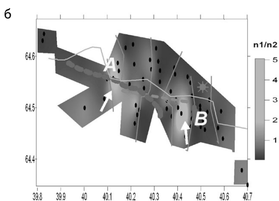
Рис. 3.5. Карты интенсивности (а) и анизотропии (б) эндогенного сейсмического излучения для частоты 2,2 Гц
