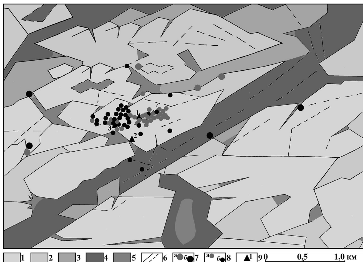
Рис. 5.10. Схема блоковой делимости участка Паанаярви и пространственное распределение эпицентров микросейсмических событий, зарегистрированных с 4 по 11 июля 2004 г.:
