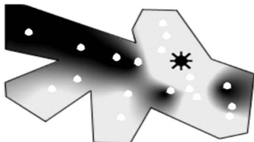
Рис. 3.3. Карты медианных значений амплитуд с учетом тренда, определяемого законом ослабления амплитуды с расстоянием
