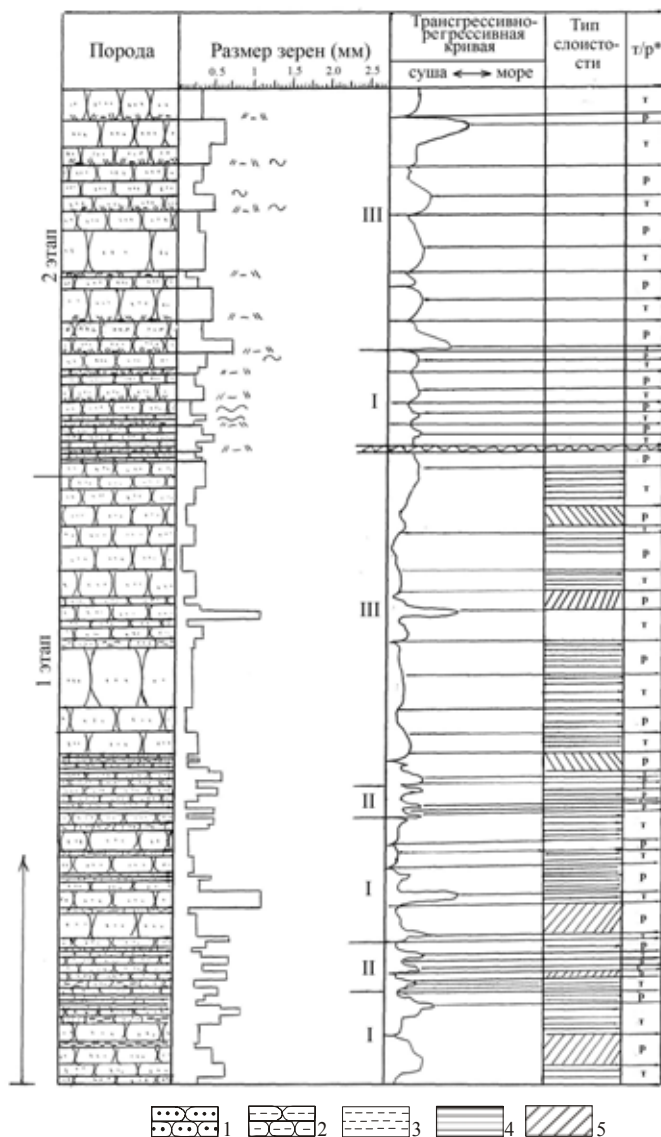
Рис. 1. Литологическая колонка и ритмограмма отложений джеджимской свиты верхнего рифея (карьер Асывовож-Р). Условные обозначения: 1 — песчаники, 2 — алевролиты, 3 — аргиллиты, 4 — горизонтальная слоистость, 5 — косая слоистость, *Т/Р — трансгрессия/регрессия.
