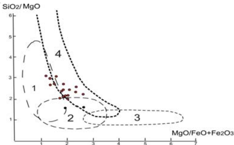
Рис. 3. Положение фигуративных точек составов лампрофиров Четласского выступа (Средний Тиман) на диаграмме \text{SiO}_2/\text{MgO} — \text{MgO}/(\text{FeO}+\text{Fe}_2\text{O}_3) . Поля: 1—алмазоносные кимберлиты внутренних районов Якутской провинции; 2—неалмазоносные и убогалмазоносные кимберлиты северных районов Якутской провинции; 3—альпикриты Чедобецкого комплекса; 4—лампроиты Австралии.
