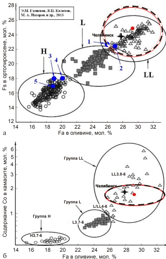
Рис. 6. Результаты классифицирования метеорита Челябинск по составу пороодообразующих минералов (а) и корреляции содержания кобальта в камасите и железистости оливина (б). Пунктирной линией показаны поля и точки средних значений критериев для метеорита Челябинск. Цифрами отмечены точки средних значений критериев для других каменных метеоритов, упавших на Землю в уральском регионе (Лобанов, Сергеева, 2002): 1 – Озерное-I, 2 – Озерное-II, 3 – Мокроусово, 4 – Урал, 5 – Свердловск.
