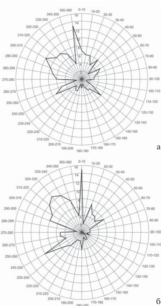
Рис. 1. Роза-диаграмма направлений спрямленных участков рек кряжей Енганепэ (а) и Манитанирда (б).
