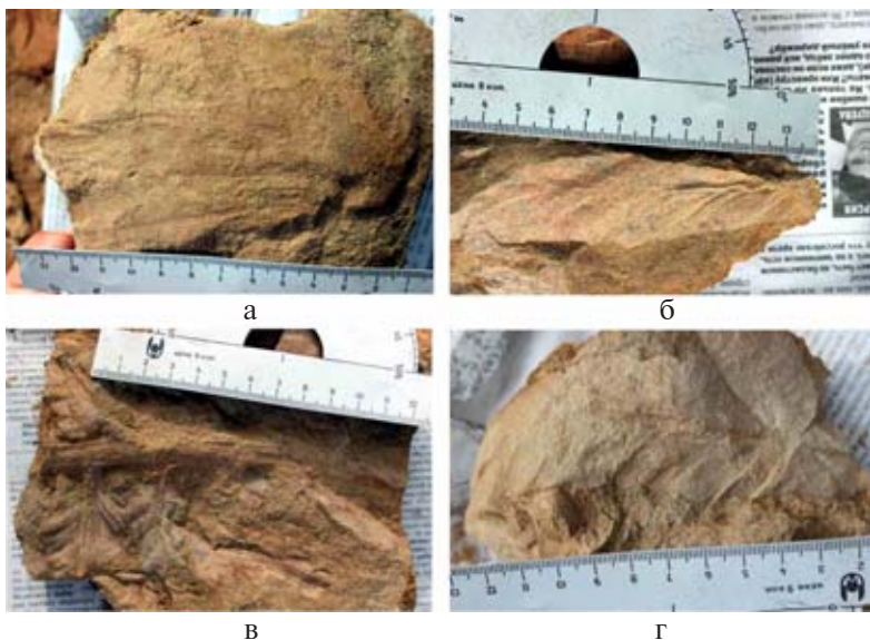
Рис.2. Образцы из местонахождения Зеглуд: а — листовая пластинка Psygmothallum expansum , б— фрагменты вай Odontopteridium (Rhachiphyllum) sp. , в — Rhachiphyllum wangenheimii , г — Rhachiphyllum wangenheimii .
