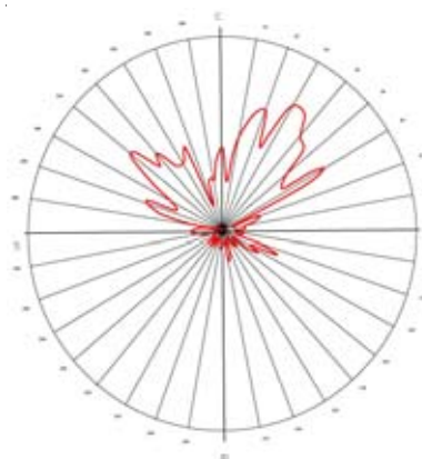
Рис. 2. Роза-диаграмма карьер-трещиноватости пород джежимской свиты верхнего рифея (карьер Асыввож-R).
