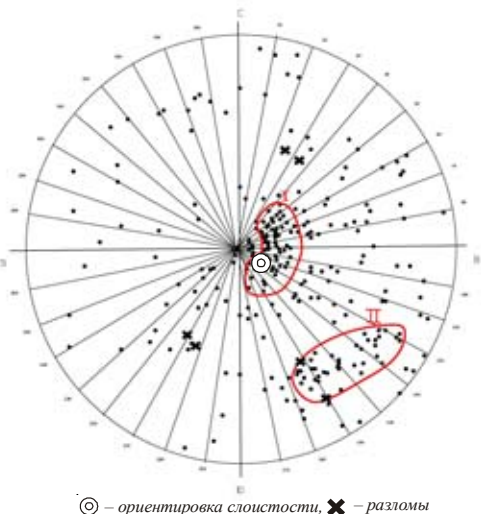
☉ — ориентировка слоистости, X — разломы Рис. 1. Точечная круговая диаграмма трещиноватости пород джежимской свиты верхнего рифея (карьер Асыввож—R).
