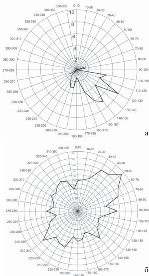
Рис. 3. Роза-диаграмма направлений спрямленных участков рек Пайпудынских хребтов (а) и Южного Тимана (б).
