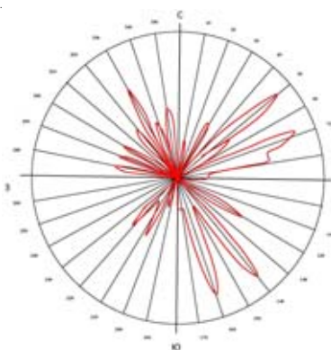
Рис. 4. Роза-диаграмма трещиноватости палеозойских пород ( D_{2-3}chr ) карьера Шераель Верхний.
