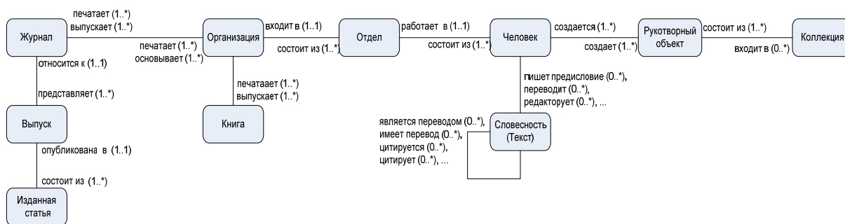
Рис. 6. Связи между сущностями в информационной модели научной электронной библиотеки
