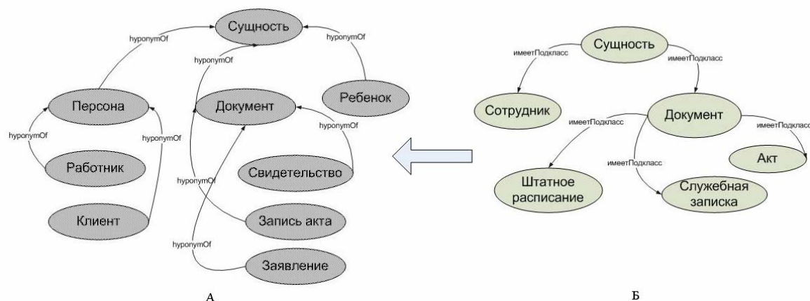
Рисунок 1. Расширение тезауруса терминами новой онтологии.
