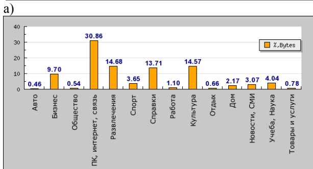
Рис.1 Ранговое распределение объема трафика по категориям для кэш-серверов
