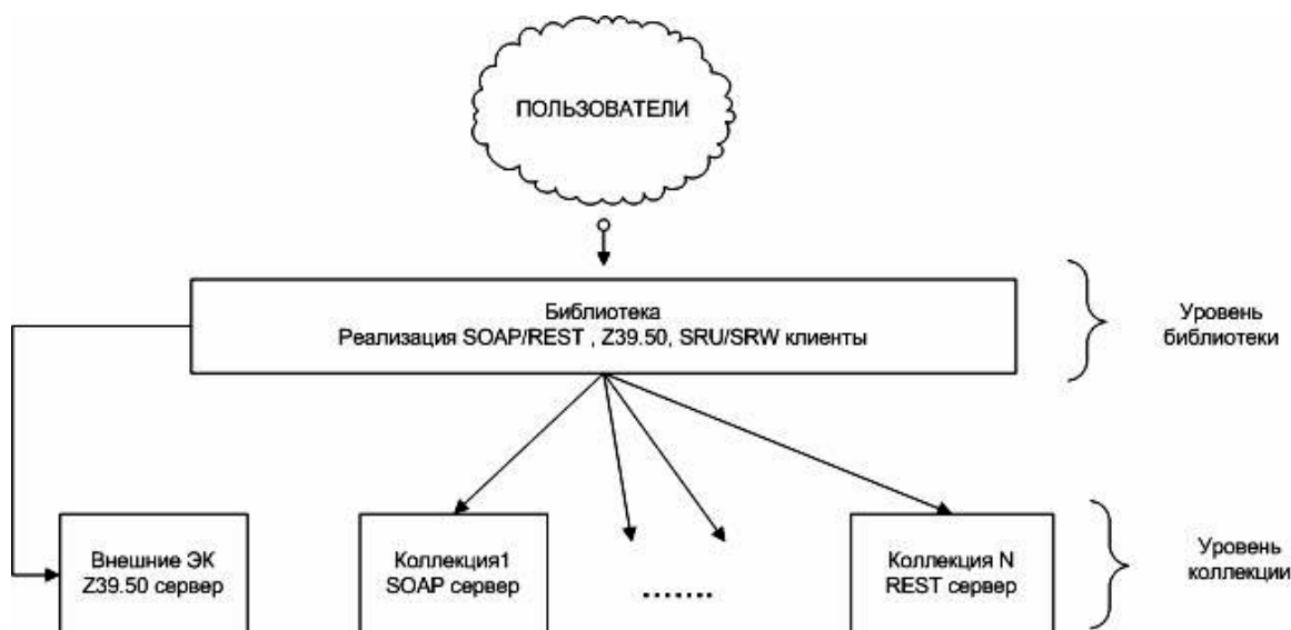
Рис. 2 Структура ПО системы ЭБ
