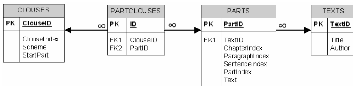
Рис. 1. Структура базы данных предназначенной для хранения синтаксической разметки
