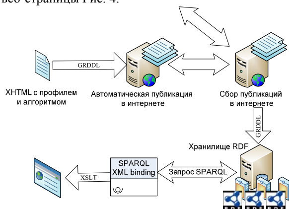
Рис. 4 Пример RDFa и GRDDL
