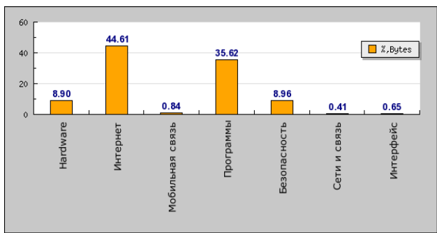
Рис.1 Ранговое распределение объема трафика по категориям для кэш-серверов
