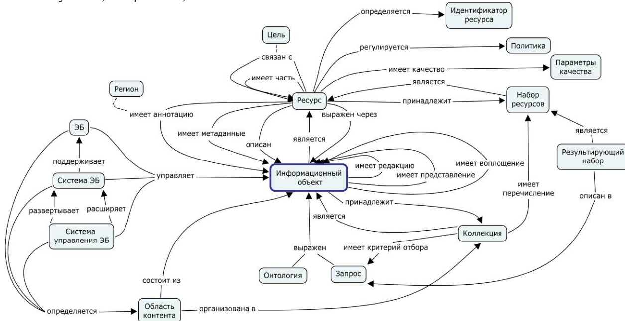
Рис. 4. Область контента ЭБ в модели DELOS DLRM
