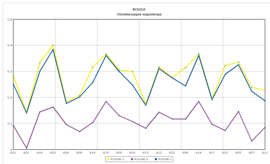
Рисунок 2 - Алгоритм Manifold Ranking является очень чувствительным к выбору темы. По горизонтальной оси отложены номера документов, заголовок которых был использован в качестве темы
