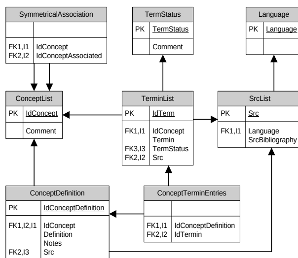
Рис.1. Структура реляционной базы данных глоссария: таблицы и поля, PK и FK(n) первичные и внешние ключи для обеспечения целостности данных, их каскадного изменения/удаления, подстановки, I(n)- индексированные поля. Стрелками показаны реляционные отношения (обычно один - ко многим).
