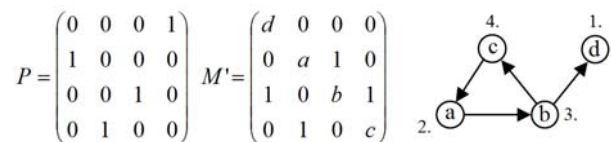
Рисунок 6. Матрица перестановки P и новая матрица смежности M'
