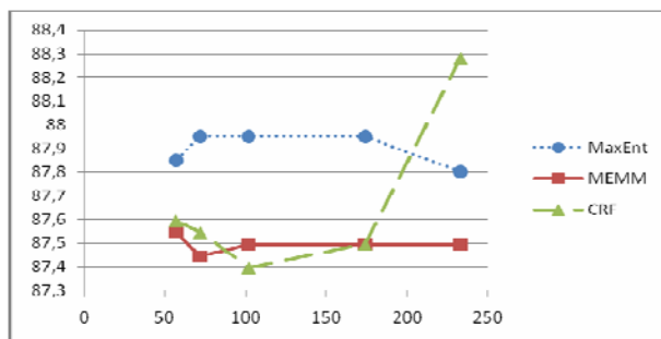
Рисунок 1. Сравнение показателя F-меры качества классификации обучаемыми методами при использовании различного объема словарных характеристик.
