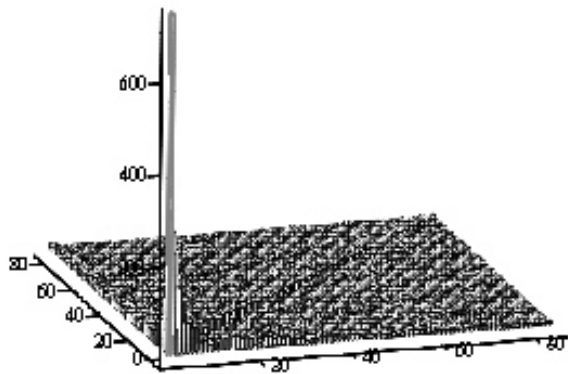
Рис.1.Изображение модифицированной матрицей связей M . По горизонтальным осям отложены номера узлов (персон), по вертикальной – весовые значения связей
