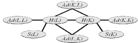
Рис 1. Марковская сеть, полученная из интерпретации формулы в таб. 1.
