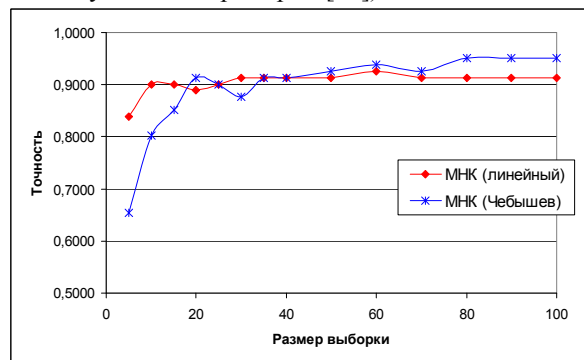
Рис. 1. Сравнение двух видов МНК.
