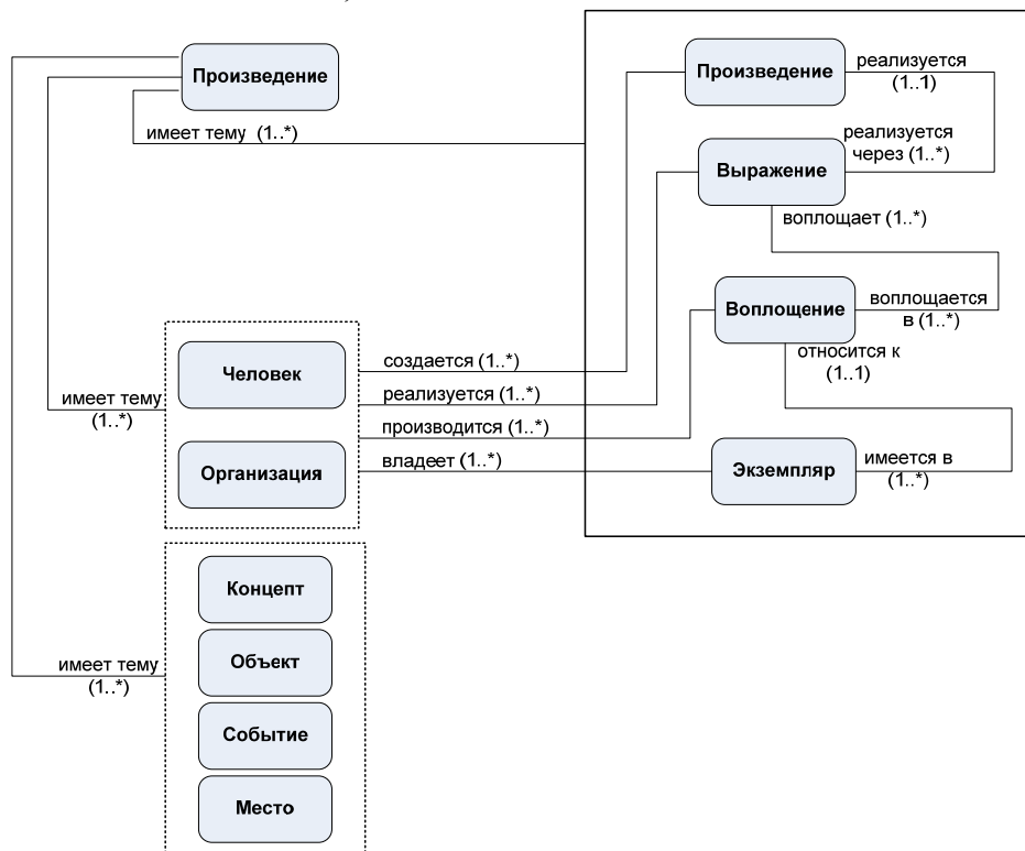
Рис. 2. Модель FRBR
