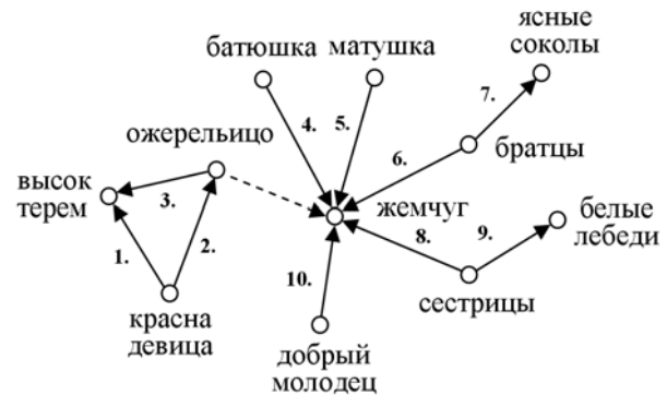
Рисунок 1. Теоретико-графовая модель фрагмента беседной песни «Как назябло, навяло лицо»
