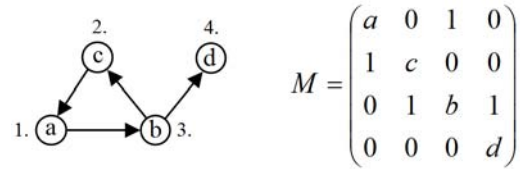
Рисунок 5. Граф G и его матрица смежности
