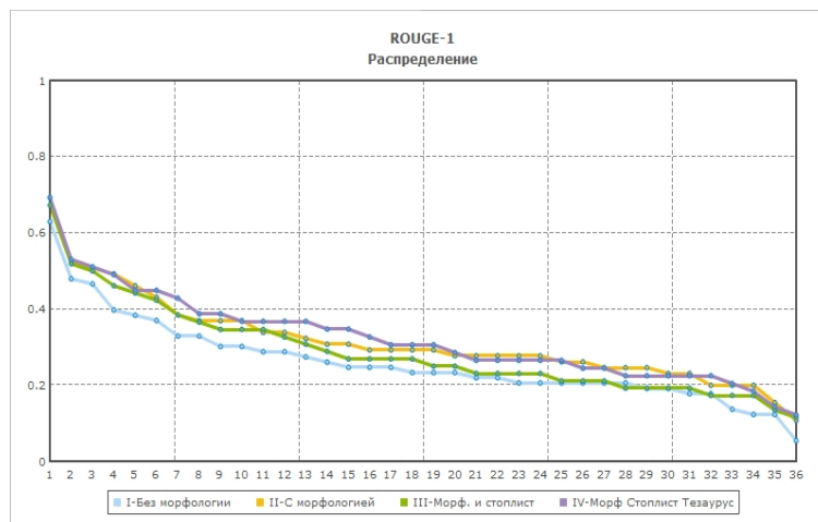
Рисунок 1 - Распределение величины ROUGE-1 при сравнении одной ручной аннотации со всеми остальными для произвольного кластера. Значения отсортированы по убыванию.
