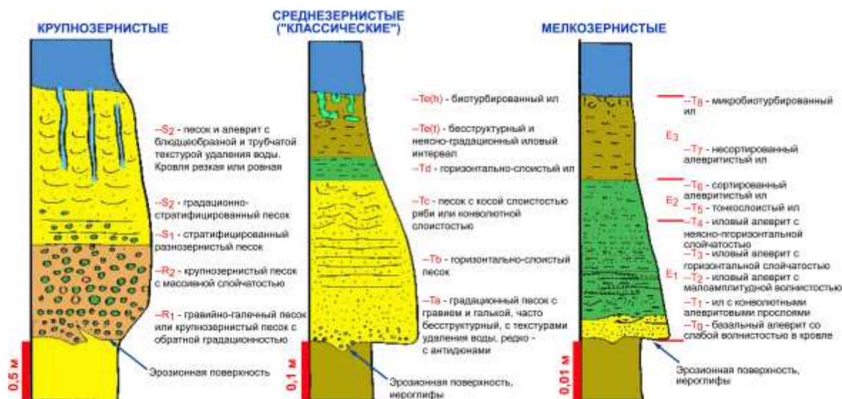
Рис. 2.18. Три типа турбидитов по плотности турбидитового потока: грубозернистые, классические и тонкозернистые. (А) по [Shanmugam, 2000]), (Б) с изменениями по [Барабошкин, 2011].
