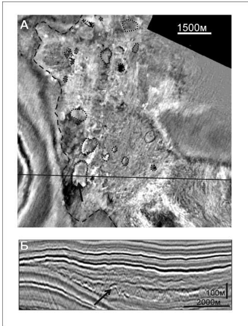
Рис. 3.20. Слайс по сейсмическому кубу для склона вала Шатского в Черном море (А) и сейсмический разрез к нему (Б). На рис. А пунктиром околнурены отдельные вероятные олистолитовые тела. Стрелкой показано одно и то же тело на слайсе и разрезе. [Митюков и др., 2012].
