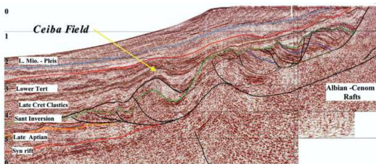
Рис. 6.16. Интерпретация сейсмического разреза для пассивной окраины Африки в Экваториальной Гвинее. Отложения альба-верхнего мела оползали по толще солей, образуя на дне моря относительные поднятия. Одно из таких поднятий препятствовало транспорту турбидитового материала в позднем мелу, и перед ним накопилось относительно большое количество турбидитовых песчаников. Песчаники стали резервуаром для месторождения Сейба [Dailly et al., 2002].
