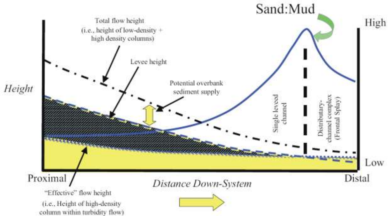
Рис. 4.49. Модель изменения турбидитовой системы вниз по склону. [Posamentier, Walker, 2006]. Effective flow height – высота высокоплотной колонны турбидитового потока, levee height – высота «леви», total flow height – общая высота колонны высокоплотного и низкоплотного потока, potential overbank sediment supply – зона потенциального привноса осадков за счет овербанка (наложенных сверху дополнительных отложений), single leveed channel – одиночные канал с «леви», Sand:mud – соотношения песчаного и глинистого материала в турбидитовом потоке, frontal splay (distributary channel complex) – фронтальный конус выноса с ветвящимся канальным комплексом. Proximal – проксимальные турбидиты, distal – дистальные турбидиты. В точке перехода от канала с «леви» к фронтальному конусу наблюдается относительно наибольшее количество песчаной фракции.
