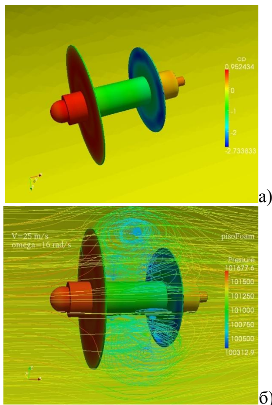
Рис. 1. Расчет обтекания диагностического комплекса «Сканлайнер»: а) коэффициент давления C_p ; б) значения поля давления и линии тока
