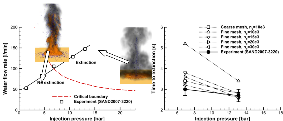
Рис.1. Моделирование подавления пламени [4]: а) – критические условия подавления пламени и результаты экспериментов (визуализация пламени с помощью FDS-Smokeview); б) – измеренное и расчётное время подавления пламени ( n_d – количество вычислительных частиц, выпускаемых за 1с).
