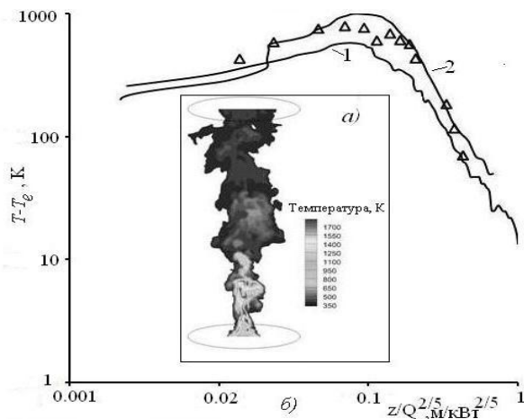
Рис. 1. а) Мгновенное поле температуры. б) Распределение осредненной температуры вдоль вертикальной оси для пламени мощностью 37,9 кВт. 1- расчет FDS, 2 – расчет, FireFOAM, маркеры – эксперимент [3]
