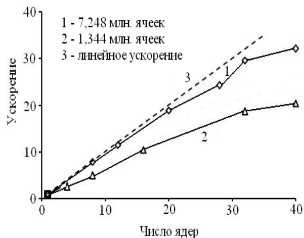
Рис. 2. FireFOAM, зависимость ускорения от числа ядер при оптимальном размещении процессов по узлам кластера
