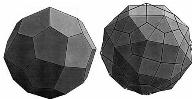
Рис. 9. Пентагонтриоктаэдр дуален комбинации куба, октаэдра и (!) пентагонтриоктаэдра.
