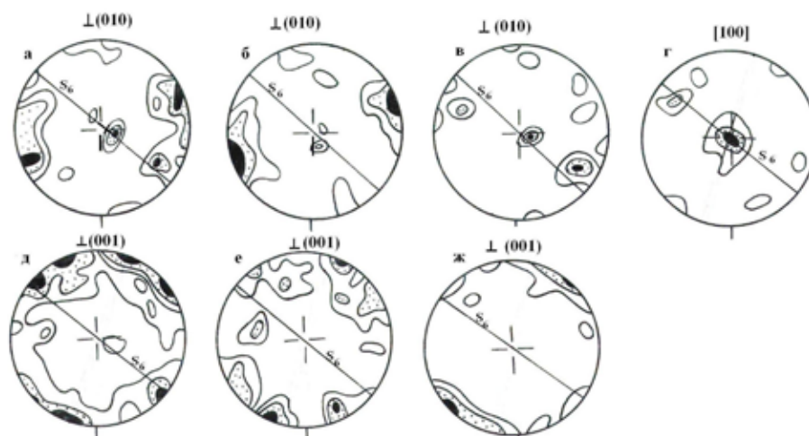
Рис. 2. Микроструктурные ориентировки осей \perp(010) , \perp(001) и [100] плагиоклаза из гнейсов \gamma_1 : а – плагиоклаз-I, II (изолинии 2.5-4.2-5.9 %, n = 60 ), б – плагиоклаз-I (изолинии 1.8-5.3-8.9 %, n = 30 ); в – плагиоклаз-II (изолинии 5.0-8.3-11.7 %, n = 30 ), г – плагиоклаз-I, II (изолинии 2.5-4.2-9.1 %, n = 60 ), д – плагиоклаз-I, II (изолинии 2.5-4.2-5.9 %, n = 60 ); е – плагиоклаз-I (изолинии 1.8-5.3-8.9 %, n = 30 ); ж – плагиоклаз-II (изолинии 5.0-8.3-11.7 %, n = 30 ); з – плагиоклаз-II (изолинии 5.0-8.3-11.7 %, n = 30 ). S_6 – сланцеватость этапа D_6 . В центр диаграммы проецируется линейность L_6 .
