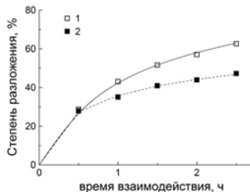
Рис. 8. Зависимость степени разложения образцов титанита, механоактивированных в течение 5 мин., от продолжительности взаимодействия с серной кислотой при 40 °C: 1 – сухая МА, 2 – мокрая МА. Экспериментальные и расчётные данные представлены символами и линиями соответственно.
