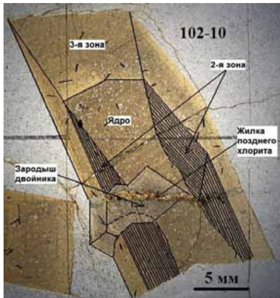
Рис. 3. Начальная фаза зарождения двойника: зародыш двойника наблюдается в клинообразном врезе кристалле ставролита. Элементы внутреннего строения кристаллов: 1 – ядро, 2 – вторая зона, 3 – третья зона. Весь двойник пересекается поздней жилой хлорита. Фрагмент косого двойника. Чёрные включения – ильменит.
