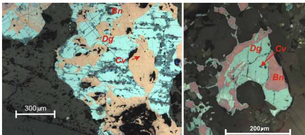
Рис. 3. Полифазные агрегаты борнита (Bn), дигенита (Dg) и ковеллина (Cv). Отраженный поляризованный свет.
