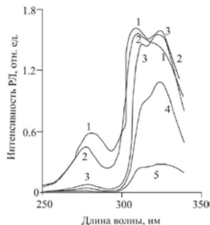
Рис. 2. Спектры РЛ K_2ZrF_6 с Ce(III) . Добавка Ce^{+3} , ppm: 1 – 1, 2 – 10, 3 – 50, 4 – 150, 5 – 200.
