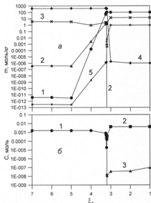
Рис. 4. Изменение состава раствора (а) и содержания твёрдых фаз (б) в системе Fe – CuSO 4 в зависимости от \xi_1 . а) Концентрации: 1 – Cu 2+ ; 2 – Cu + ; 3 – H + ; 4 – Fe 2+ ; 5 – Fe 3+ ; б) содержания: 1 – Cu; 2 – Fe 2 O 3 ; 3 – FeOOH.
