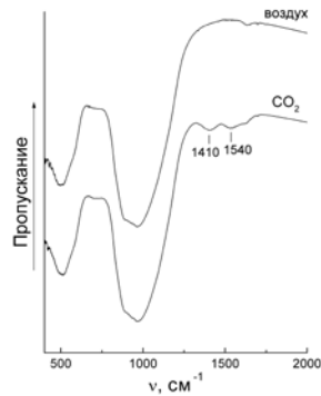
Рис. 2. ИК спектры шлака после МА воздушной среде и в \text{CO}_2 .
