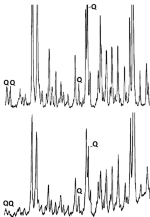
Рис. 4. Дебаеграммы бледно-жёлтого кианита с примесью кварца (Q) до (вверху) и после опыта (внизу). Д.Л. Рогачёв, Е.А. Селиванова.
