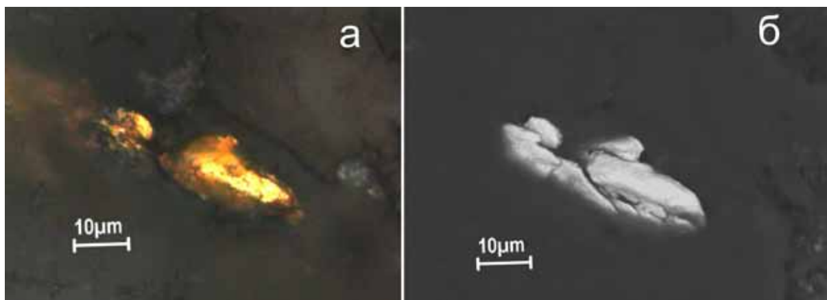
Рис. 4. Минеральная фаза \text{Cu}_2\text{Zn} в отражённом свете (а) и отражённых электронах (б).
