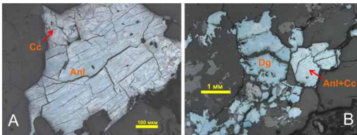
Рис. 4. Минералы группы халькозина из кварц-карбонатных жил.
