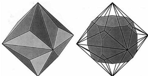
Рис. 7. Тригонтриоктаэдр дуален кубу, усечённому гранями октаэдра.
