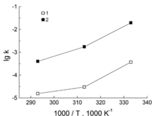
Рис. 9. Зависимость \lg K^{\text{cr}} от обратной температуры: 1 – сухая МА, 2 – мокрая МА.
