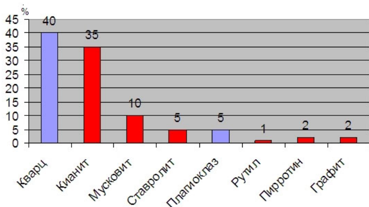
Рис. 8. Содержание главных минералов кианитовых руд.
