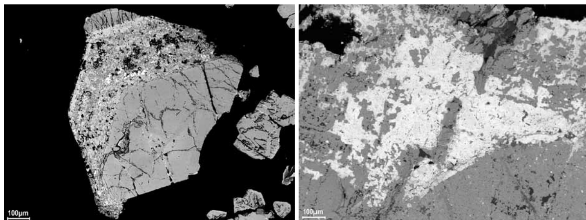
Рис. 4. Высокая степень фазовой неоднородности «кремового» циркона. РЭМ, BSE-изображения. а – кайма «кремового» циркона на обломке «шоколадного», б – скопление включений торита (светло-серое).
