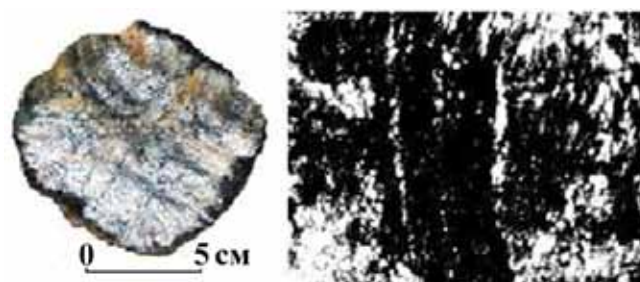
Рис. 5. Слева: поперечный срез параморфозы кианита. Справа: шлиф чёрной оторочки параморфозы, без анализатора.
