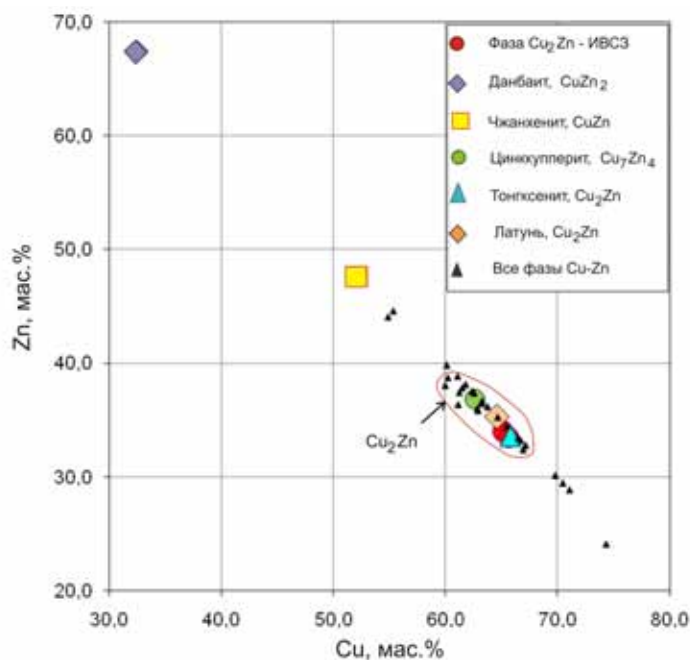
Рис. 5. Диаграмма составов природных фаз Cu-Zn.
