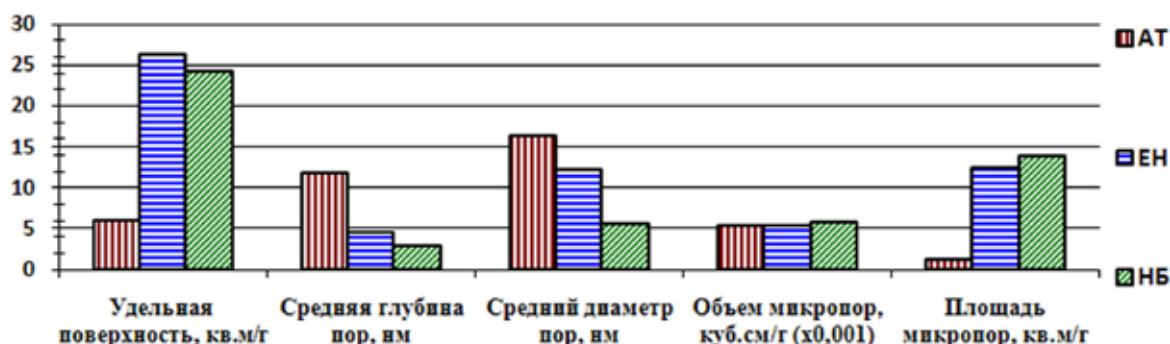
Рис. 3. Гистограммы характеристик пористости на газоанализаторе TtiStar 3020.
