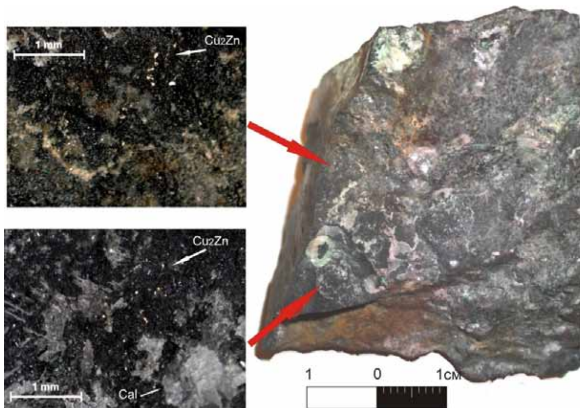
Рис. 3. Выделения минеральной фазы \text{Cu}_2\text{Zn} в образце миндалевидного диабаза. Снимки слева: темное – силикаты, светло-серое – кальцит. На снимке справа отчетливо видны миндалины, выполненные кальцитом и сульфидами меди в центре.
