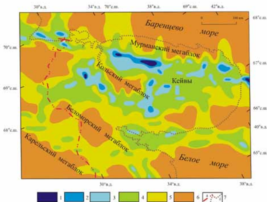
Рис. 1. Характер распределения градиентов напряжений, рассчитанных для архея – интервал 2.9-2.6 млрд. лет назад. 1-6 – нормированные градиенты напряжений: 1 – 80 \div 100 %, 2 – 60 \div 80 %, 3 – 40 \div 60 %, 4 – 20 \div 40 %, 5 – 10 \div 20 %, 6 – 0 \div 10 %; 7 – а) государственная граница России, б) современная береговая линия.
