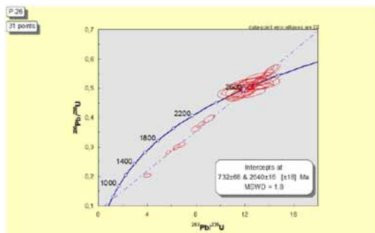
Рис. 9. Изохронная диаграмма с конкордией для циркона из пробы П-26.
