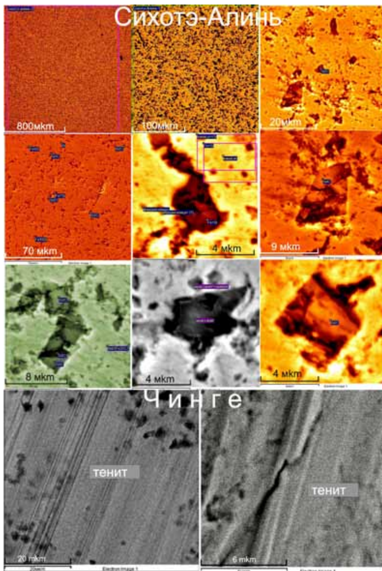
Рис. 13. Железные метеориты Сихотэ-Алинь (октаэдрит) и Чинге.
