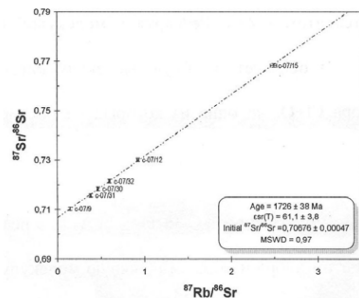
Рис. 3. Rb-Sr-изохрона для образцов базальтов ильмозёрской и панареченской свит.
