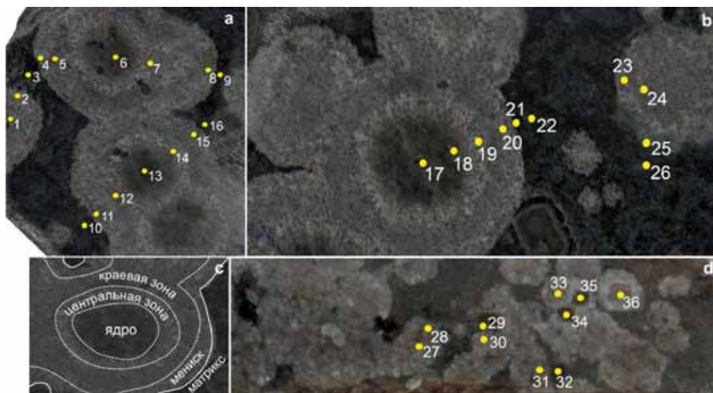
Рис. 2. Внутреннее строение вариолей и положение точек LA-ICP-MS анализа: а, б – крупные зональные вариолы в кровле массивного лавового потока; с – внутренняя зональность глобул; д – зона микровариолей в лавовом потоке.
