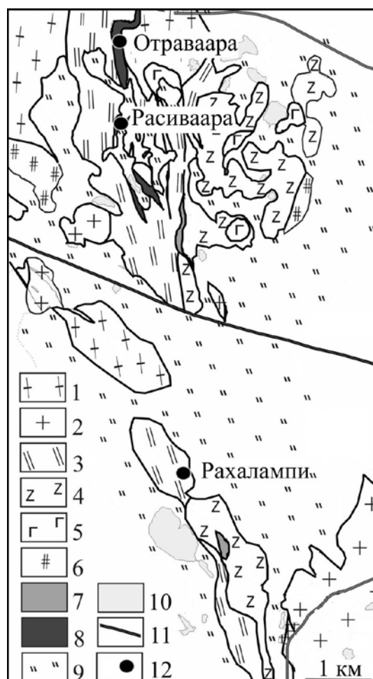
Рис. 1. Геологическое строение сланцевого пояса Коверо (К.А. Новосёлов и др.): 1 – гнейсы; 2 – граниты; 3 – кристаллические плагиоклаз-амфиболовые сланцы; 4 – амфиболиты; 5 – метагабброиды; 6 – кварц-полевошпат-слюдистые сланцы; 7 – серпентиниты; 8 – сульфидная минерализация; 9 – болота; 10 – озёра; 11 – дороги; 12 – рудопроявления.
