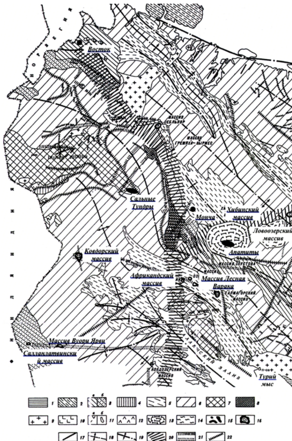
Рис. 1. Тектоническая схема западной части Кольского п-ова (по А.В. Галахову [4]) и размещение исследованных объектов. Условные обозначения: 1 – слабо дислоцированные девонские отложения; 2 – докембрийские дислоцированные отложения; 3 – синклинии, сложенные преимущественно вулканогенно-осадочными породами протерозоя и нижнего палеозоя (а – верхний структурный ярус, б – нижний структурный ярус); 4 – синклинии, сложенные гнейсами и сланцами протерозоя; 5 – синклинии гнейсовых комплексов архея; 6 – архейские гнейсы, граниты, включающие мегматиты и основные интрузивные породы; 7 – основные породы верхнего архея; 8 – основные породы протерозоя; 9 – граниты протерозоя; 10 – основные и ультраосновные породы протерозоя и, предположительно, нижнего палеозоя; 11 – протерозойские щелочные интрузии, щелочные граниты (а) и щелочные и нефелиновые сиениты Сахариокского и Кургинского массивов (б); 12 – комплексы габбро-сиенитов, нефелиновых сиенитов и щелочных гранитов массива Гремяха-Вырмес. Герцинские (?) щелочные интрузии: 13 – нефелиновые сиениты и мельтейгид-уртиты Хибинского массива; 14 – луювриты, фойяиты, уртиты и эвдиалитовые луювриты Ловоозерского массива; 15 – щелочные и нефелиновые сиениты мелких массивов; 16 – каледонские многофазные интрузии щелочных ультраосновных пород; 17 – дайки габбро-диабазов; 18 – оси антиклинориев; 19 – оси синклинориев; 20 – зоны глубинных разломов, простирающихся до поверхности Мохоровичича; 21 – глубинные разломы в докембрийском фундаменте; 22 – разломы, расколы и трещины небольшой глубины заложения. Синим цветом подчеркнуты названия исследованных объектов.
