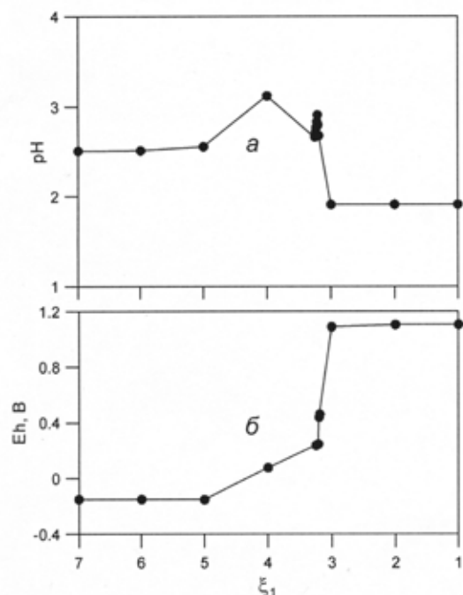
Рис. 3. Изменение pH (а) и Eh (б) системы Fe – CuSO 4 в зависимости от \xi_1 .
