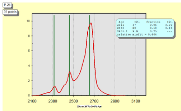
Рис. 8. PD-график для циркона из пробы П-26.
