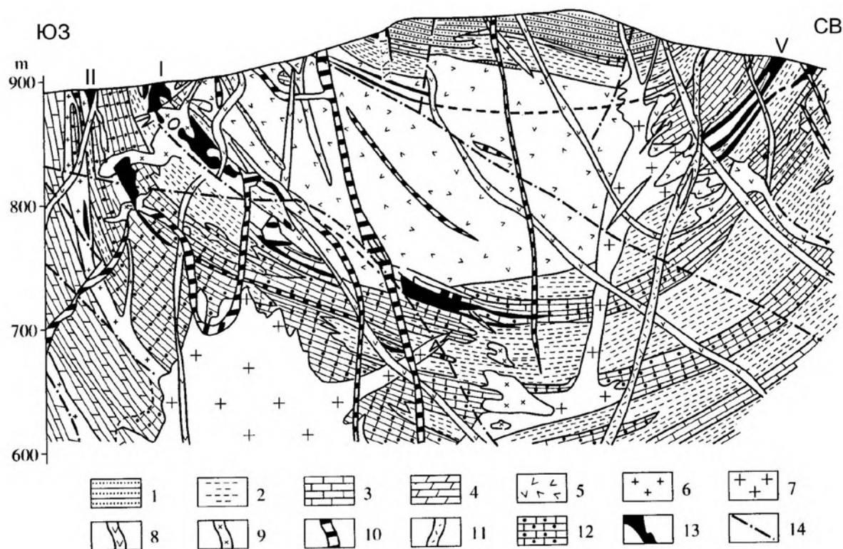
Рис. 14. Позиция Ермаковского месторождения в борту Кижингино-Кудунской рифтогенной впадины.
