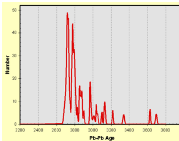
Рис. 4. PD-график для циркона из пробы П-21.
