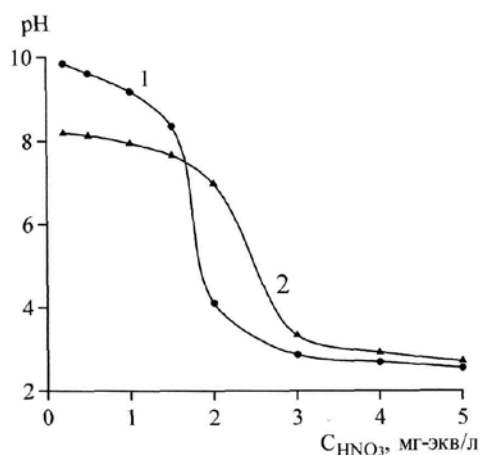
Рис. 1 Результаты потенциометрического титрования при различной продолжительности взаимодействия – 1 сут. (серия A1) и 30 сут. (серия A30).
