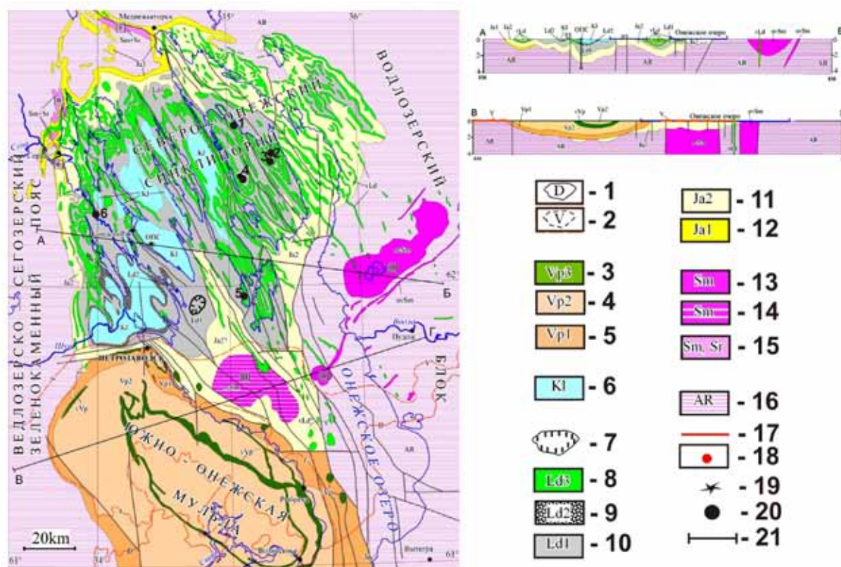
Рис. 7. Схема строения Онежской структуры
