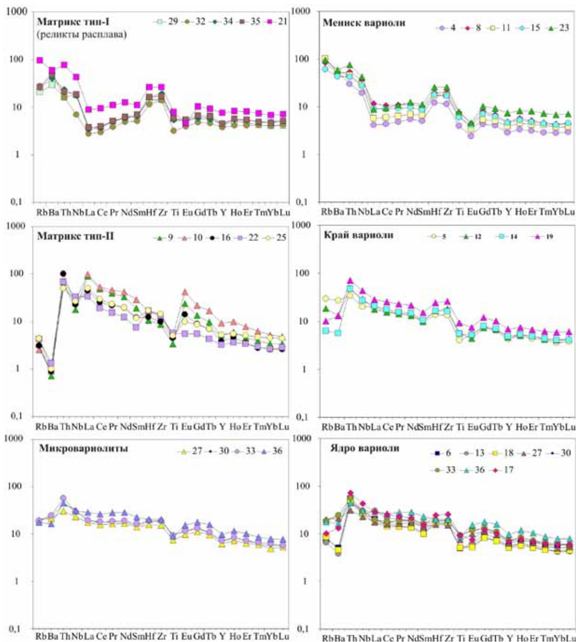
Рис. 3. Распределение редких и редкоземельных элементов в ликвационных образованиях по данным LA-ICP-MS анализа.
