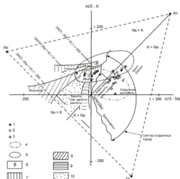
Рис. 4. Положение гнейсов кольской серии района Пулозеро–Полнек-Тундры на диаграмме Al/3-Na vs Al/3-K [12]. 1 – умереннокальциевые гнейсы; высококальциевые гнейсы: 2 – гранат-биотитовые, 3 – биотитовые; поля архейских супракrustальных пород: 4 – кольский комплекс Терского, Титовского и Аннамско-Хихнаярвинского блоков [7], 5 – кольский комплекс Центрально-Кольского блока [1]; поля составов: 6 – базальты; 7 – спилиты; 8 – вулканы щелочно-натрового атлантического типа (и соответствующих щелочных интрузивных пород); 9 – вулканы известково-щелочного тихоокеанского типа (и известково-щелочных интрузивных пород); 10 – вулканы промежуточного типа (и интрузивных пород того же состава).
