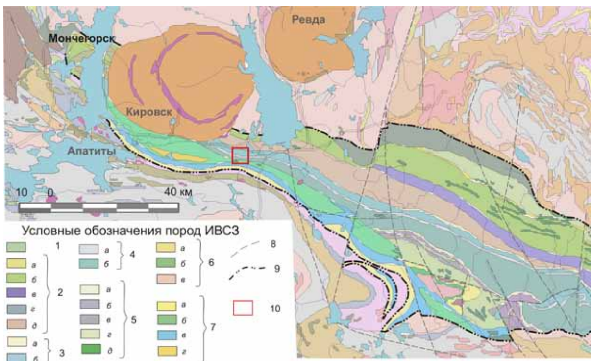
Рис. 1. Схема геологического строения Имандра-Варзугской структурной зоны (ИВСЗ) [17] (с упрощениями).
