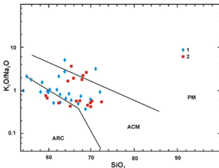
Рис. 7. Диаграмма K_2O/Na_2O - SiO_2 по [13]. Бассейны тектонической обстановки: РМ – пассивных окраин, АСМ – активных континентальных окраин, АРС – океанических дуг. 1 – умереннокальциевые гнейсы кольской серии, 2 – высококальциевые гнейсы кольской серии.
