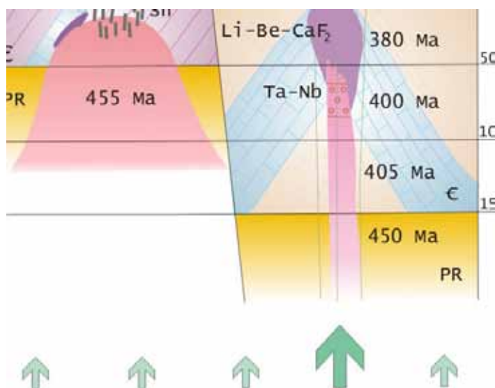
Рис. 18. Схема формирования редкометально-флюоритового Вознесенского месторождения (справа) и оловорудного Ярославского (слева).
