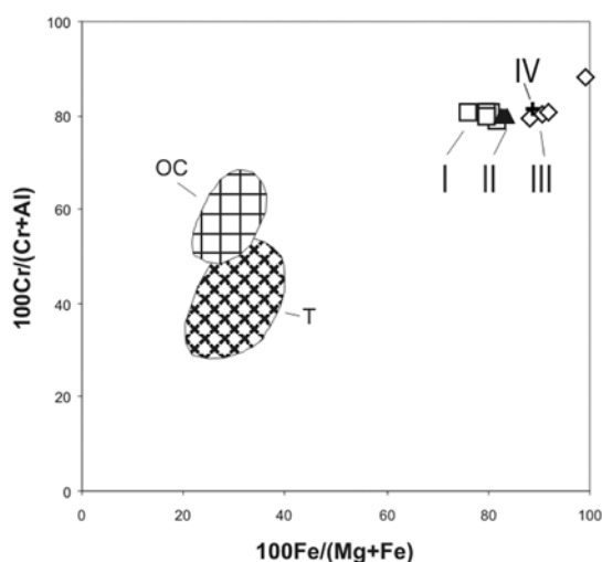
Рис. 2. Соотношение хромистости и железности хромшпинелидов: I – из коматиитов массива Кауниинлампи (Суомуссалми); II – из коматиитов массива Вара (Суомуссалми); III – из серпентинитов западной части пояса Иломантси; IV – из коматиитов Кряжа Ветреный пояс [4]; OC – островодужных склонов глубоководных желобов; T – составы аксессуарных хромшпинелидов из гарцбургитов и лерцолитов Тихого океана [1].
