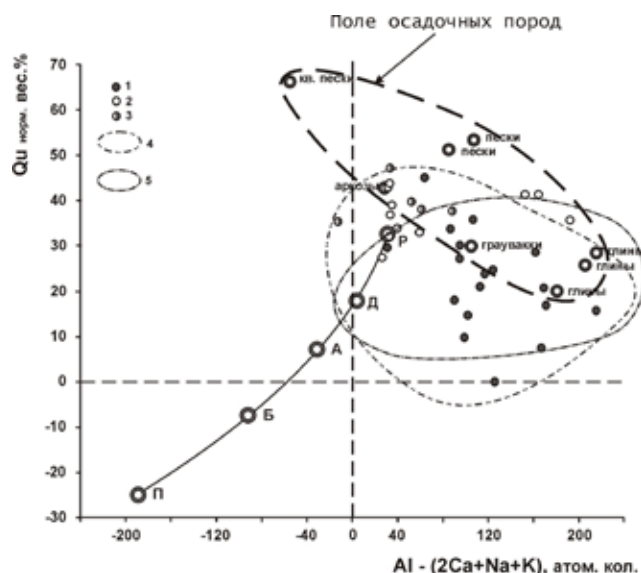
Рис. 5. Положение гнейсов кольской серии района Пулозеро – Полнек-Тундры на диаграмме Qm vs [Al - (2Ca+Na+K)] [2]. Средние типы: П – пикриты, Б – базальты, А – андезиты, Д – дациты, Р – риолиты (Соловьёв, 1970); пески, аркозы, граувакки и глины (Ронов, и др., 1963; 1970). 1 – умереннокальциевые гнейсы; высококальциевые гнейсы: 2 – гранат-биотитовые, 3 – биотитовые; поля архейских супракrustальных пород: 4 – кольский комплекс Терского, Титовского и Аннамско-Хихнаярвинского блоков [7], 5 – кольский комплекс Центрально-Кольского блока [1].
