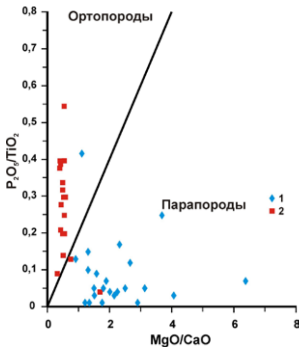
Рис. 2. Диаграмма P_2O_5/TiO_2 – MgO/CaO для гнейсов кольской серии [16]. 1 – умереннокальциевые гнейсы; 2 – высококальциевые гнейсы.
