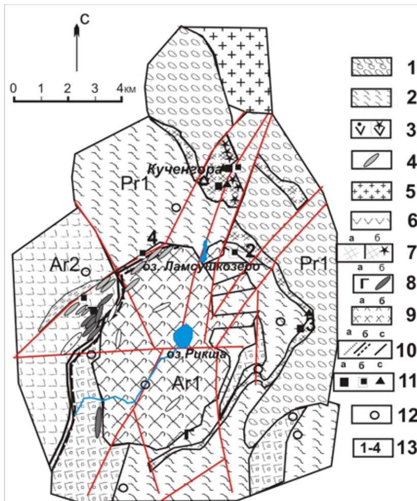
Рис. 2. Схема строения Рикшанской кольцевой структуры [7].
