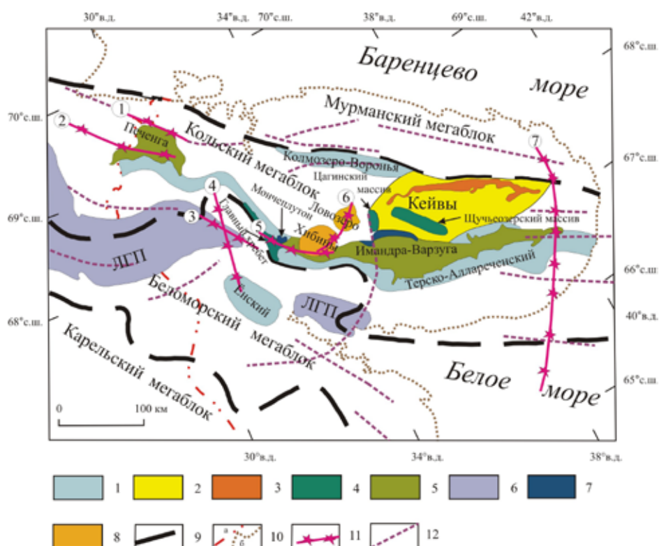
Рис. 4. Ослабленные зоны в фундаменте Кольского региона в архее, 2.6-2.5 млрд. лет назад. Условные обозначения см. на рис. 2. Цифры на карте: (а) раннепротерозойские магмапроводящие зоны, по геологическим данным и подтвержденные тектонофизическим моделированием: 1 – г. Генеральская, 2 – Порьиташская, 3 – Сальнотундровская-1, 4 – Сальнотундровская-2, 5 – Мончетундровская; (б) ослабленные зоны в фундаменте, активизировавшиеся в палеозое: 6 – Хибинская; (в) 7 – Восточно-Кольская (возраст и генезис не известны).
