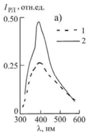
Рис. 3. Спектры РЛ исходных фторосульфатоцирконатных соединений (1) и после их быстрого нагрева (2): а – \text{Cs}_2\text{ZrF}_4\text{SO}_4 ; б – \text{Rb}_3\text{Zr}_2\text{F}_9\text{SO}_4 \cdot 2\text{H}_2\text{O} .
