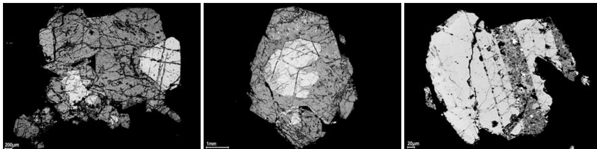
Рис. 5. Характер срастаний «шоколадного» и «кремового» циркона. РЭМ, BSE-изображения. На всех снимках «шоколадный» циркон – светло-серый, «кремовый» – тёмно-серый, сильно неоднородный. а – ксеноморфная кайма «кремового» циркона, обрастающая реликт неправильной формы (слева) и дипирамидальный кристалл (справа) «шоколадного» циркона. б – сrostок дипирамидальных кристаллов «шоколадного» в кайме «кремового». в – линейные зоны «кремового» циркона, «сшивающие» обломки «шоколадного». На рис. 5 в видно проникновение «кремового» циркона в узкие трещины «шоколадного».
