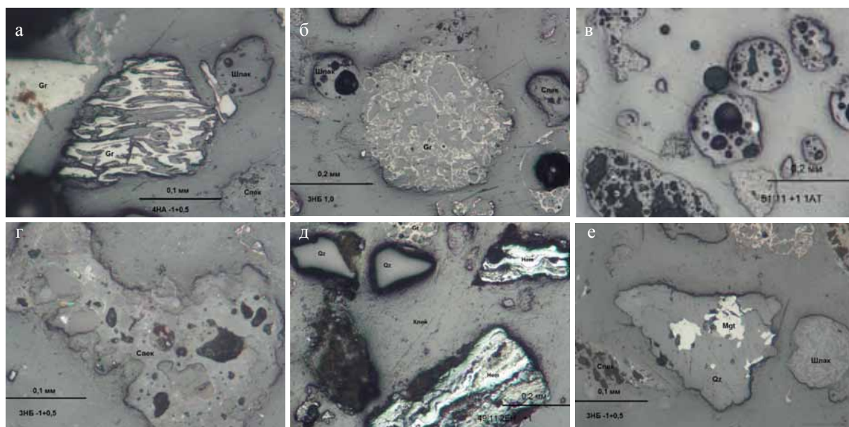
Рис. 1. Основные минералогические фазы золоотходов: а – частица сплошного графита с грубой слоистостью; б – частица пористого графита со сложным кружевоподобным строением; в – шарообразные образования шлака с включениями сульфидных и оксидных фаз (светлое); г – спёк из шлака, обломков силикатных частиц и оксидов железа; д – неоднородные пористые частицы гематита; е – обломок кварца с включениями магнетита.
