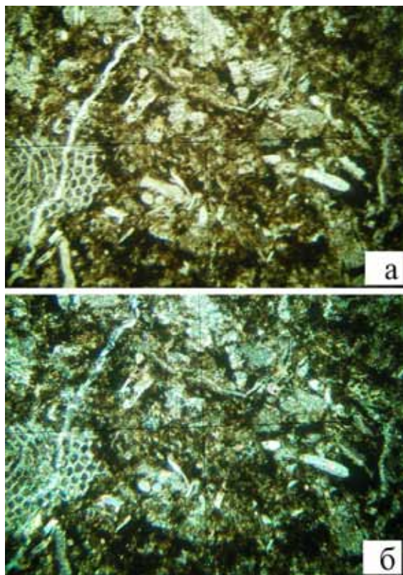
Рис. 3. Участки скрытокристаллического бёмита и органического вещества (тёмное) в био-литокластическом пакстоуне. Справа в нижней части виден фрагмент рецептакулита, шахта Новокальинского месторождения, горизонт 800 м, шлиф 07-8, а – естественный свет, б – поляризованный свет, увеличение \times 140 .
