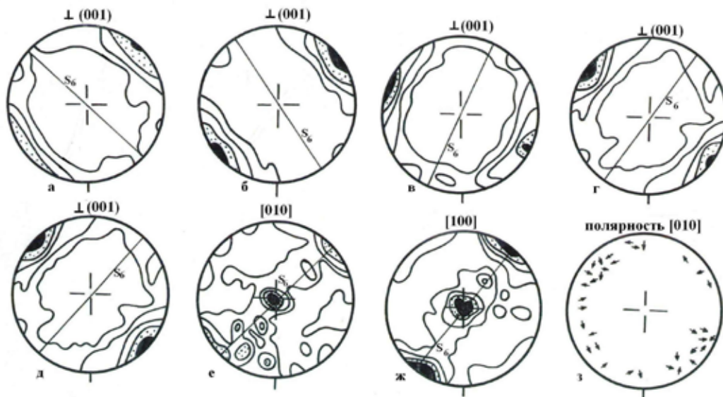
Рис. 3. Микроструктурные ориентировки биотита. а – гнейс \gamma_1 (изолинии 0.05-5-10-25 %, n=100 ); б – гранит \gamma_8 (изолинии 0.5-5-10-17 %, n=100 ); в – гнейс \gamma_1 (изолинии 0.4-2.3-6.9-11.5-13. %, n=214 ); г – гранодиорит \gamma_3 (изолинии 5-10-25 %, n=100 ); д – гнейсов \gamma_1 : д – изолинии 0.5-5-10-25 %, n = 100 ; е – изолинии 0.5-2.5-3.5-12 %, n = 100 ; ж – изолинии 0.5-2.5-3.5-12 %, z = 104 ; г – диаграмма полярности [010] = Nm; S_6 – сланцеватость этапа D_6 . В центр диаграммы проецируется линейность L_6 .
