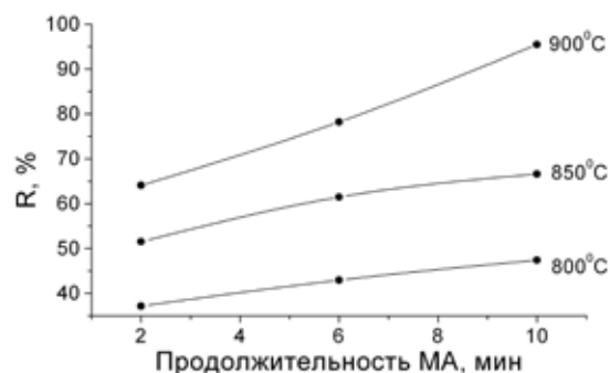
Рис. 6. Зависимость степени трансформации бадделеита в цирконат кальция при прокаливании смесей бадделеита и кальцита при 800, 850 и 900 °C в течение 5 час. в зависимости от продолжительности предварительной МА.
