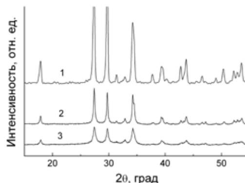
Рис. 2. Дифрактограммы титанита: 1 – исходный, 2 – после мокрой МА в течение 10 мин., 3 – после сухой МА в течение 10 мин.
