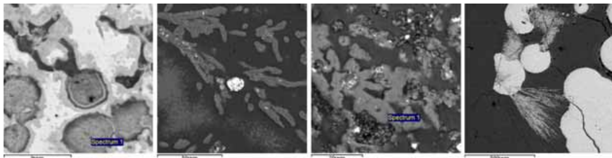
9. Минеральное срастание (сп. 1 – «серая почка» Fe-Cu-Se-Pb-U соединение, Y до 2.5-3 %). СВ-7а-12. 10. Веточки – V-Cr-Fe гидроксиды. Округлое белое стяжение Au Pd(Sb,As)-фаза. СВ-9-1. 11. То же. СВ-9-4-1 12. Гематит, гётит («шарики и снопики»). СВ-7-12.
