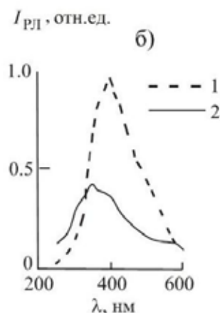
Рис. 3. Спектры РЛ исходных фторосульфатоцирконатных соединений (1) и после их быстрого нагрева (2): а – \text{Cs}_2\text{ZrF}_4\text{SO}_4 ; б – \text{Rb}_3\text{Zr}_2\text{F}_9\text{SO}_4 \cdot 2\text{H}_2\text{O} .
