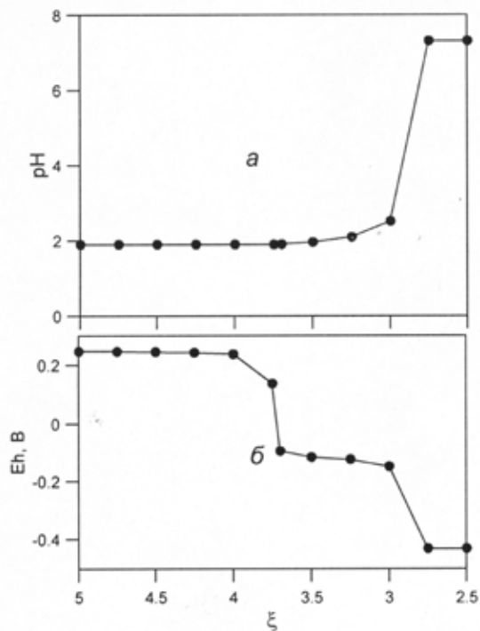
Рис. 1. Изменение pH (а) и Eh (б) закрытой к атмосфере системы Fe – \text{CuSO}_4 в зависимости от \xi .
