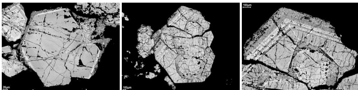
Рис. 6. Характер срастаний «жёлтого» циркона с «кремовым» и «розовым». РЭМ, BSE-изображения. Зоны разных типов циркона: ж – жёлтый, к – кремовый, р – розовый.
