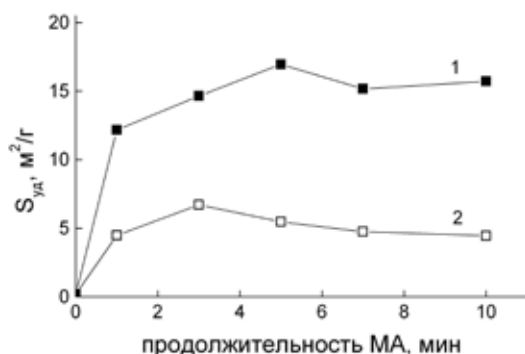
Рис. 1. Зависимость удельной поверхности титанита от продолжительности МА в планетарной мельнице: 1 – мокрая МА, 2 – сухая МА.
