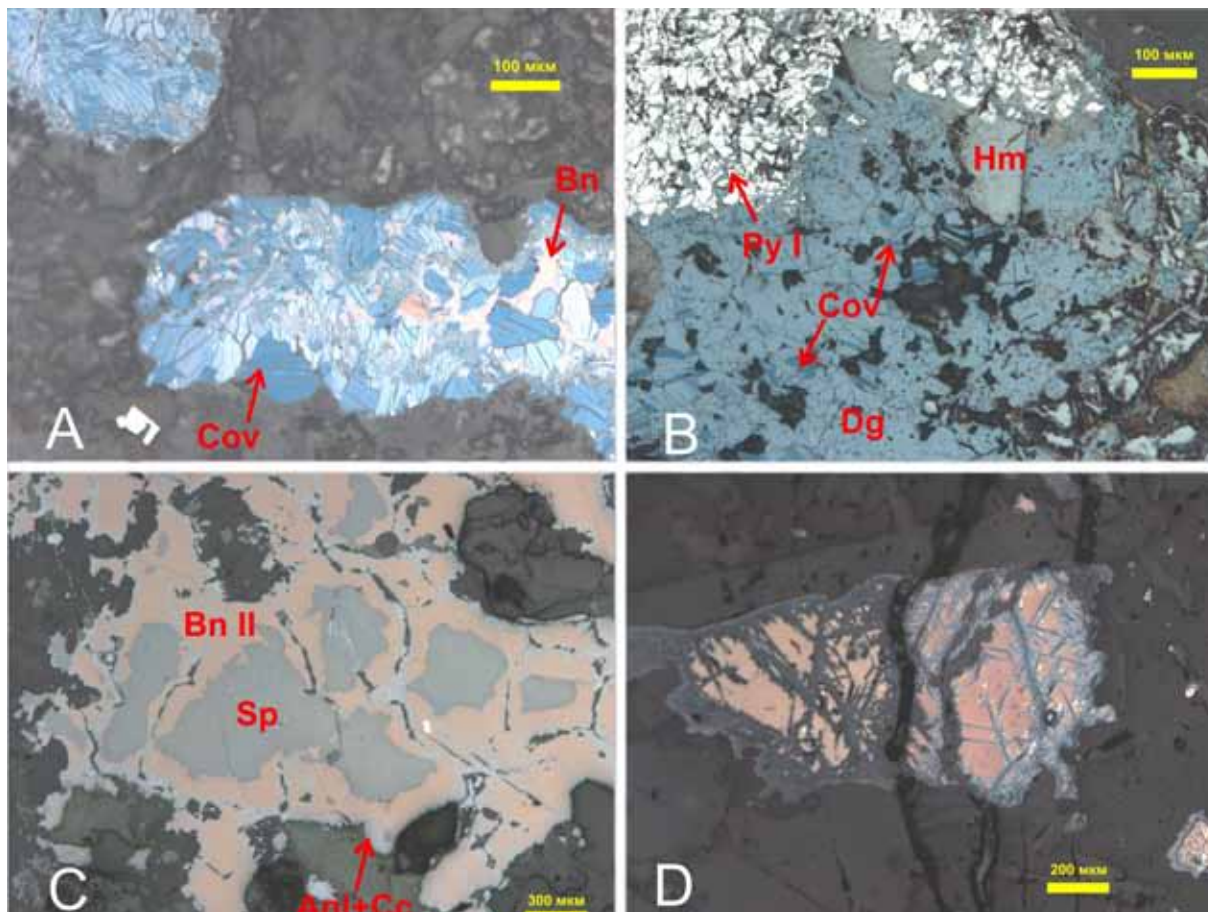
Рис. 5. Характер выделений борнита и минералов группы ковеллина.
