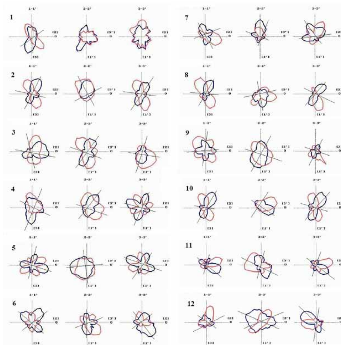
Рис. 1. Акустополяриграммы образцов. Синяя линия – положение ВП, красная – ВС. Цифры слева – номера образцов; в квадратных скобках – ориентировки граней; 1-1', 2-2', 3-3' – направления прозвучивания образцов кубической формы. Прямые скрещенные линии – проекции элементов упругой симметрии на грани.
