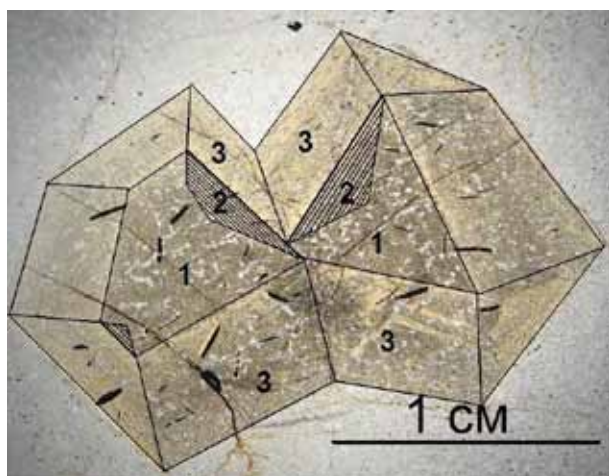
Рис. 1. Структура зональности в сростке кристаллов ставролита: 1 – ядро, 2 – вторая зона (ретуширована), 3 – третья зона. Фото шлифа. Чёрное – включения ильменита.
