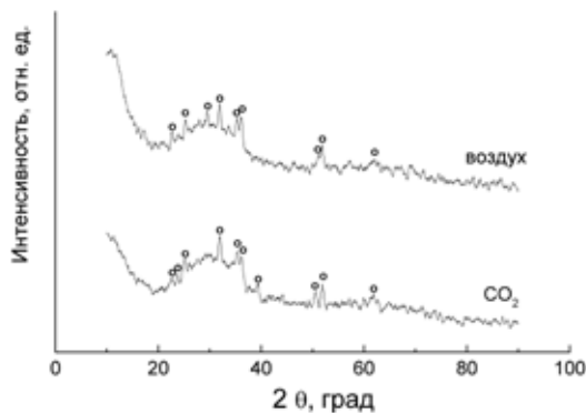
Рис. 1. Рентгенограммы шлака после МА воздушной среде и в \text{CO}_2 (о – рефлексы оливина).
