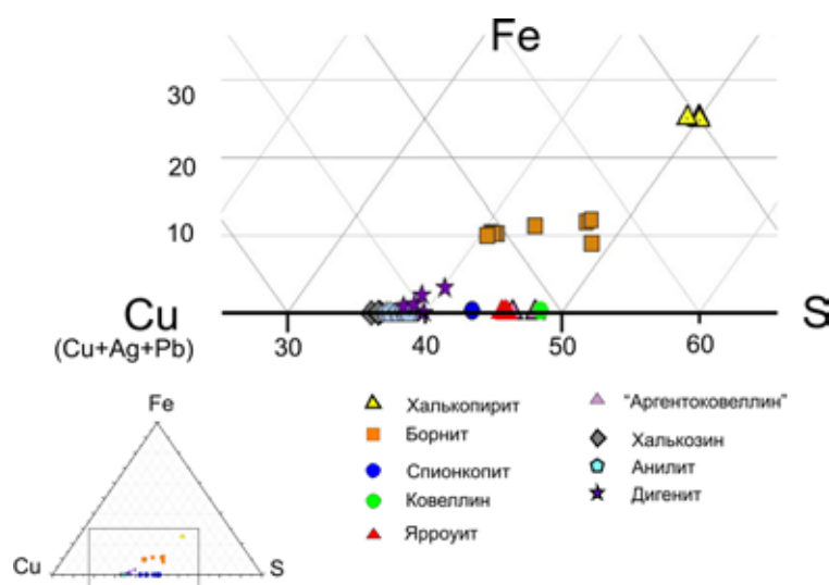
Рис. 3. Фрагмент тройной диаграммы составов минералов системы Cu-Fe-S.
