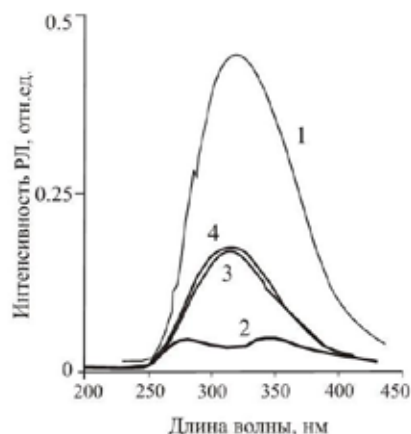
Рис. 4. 1 – \text{Rb}_3\text{H}_3\text{Zr}_3\text{F}_3(\text{PO}_4)_5 , 2 – \text{ZrF}_4 \cdot \text{Rb}(\text{PO}_4)_{0.33} \cdot \text{RbNO}_3 , 3 – \text{Rb}_2\text{Zr}_3\text{OF}_6(\text{PO}_4)_2 \cdot 2\text{H}_2\text{O} , 4 – \text{RbZrF}_2\text{PO}_4 \cdot 0.5\text{H}_2\text{O} .
