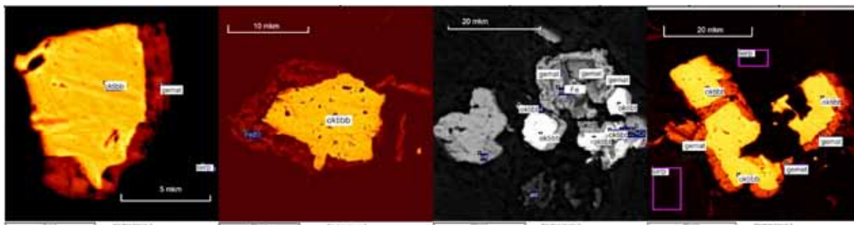
Рис. 3. Участок Оловозеро. Скв. 3, гл. 36.2 м. Составы и строение октибеггита (аваруита) – гематита в нём.
