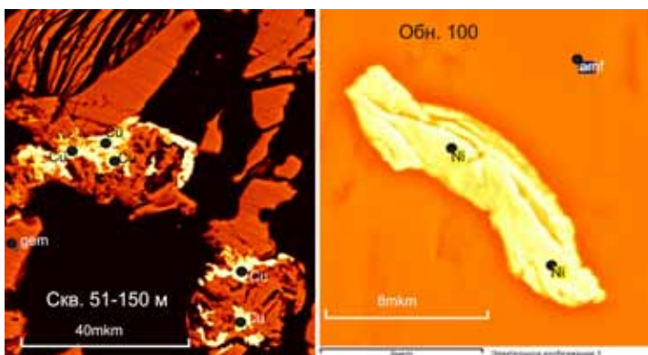
Рис. 6. Участок Выжига (рис. 1, т. 7). Скв. 51, гл. 150 м. Самородная медь и самородный никель.
