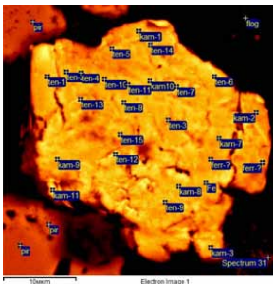
Рис. 8. Плессит (скв. 132, гл. 149). Видно тонкое прорастание камасита и тэнита с характерной системой пересекающихся деформированных полос – видманштеттовых фигур, характерных для железных метеоритов из группы октаэдритов.
