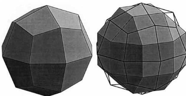
Рис. 8. Тетрагонтриоктаэдр дуален комбинации куба, октаэдра и ромбододекаэдра.
