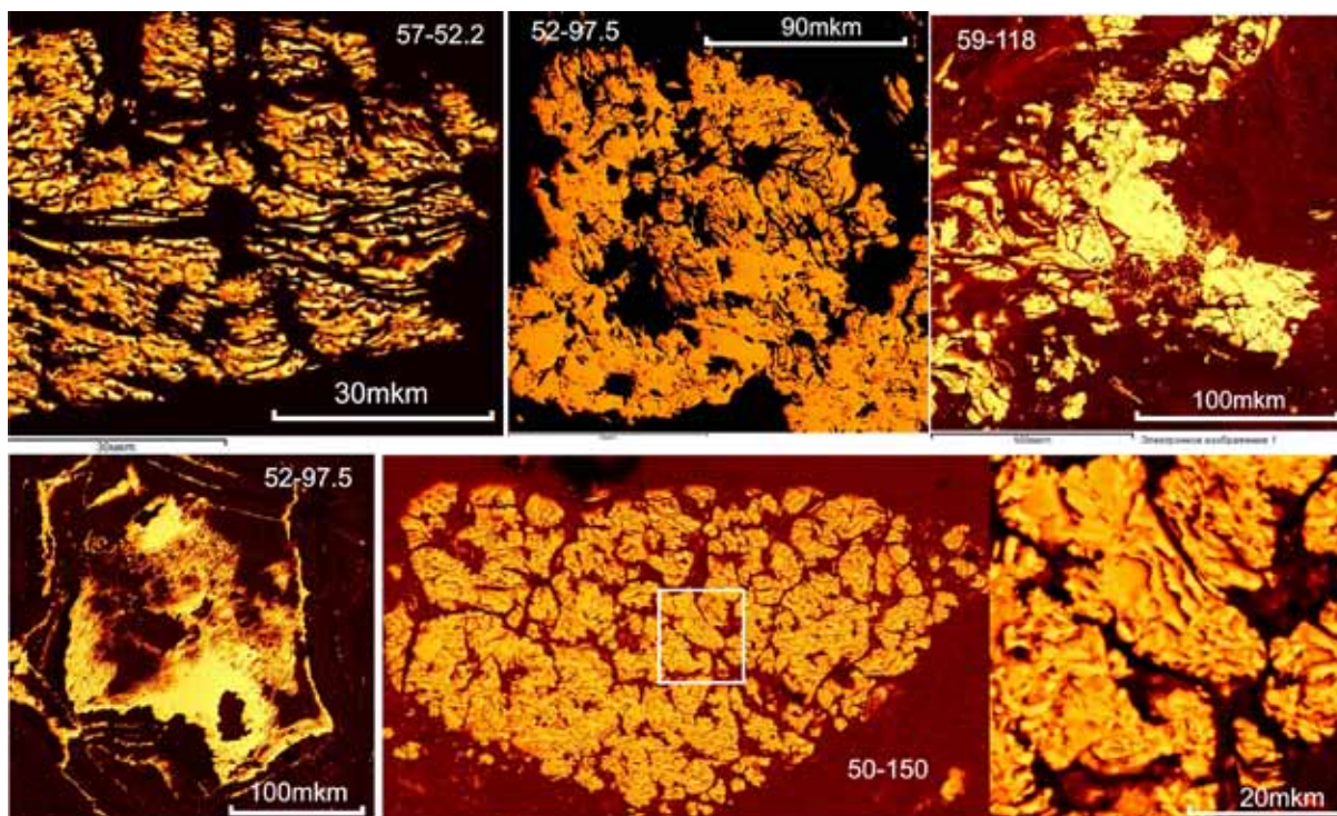
Рис. 4. Участок Выжига (рис. 1, т. 7). Скв. 51, гл. 150 м. Структура гематита «железная роза».
