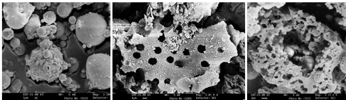
Рис. 2. Микрофотографии частиц золоотходов: слева – Апатитской ТЭЦ (АТ); в центре – пос. Ёнского (ЁН); справа – г. Новосибирска (НБ).
