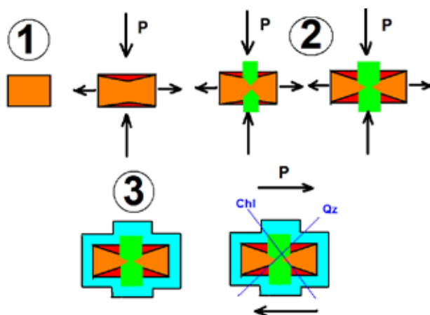
Рис. 8. Схема образования двойников ставролита (пояснения в тексте).
