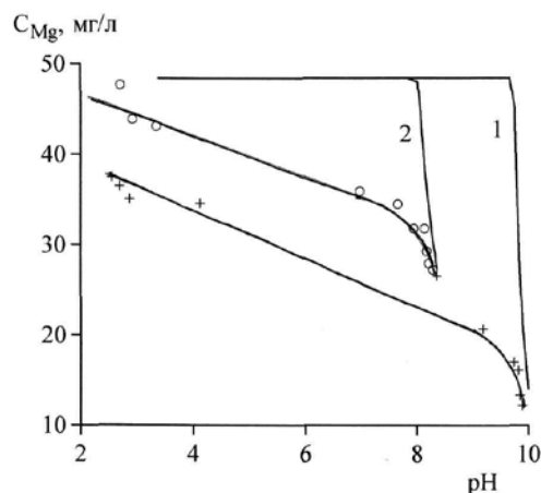
Рис. 2. Зависимость концентрации Mg от pH суспензии; расчётные данные для брусита (1) и клиноэнстатита (2); экспериментальные данные, продолжительность взаимодействия в течение 24 час. (+) и 30 сут. (o).
