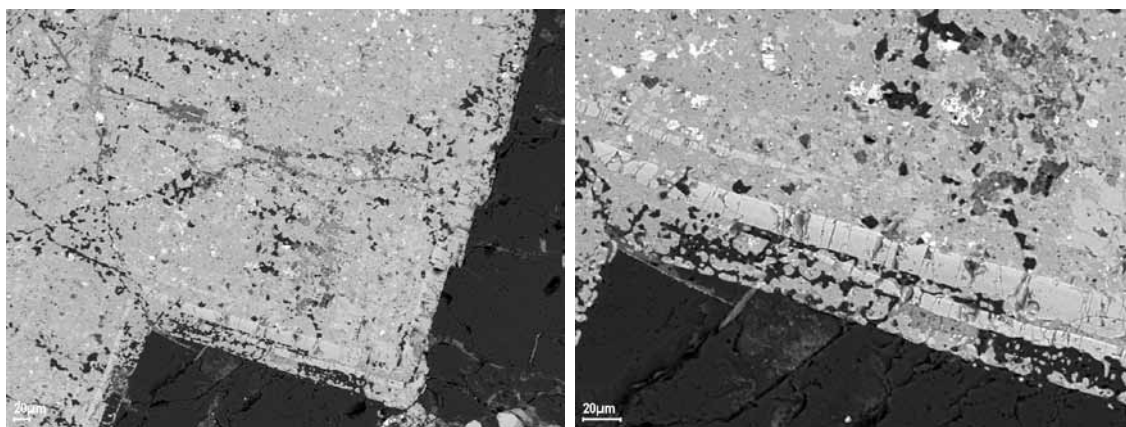
Рис. 1. Совместный (эвтектический) рост краевых зон «кремового» циркона и кварца. Глобулярная морфология сростков (б). РЭМ, BSE-изображение.
