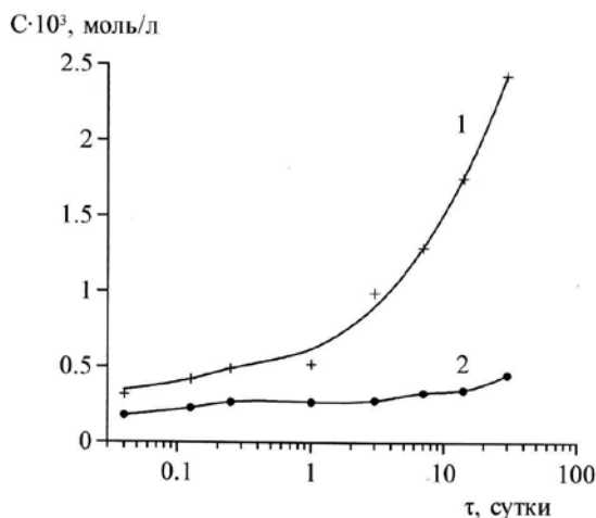
Рис. 3. Кинетические кривые растворения компонентов метасерпентина MgO (1) и SiO 2 (2).
