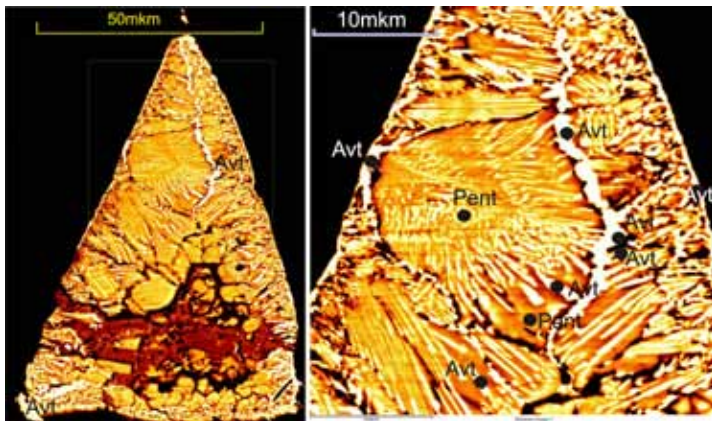
Рис. 5. Октиббегит или аварунит из скв. 51, гл. 150 м. Эмульсионная структура распада твёрдых растворов аварунита (октиббегита) в пентландите (решётчатая, звёздчатая, графическая, пламенивидная и пр.).
