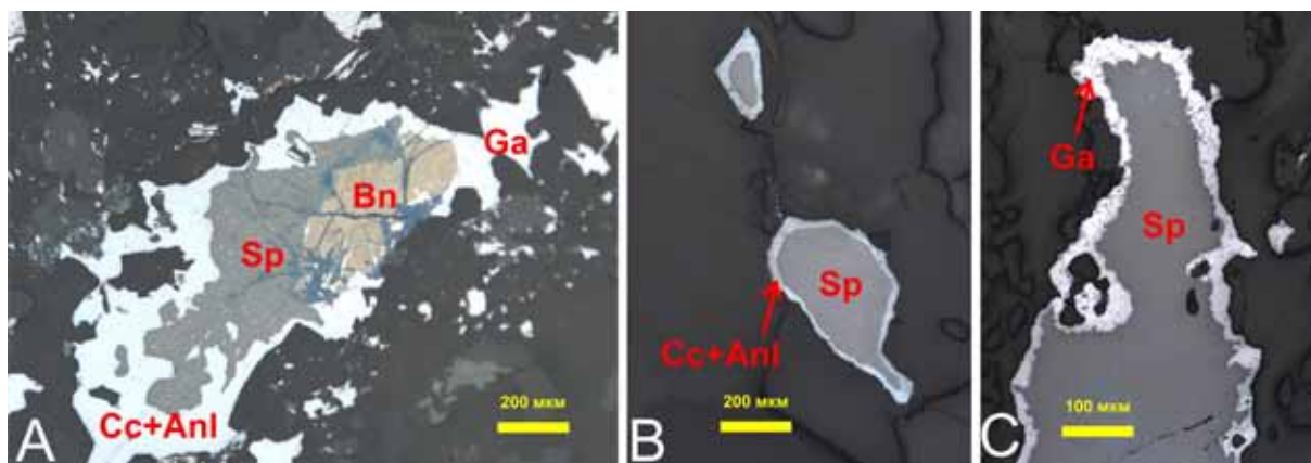
Рис. 7. Взаимоотношения сульфидных минералов в кварц-карбонатных жилах.
