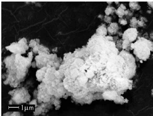
Рис. 4. СЭМ-изображение смеси бадделеита и кальцита после двухминутной МА в планетарной мельнице.
