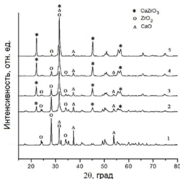
Рис. 7. Рентгенограммы обработанной в течение 8 часов в шаровой мельнице смеси бадделеита и кальцита, прокаленной при 900 °С в течение 3 часов (1), и прокаленных при 900 °С в течение 1 часа смесей бадделеита и кальцита с применением предварительной МА в АГО-2 в течение: 2 – 2 мин., 3 – 6 мин., 4 – 10 мин. 5 – смесь бадделеита и кальцита после 10 мин. МА в АГО-2, прокаленная 3 часа при 900 °С.
