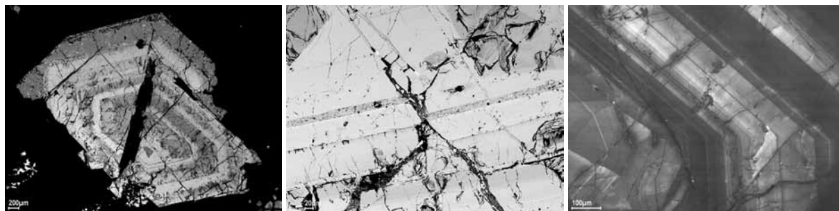
Рис. 2. Внутрифазовая неоднородность (зональность) «шоколадного» циркона. РЭМ, а, б – BSE-изображения, в – CL-изображение. (а) Первичная зональность представлена чередованием идиоморфных зон тёмно-шоколадного (светлые в BSE, слабо трещиноватые) и светло-шоколадного (более тёмные в BSE, с грубой поперечной трещиноватостью) циркона. В центре кристалла – крупный росток кварца. Вторичная зональность (обрастание «шоколадного» циркона «кремовым») представлена внешней зоной в верхней части кристалла («кремовый» циркон – самый тёмный в BSE, насыщенный включениями). (б) Смещение зон (нарушение рисунка зональности) вблизи трещины. (в) Первичная зональность более высокого порядка.
