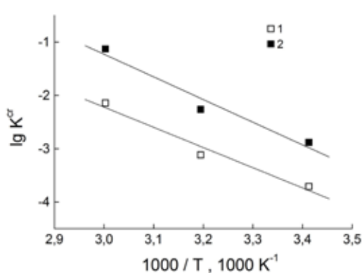
Рис. 10. Зависимость \lg k от обратной температуры: 1 – сухая МА, 2 – мокрая МА.
