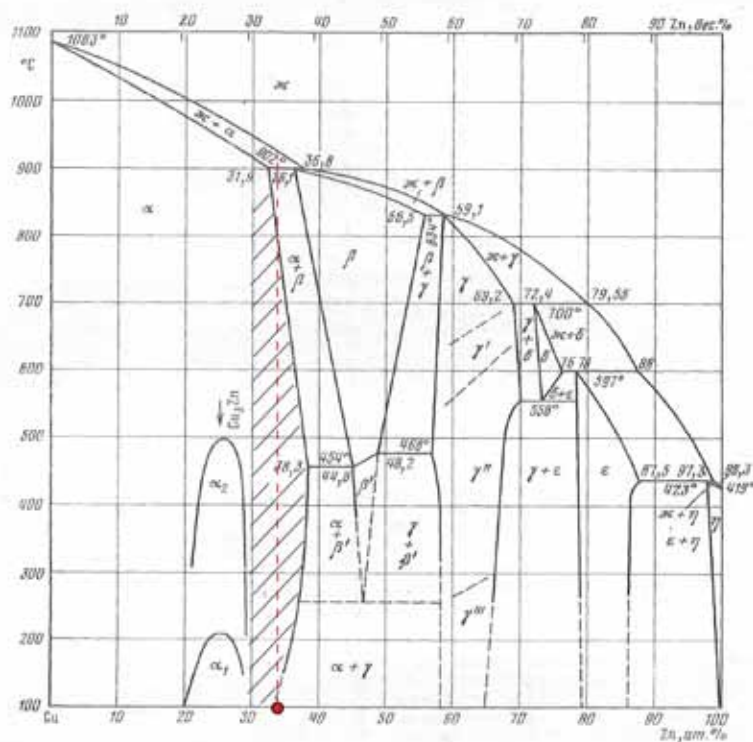
Рис. 6. Диаграмма состояния бинарной системы Cu-Zn.
