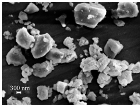
Рис. 4. СЭМ-изображение образца шлака после МА в \text{CO}_2 .
