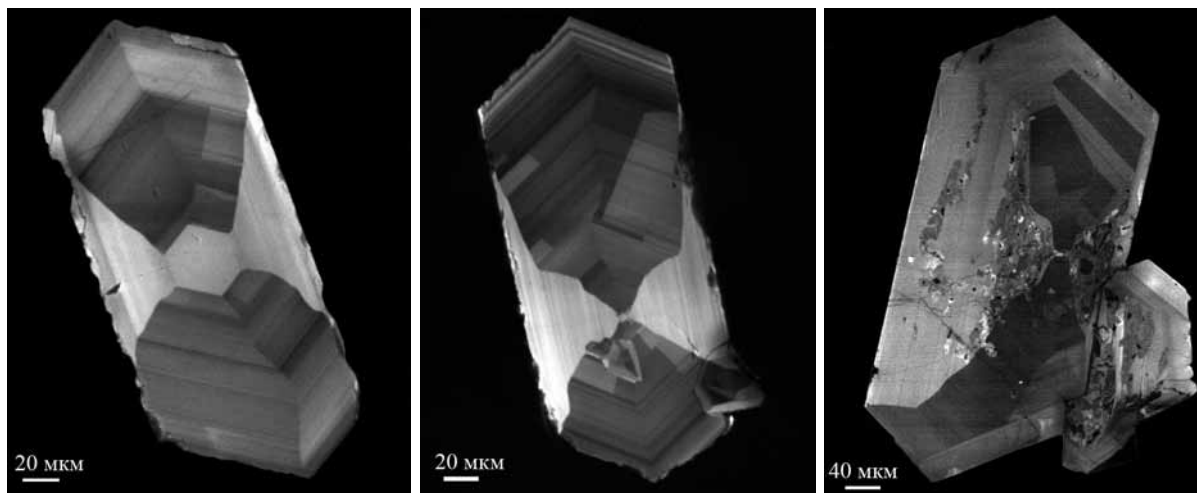
Рис. 3. Внутрифазовая неоднородность «жёлтого» типа циркона. РЭМ, CL-изображения.
