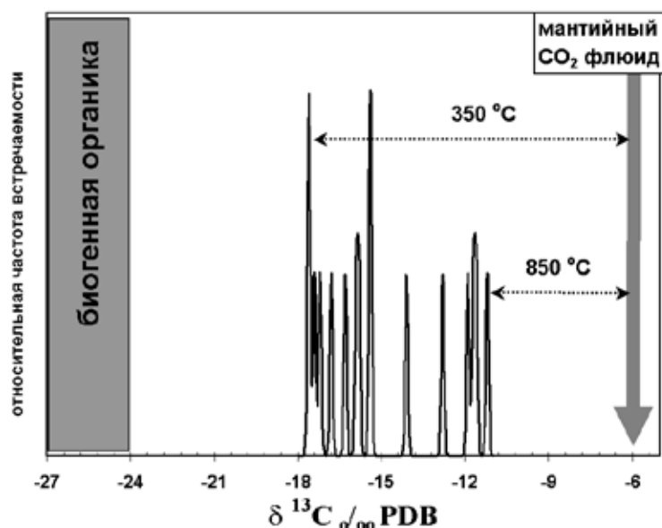
Рис. 2. Изотопный состав графита в кварцевых бластомилонитах о. Высокий. Стрелками показаны температуры равновесия изотопной системы углекислый газ-графит.
