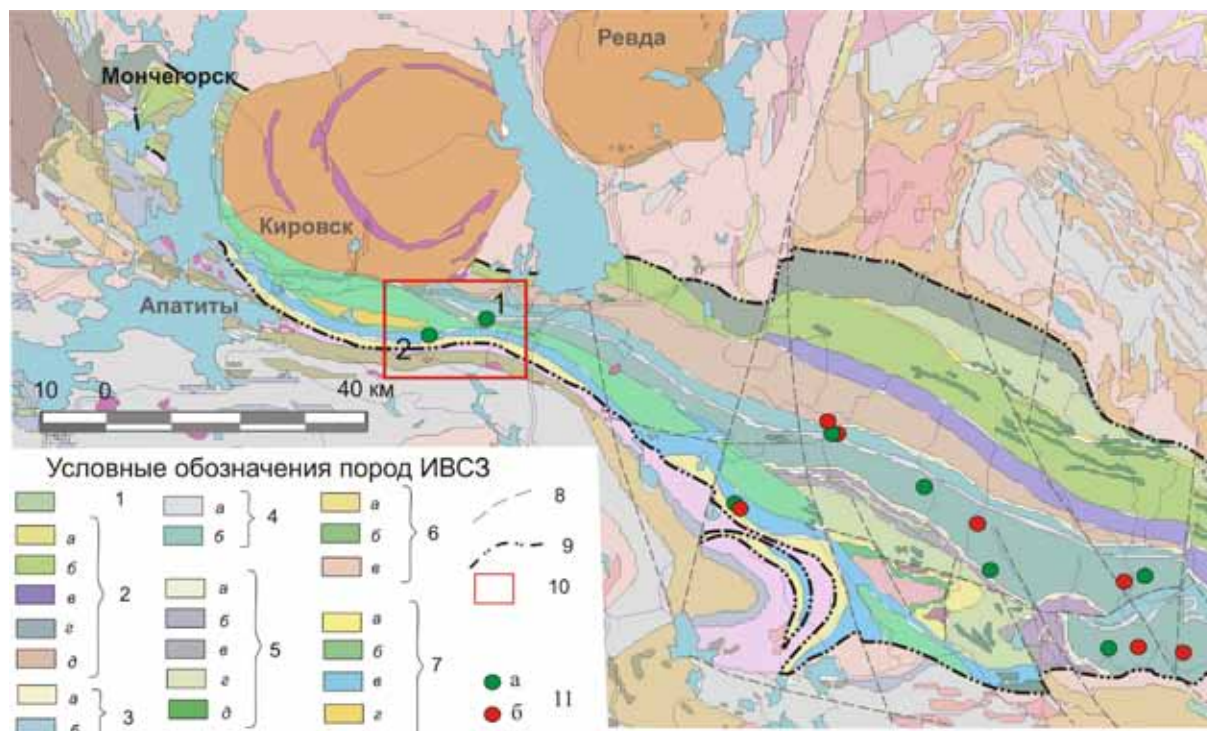
Рис.1 Схема геологического строения ИВСЗ с проявлениями медно-колчеданных руд.
