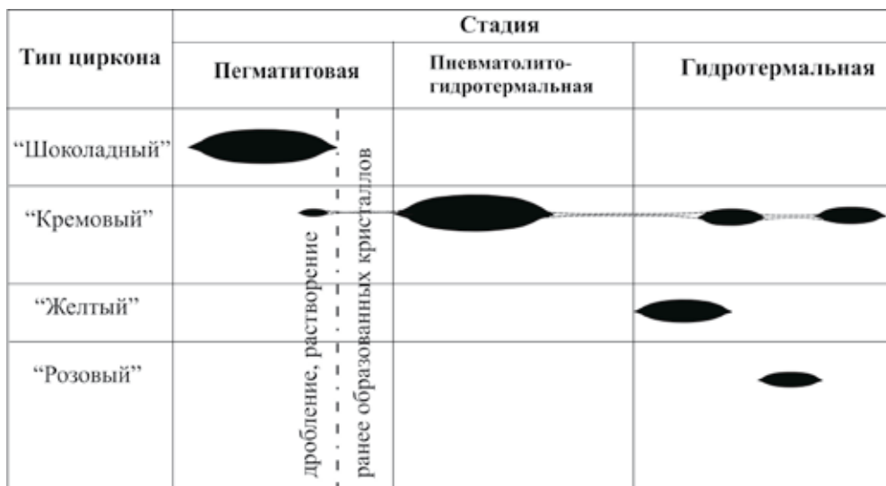
Рис. 10. Схема последовательности образования генераций циркона в пегматитовом теле «Цирконовое», массив щелочных гранитов Белых тундр, Кольский п-ов.
