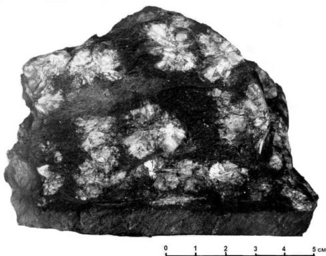
Рис. 5. Параморфическая руда.
