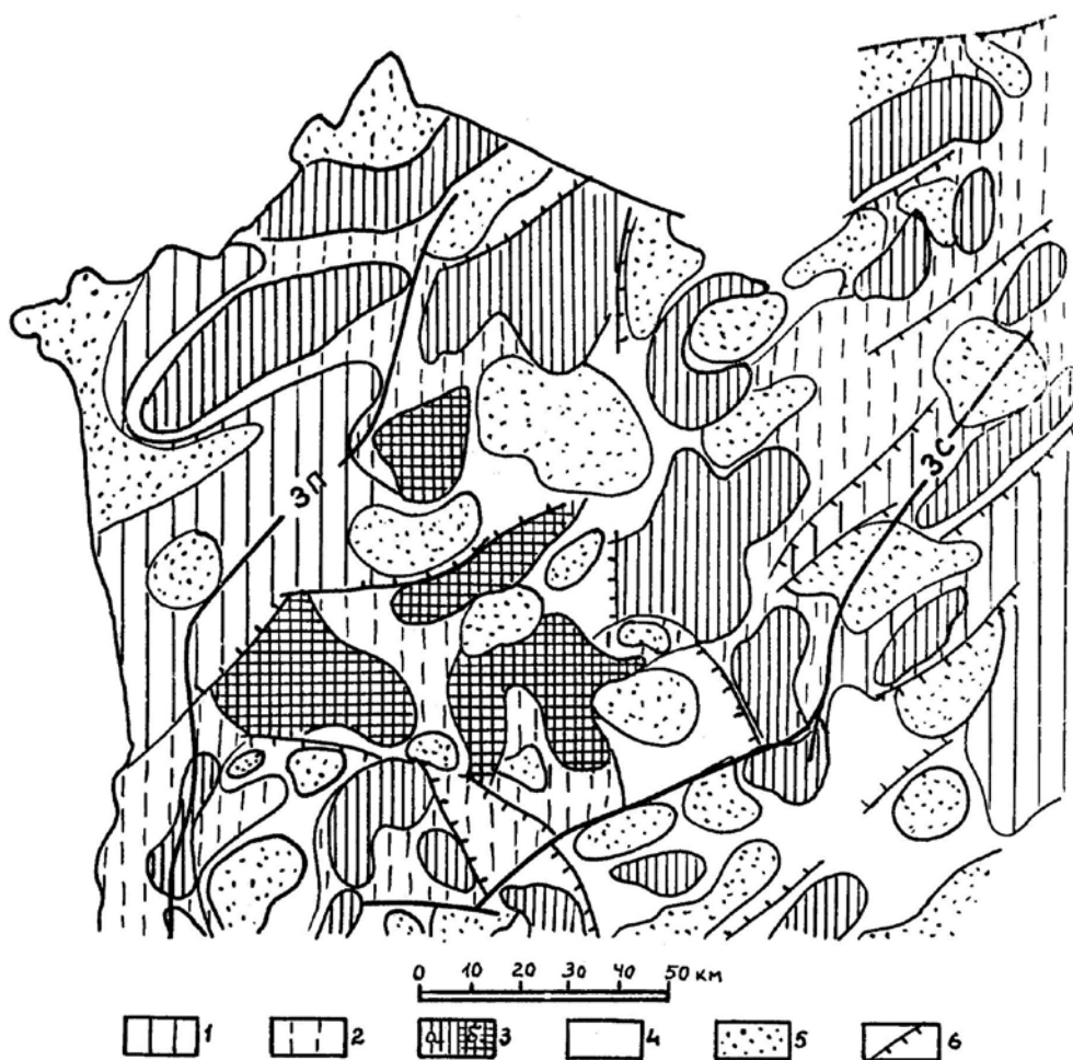
Рис. 17. Схема гравитационного поля юга Ханкайского массива (Р.Г. Кулинич, 1967).
