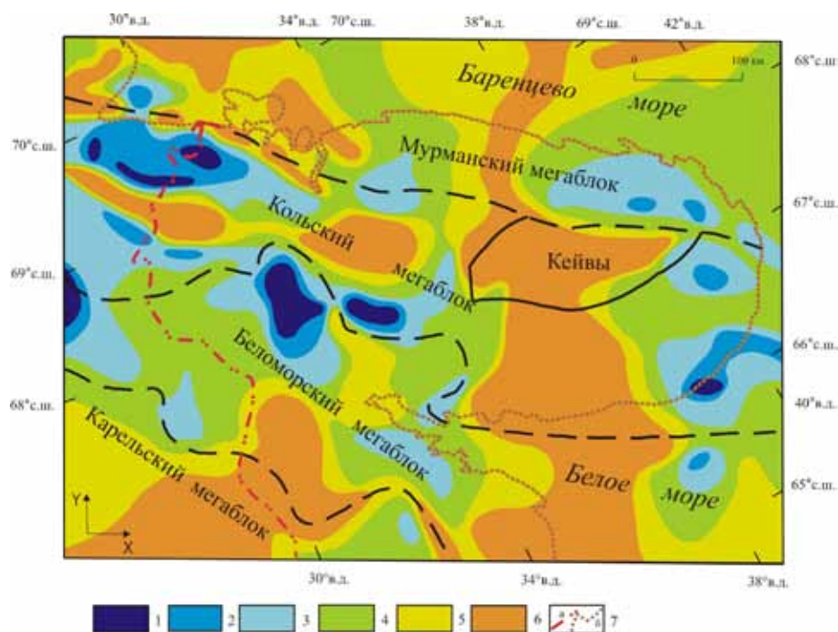
Рис. 3. Распределение градиентов напряжений для архея – 2.6-2.5 млрд. лет назад. Условные обозначения см. на рис. 1.
