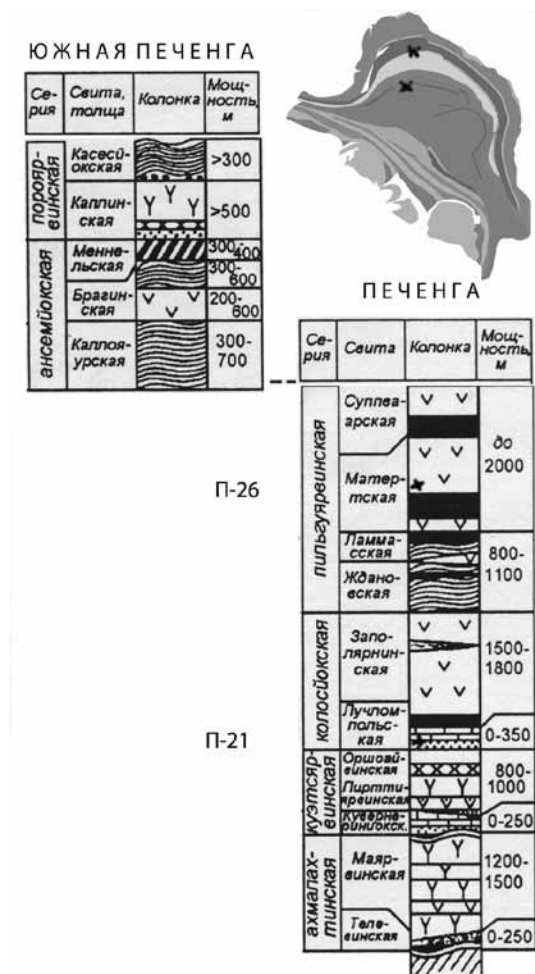
Рис. 1. Сводные стратиграфические колонки для Южно- и Северо-Печенгской зон по [9, 13] с указанием мест отбора проб на циркон.
