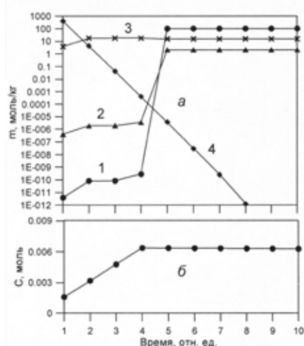
Рис. 6. Изменение состава раствора (а) и содержания меди (б) в системе Fe – CuSO 4 в зависимости от времени. а) Концентрации (m – моль/кг): 1 – Cu 2+ ; 2 – Cu + ; 3 – H + ; 4 – Fe 2+ .
