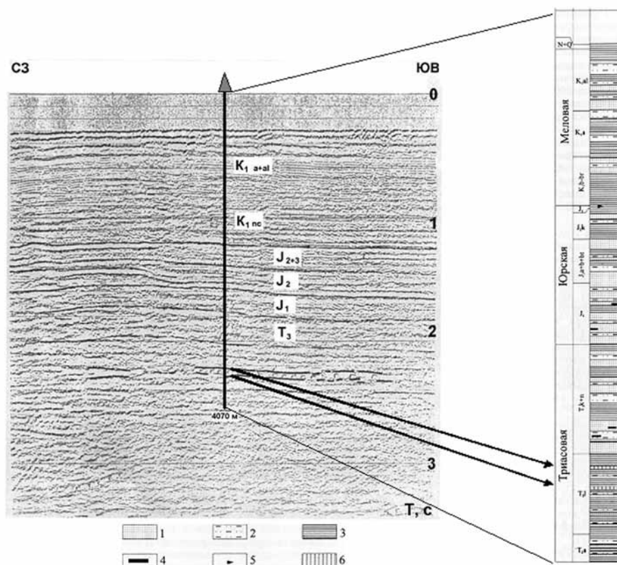
Рис. 3. Сопоставление сейсмического разреза (фрагмент профиля 088513) Лудловской площади и разреза скважины, вскрывшей пластовые тела силлов в терригенном разрезе триаса [15]. Стрелками показано положение силлов в разрезе скважины. Литологический состав: 1 – песчаники, 2 – алевролиты, 3 – глины, аргиллиты, 4 – угленосность, 5 – битуминозные аргиллиты, 6 – базальты.
