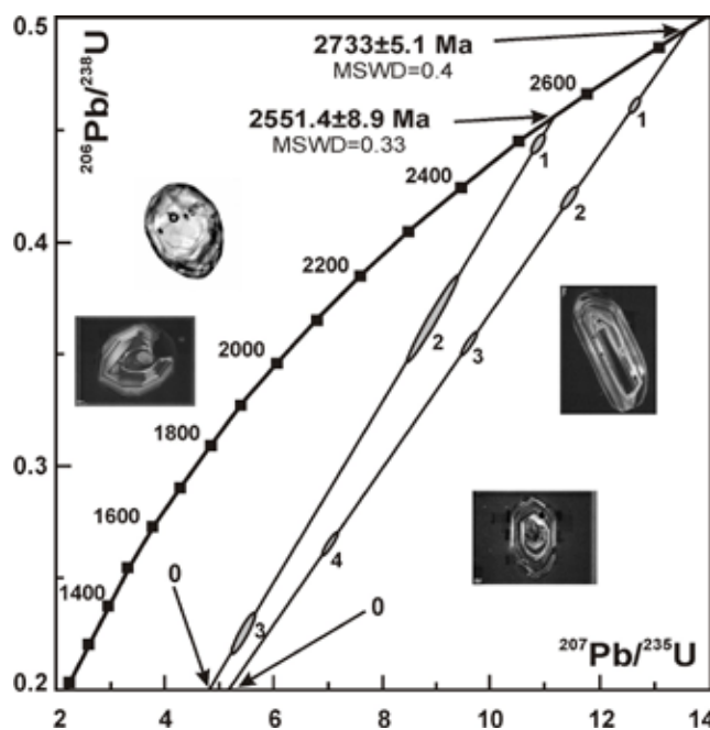
Рис. 8. U-Pb диаграмма с конкордией для цирконов из высококальциевых гнейсов кольской серии.
