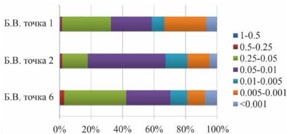
Рис. 2. Процентное содержание фракций в ДО исследованных озёр.
