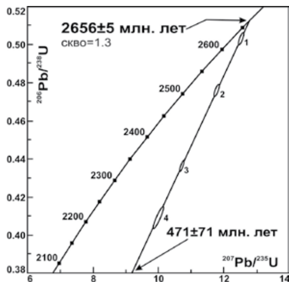
Рис. 8. U-Pb диаграмма с конкордией для циркона из пегматитового тела «Цирконовое», массив щелочных гранитов Белых тундр, Кольский п-ов.
