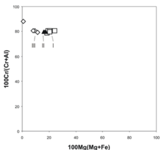
Рис. 3. Соотношение хромистости и магнезиальности хромшпинелидов: I – из коматиитов массива Кауниинлампи; II – из коматиитов массива Вара; III – из серпентинитов западной части пояса Иломантси [6,7]; IV – из коматиитов Кряжа Ветреный пояс [4].
