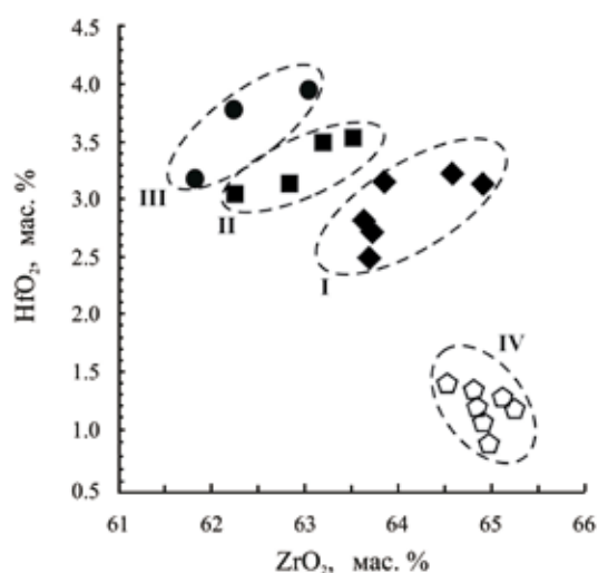
Рис. 7. Диаграмма ZrO_2 - HfO_2 для циркона из пегматитового тела «Цирконовое», Белые тундры, Кольский п-ов. Группы: I – «шоколадный», II – «жёлтый», III – «розовый» типы циркона. Группа IV магматического циркона из массивов Белые тундры и Западнокейвского показана по [2].
