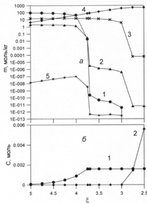
Рис. 2. Изменение состава раствора (а) и содержания твёрдых фаз (б) в закрытой к атмосфере системе Fe – \text{CuSO}_4 в зависимости от \xi . а) Концентрации: 1 – \text{Cu}^{2+} ; 2 – \text{Cu}^+ ; 3 – \text{H}^+ ; 4 – \text{Fe}^{2+} ; 5 – \text{Fe}^{3+} ; б) Содержания: 1 – Cu; 2 – \text{Fe}_3\text{O}_4 .
