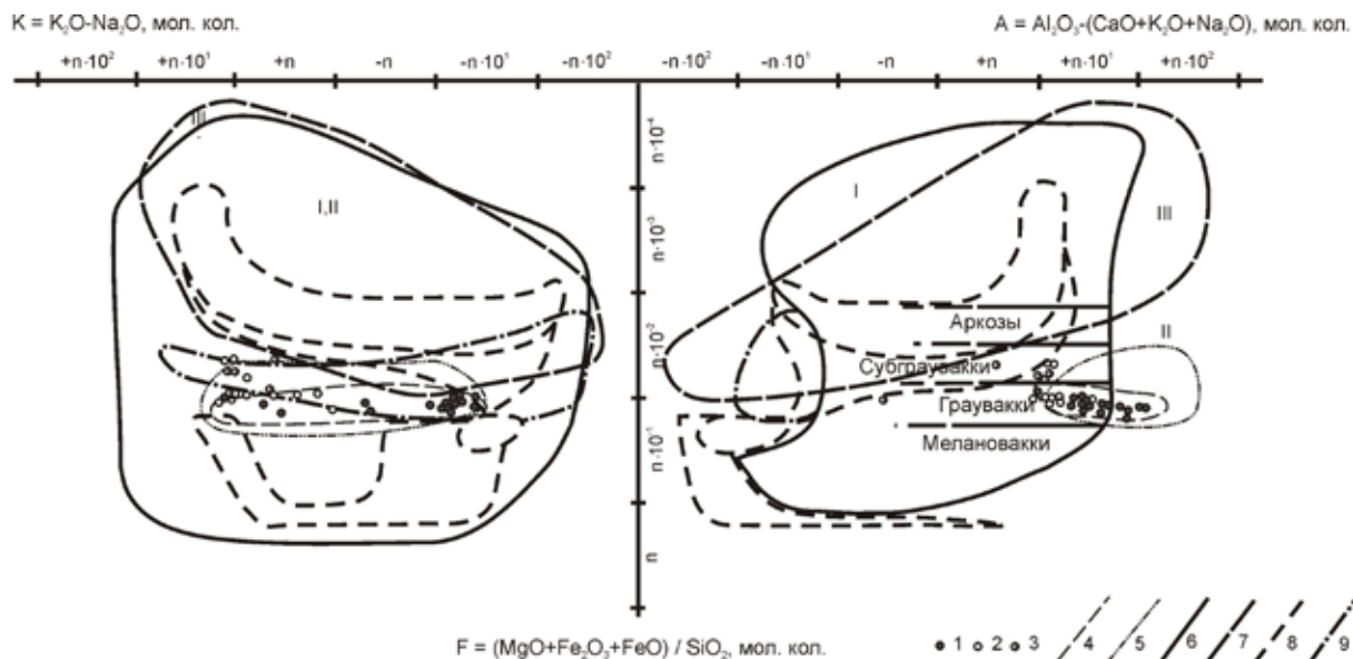
Рис. 3. Положение гнейсов кольской серии на диаграмме Предовского ФАК [10] для реконструкции исходного состава метаморфических пород.
