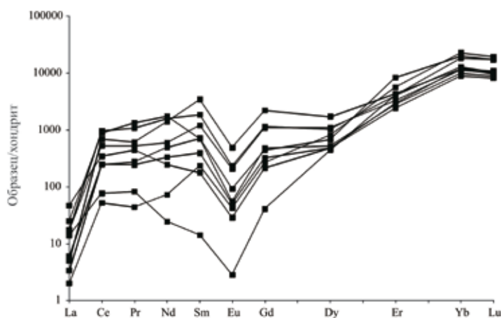
Рис. 9. Распределение редкоземельных элементов в «жёлтом» цирконе из пегматитового тела «Цирконовое», Белые тундры, Кольский п-ов.
