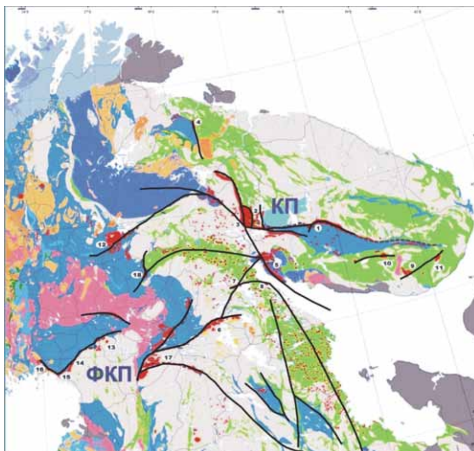
Рис. 1. Тренды рифтогенных поясов и известные раннепротерозойские базитовые комплексы северной половины ВСКБОИП (Митрофанов Ф.П., 2011). КП – Кольский пояс; ФКП – Фенно-Карельский пояс; номера расслоенных комплексов: 1 – Фёдорово-Панский; 2 – Мончеплутон; 3 – Мончетундровский, Волчетундровский массивы, Главный хребет; 4 – г. Генеральская; 5 – Кандалакшский и Колвицкий массивы; 6 – Луккулайсваара; 7 – Кондозёрский массив; 8 – Толстик; 9 – Ондомозёрский; 10 – Песчаноозёрский; 11 – Пялочный; 12 – Кейвица; 13 – Портимо (Контярви, Сиика-Кямя; Ахмаваара); 14 – Пеникат; 15 – Кеми; 16 – Торнио; 17 – Койллисмаа; 18 – Аканваара. В Беломорском домене много мелких будинированных тел.
