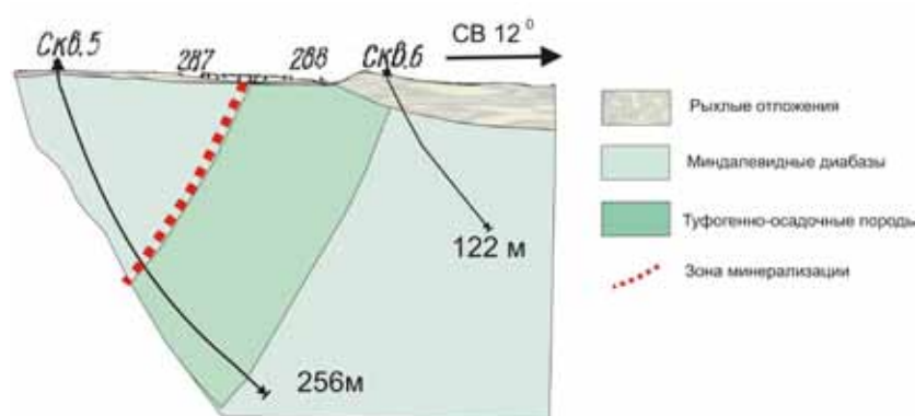
Рис.2. Схематический разрез по участку «33 км» по Зильбер [8] с упрощением.
