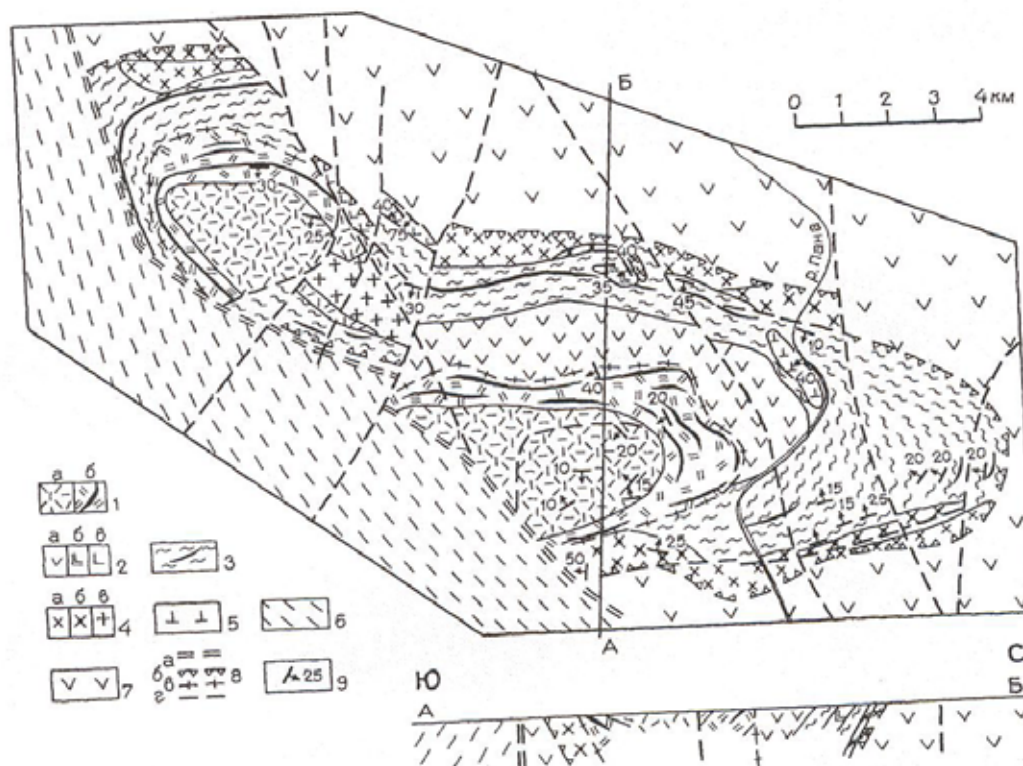
Рис. 2. Схематическая геологическая карта Панареченской вулcano-тектонической структуры (ПВТС).
