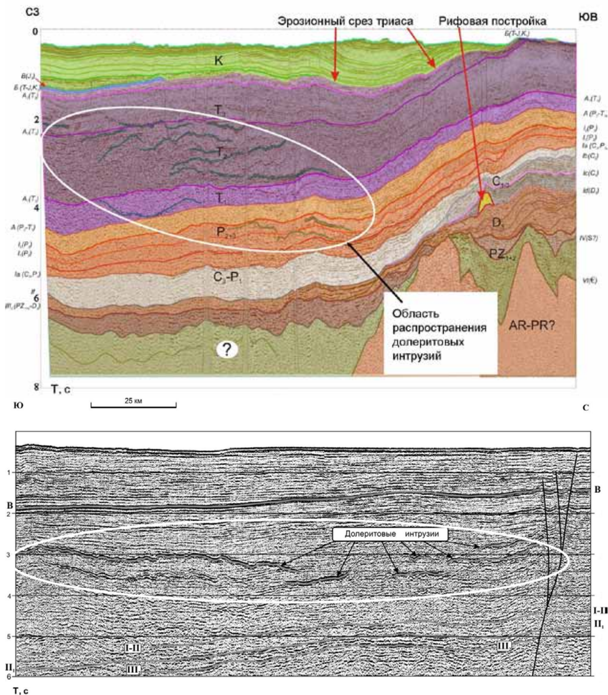
Рис. 2. Сейсмогеологические разрезы, иллюстрирующие распространение базальтоидных силлов в осадочном чехле впадин: сверху – Северо-Баренцевоморской (профиль 200705, по [9] с изменениями), внизу – Южно-Баренцевоморской (профиль 81108, по [22] с изменениями). По бокам разрезов – индексы отражающих сейсмических горизонтов и их стратиграфическая привязка (в скобках). Положение профилей на рис. 1.
