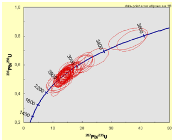
Рис. 5. Изохронная диаграмма с конкордией для циркона из пробы П-21.
