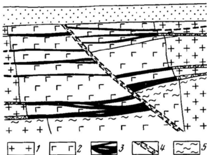
Рис. 8. Поперечный схематический разрез Диабазового месторождения (В.Н. Горбунов, 1972).
