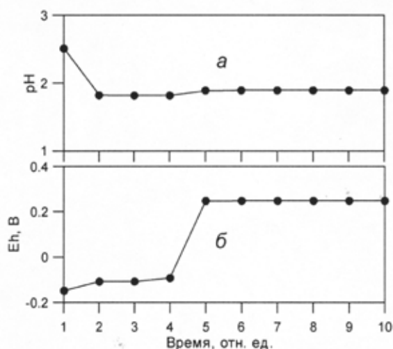
Рис. 5. Изменение pH (а) и Eh (б) системы Fe – CuSO 4 в динамическом режиме.
