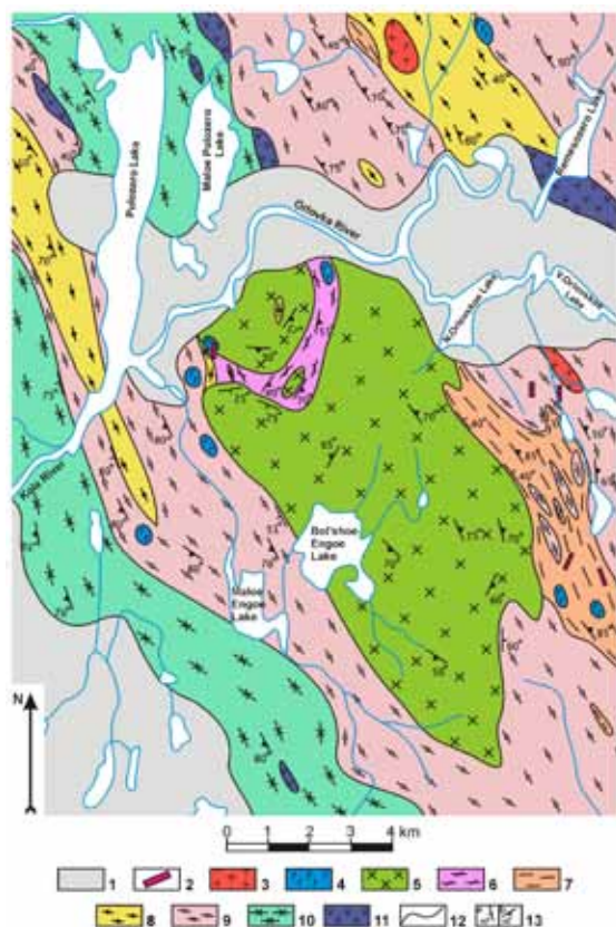
Рис.1. Обзорная геологическая карта района Пулозеро – Полнек-Тундра (по материалам С.А. Дюкова (1957); В.В. Балаганского, М.Н. Богдановой (1987) и личным наблюдениям Л.С. Петровской, М.Н. Петровского [9]). 1 – четвертичные отложения; 2 – пегматоидные жилы; 3 – плагиомикроклиновые граниты; 4 – метагаббро; 5 – эндербиты варьирующего состава от кварцевого диорита до плагиогранита; 6 – высококальциевые гранат-биотитовые и биотитовые гнейсы; 7 – двуслюдяные гнейсы; 8 – гранат-силлиманит-биотитовые гнейсы с подчиненными прослоями биотитовых и гранат-биотитовых гнейсов; 9 – гранат-биотитовые гнейсы с прослоями гранат-силлиманит-биотитовых и биотитовых гнейсов; 10 – пироксеновые и амфибол-пироксеновые гнейсо-диориты, диориты и частично гранодиориты; 11 – амфиболиты; 12 – геологические границы; 13 – элементы залегания: а) контактов, б) гнейсовидности.
