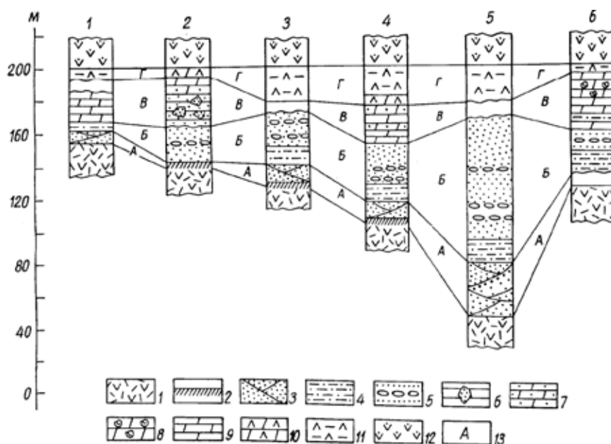
Рис. 2. Схематические стратиграфические колонки лучломпольской свиты Северо-Печенгской зоны по [7]: 1 – руч. Колос-йоки около пос. Никель; 2 – руч. Колос-йоки, 2.5 км от оз. Лучломполо; 3 – руч. Колос-йоки, 2 км от оз. Лучломполо; 4 – руч. Колос-йоки, 1.5 км от оз. Лучломполо; 5 – 0.5 км к востоку от оз. Лучломполо; 6 – оз. Иллепин-ярви. 1 – субщелочные вулканиты пирттиярвинской свиты; 2 – зона выветривания вулканитов; 3 – косослоистые красноцветные гематит-магнетитовые аркозовые метапсаммиты; 4 – тонкослоистые магнетит-гематитовые полевошпат-кварцевые и аркозовые пелитовые метаалевролиты; 5 – мелкогалечные аркозовые и полевошпат-кварцевые конгломераты, метагравелиты и метапсаммиты с гематитом; 6 – тонкослоистые магнетитовые полевошпат-кварцевые и граувакковые метапсаммиты с обломками аркозовых метаалевролитов; 7 – песчанистые доломиты; 8 – органогенные доломиты; 9 – доломиты; 10 – доломиты с туфогенным материалом; 11 – туффиты; 12 – базальтовые вулканиты запольяринской свиты; 13 – индекс пачек.
