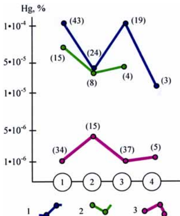
Рис. 3. Графики распределения ртути в основных типах магматических пород и апатитах Хибинского массива.
