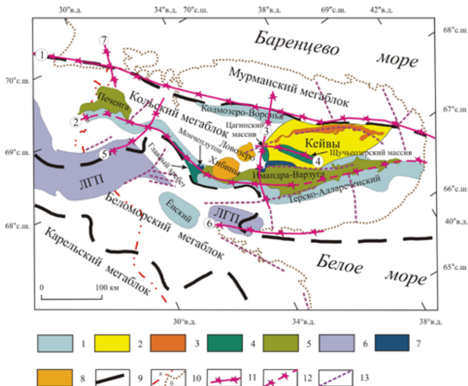
Рис. 2. Ослабленные зоны в фундаменте Кольского региона, сформировавшиеся в архее в интервале 2.9-2.6 млрд. лет назад. 1 – архейские пояса Колмозеро-Воронья, Терско-Аллареченский, Ёнский; 2 – высокоглинозёмистые гнейсы Кейвской серии (песчовотундровская толща); 3 – высокоглинозёмистые гнейсы Кейвской серии (песчовотундровская толща); 4 – массивы анортозитов и габбро-анортозитов (архей/ранний протерозой); 5 – Печенга-Имандра-Варзугская палеорифтогенная структура; 6 – Лапландский гранулитовый пояс; 7 – расслоенные массивы основных и ультраосновных пород (ранний протерозой); 8 – щелочные интрузивы (палеозой); 9 – разломы (зоны разломов) на контакте мегаблоков; 10 – а) государственная граница России, б) современная береговая линия; 11 – магмапроводящие зоны, установленные по аномальным значениям градиентов напряжений; 12 – магмапроводящие зоны, выделенные в поле градиентов средних значений по отдельным локальным аномалиям и совпадающие с областью развития пород Терско-Аллареченского пояса; 13 – ослабленные зоны в фундаменте, выделенные в поле градиентов напряжений со значениями ниже средних. Цифры в кружочках: (а) архейские магмапроводящие зоны, известные по геологическим данным и подтверждённые результатами тектонофизического моделирования: 1 – пояс Колмозеро-Воронья, 2 – Терско-Аллареченский пояс, 3 – Цагинская, 4 – Щучьёозёрская; (б) ослабленные зоны в фундаменте, активизировавшиеся в раннем протерозое: 5 – Туломская, 6 – Колвицкая, 7 – Лиинахамарская.
