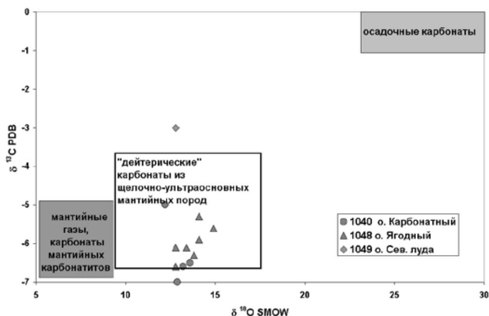
Рис. 1. Изотопный состав углерода и кислорода в карбонатах из карбонатных метасоматических пород Порей губы.
