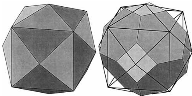
Рис. 10. Тетрагексаэдр дуален октаэдру, усечённому гранями куба.
