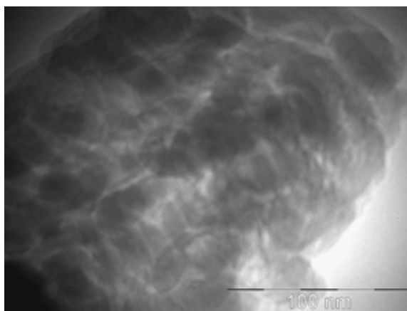
Рис. 7. ПЭМ-изображения образца геополимера на основе шлака, механоактивированного в \text{CO}_2 .
