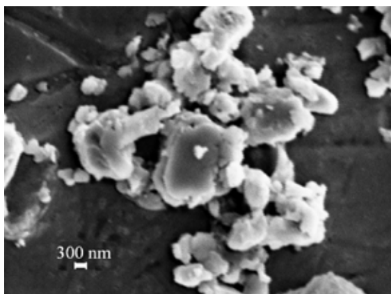
Рис. 3. СЭМ-изображение образца шлака после МА в воздушной среде.
