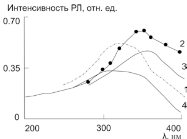
Рис. 1. Ультрафиолетовая часть спектра РЛ фторометаллатов: 1 – K_2ZrF_6 , 2 – Rb_2ZrF_6 , 3 – Cs_2ZrF_6 , 4 – K_2HfF_6 .
