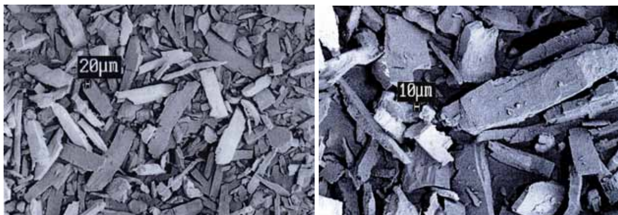
Рис. 3. Формы частиц кианита под электронным микроскопом (SEM LEO 420), напыление золотом.
