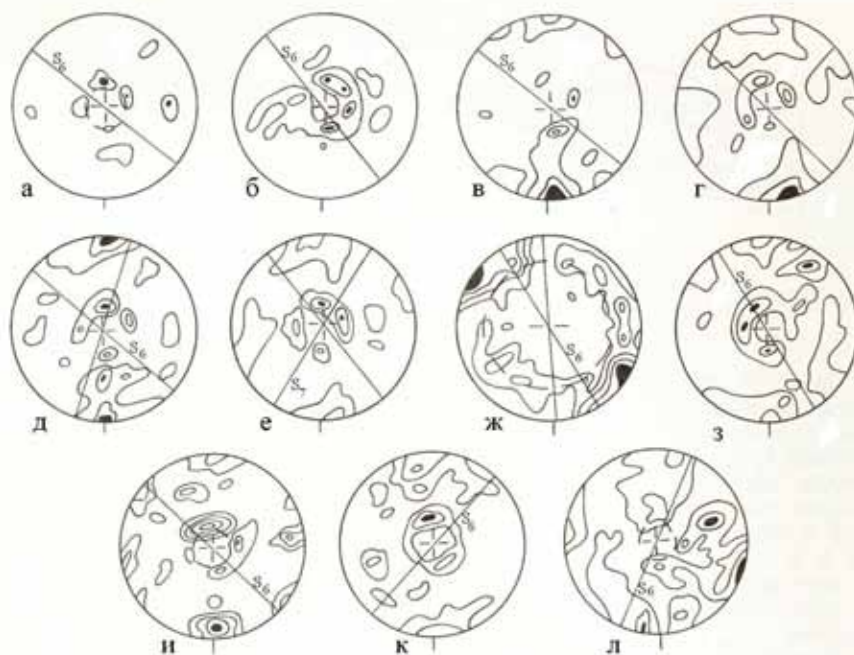
Рис. 1. Ориентировки осей [0001] кварца (здесь и ниже равноугольная проекция на верхнюю полусферу): а – гнейс \gamma_1 (изолинии 4.8-7.3 %, n = 41 ), б – гранит \gamma_8 (изолинии 2.7-8.3 %, n = 36 ), в – гнейс \gamma_1 (изолинии 6.5-8.5-15.2 %, n = 46 ), г – гранит \gamma_8 (изолинии 2.3-7.1-11.9 %, n = 42 ), д – гнейс \gamma_1 (изолинии 2.5-3.5-4.5 %, n = 100 ), е – гранит \gamma_8 (изолинии 1.5-3.5-5.5 %, n = 100 ), ж – гранодиорит \gamma_3 (изолинии 3.5-5.5-6.5 %, n = 100 ), з – гранит \gamma_8 (изолинии 3.5-5.5-6.5 %, n = 100 ), и – гнейс \gamma_1 (изолинии 1.5-2.5-3.5-5.8 %, n = 104 ), к – лейкогранит \gamma_{5,6} (изолинии 1.5-4.5-5.5 %, n = 100 ), л – гранодиорит \gamma_3 (изолинии 1.5-3.5-4.5 %, n = 100 ); S_6 – сланцеватость этапа D_6 . В центр диаграммы проецируется линейность L_6 .
