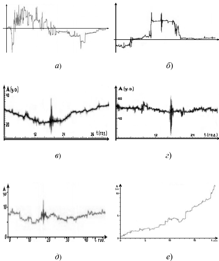
Рис. 2. Деформационные процессы в массиве горных пород РГС «Берегово» (Украинское Закарпатье) во время ряда землетрясений: a – в Турции 23.10.2011 г., M = 7,2 ; б – в Охотском море (около Сахалина) 14.08.2012 г., M = 7,7 ; в – на Аляске 5.01.2013 г., M = 7,8 ; г – в Эгейском море 8.01.2013 г., M = 5,8 ; д – в Чили 1.04.2014 г., M = 8,1 ; е – в период подготовки слабого ( M = 1,6 ) местного ( M = 18 км) землетрясения в Закарпатье (май 2014 г.)
