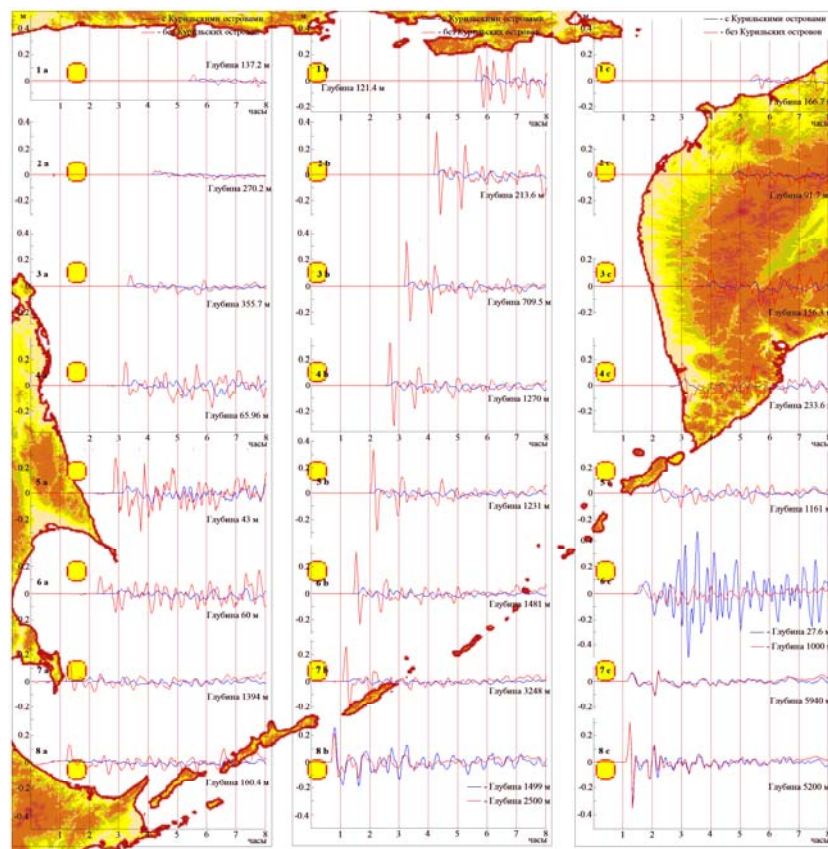
Рис. 2. Колебания уровня моря в различных точках Охотского моря по результатам моделирования с Курильскими островами и без них
