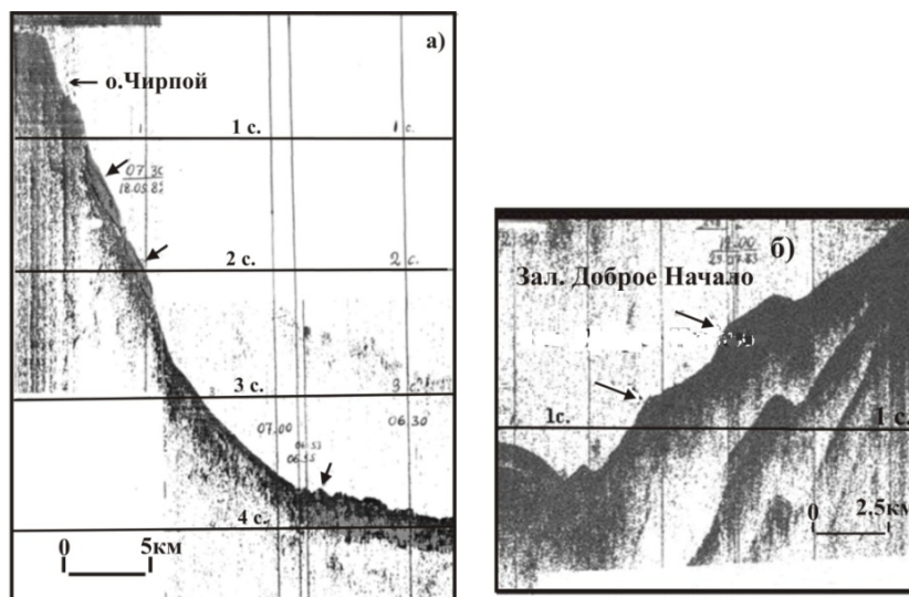
Рис. 1. Фрагменты профилей НСП, пересекающие: а – северный склон о. Чирпой; б – залив Доброе Начало
