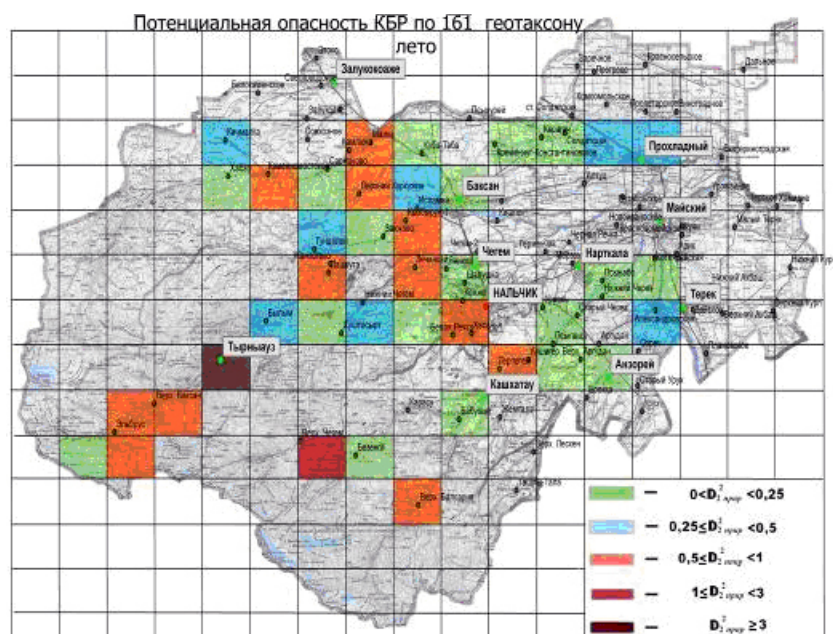
Рис 2. Сезонные (лето) численные оценки потенциальной экзогенной опасности территории КБР
