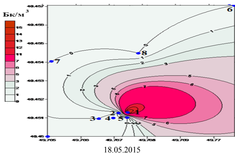
Рис. Карта (2D формат) распределения концентрации радона ( Rn ) на поверхности земли (пос. Масазыр, 2015 г.).
