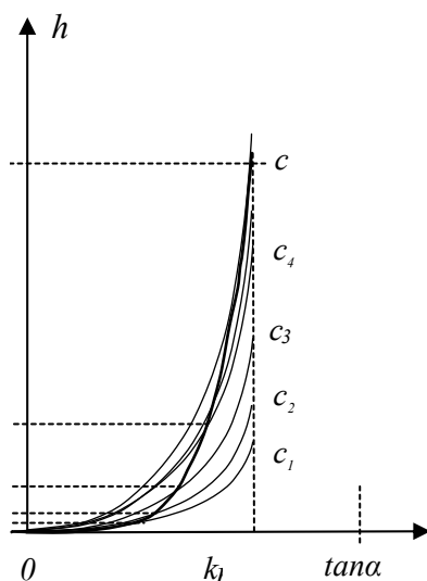
Рис. 2. Схематическая зависимость h_c(k, c)
