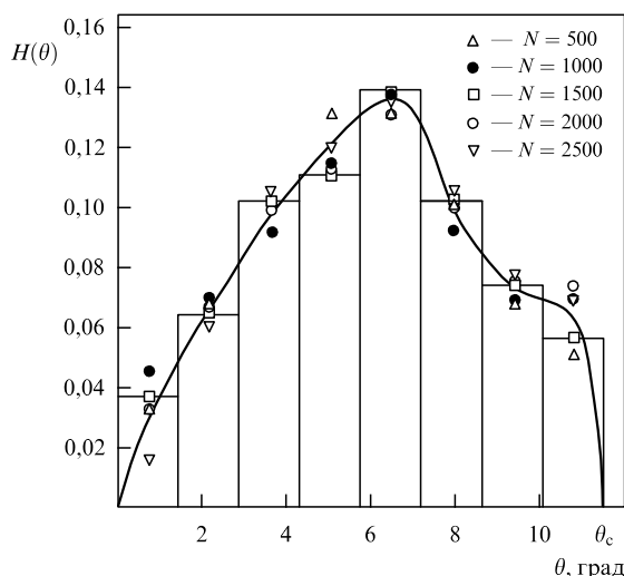
Рис. 9. Дискретные значения H(\theta_n) функции распределения по углам атаки, найденные при N = 500, 1000, 1500, 2000 и 2500 из нормированных гистограмм, подобных приведённой на рисунке для N = 1500 ; сплошной кривой показана аппроксимация функции H(\theta) , определённой в (28).
