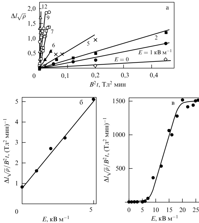
Рис. 4. Зависимости нормированного среднего пробега дислокаций \Delta l за время t экспозиции кристалла NaCl (Ca: 10 ppm) в магнитном B и электрическом E полях (а) от произведения B^2 t для нескольких значений E , указанных на рисунке, а также от поля E при его (б) низких, E < 5 \text{ кВ м}^{-1} , и (в) принадлежащих более широкому интервалу, E < 25 \text{ кВ м}^{-1} , величинах.
