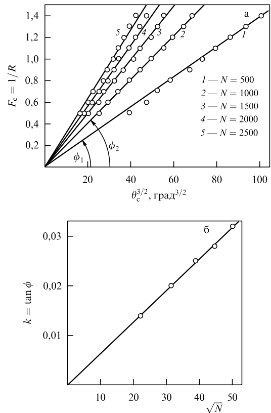
Рис. 7. Зависимости пороговой силы F_c (а) от критического угла атаки \theta_c и (б) от числа стопоров N в спрямляющих координатах, отвечающих формуле (36).
