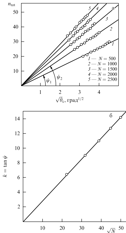
Рис. 8. Зависимость среднего числа n_{tot} стопоров на дислокации (а) от критического угла атаки \theta_c и (б) от числа стопоров N в спрямляющих координатах, отвечающих формуле (37).
