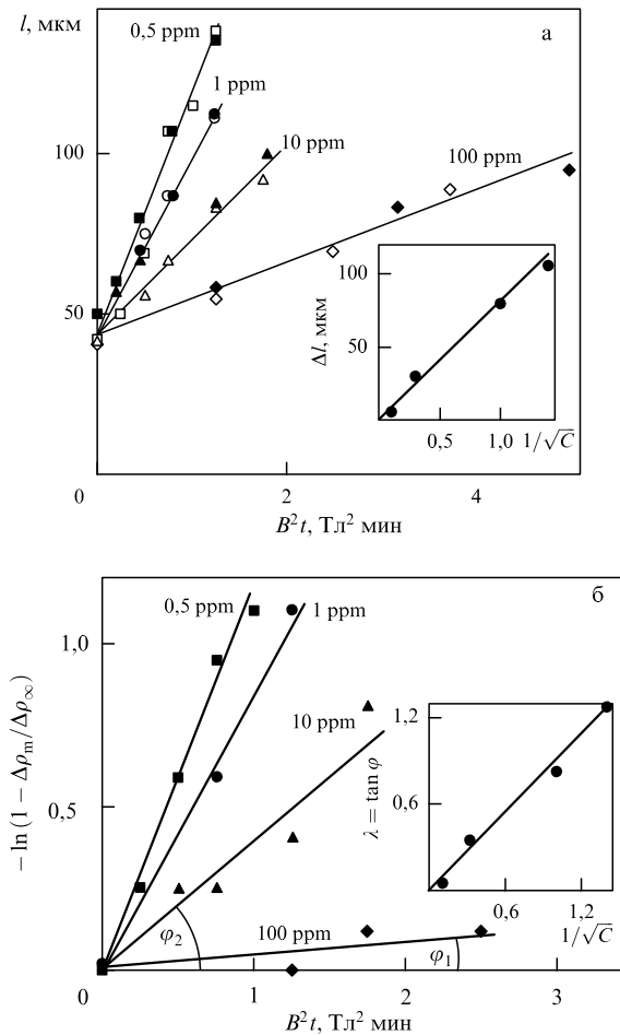
Рис. 1. Зависимости (а) средней длины пробега l и (б) относительной плотности \Delta\rho_m/\Delta\rho_\infty подвижных дислокаций в кристаллах NaCl(Ca) от величины магнитной индукции B и времени t выдержки образцов в магнитном поле ( B^2 t ). На вставках рис. а и б приведены соответственно зависимости приращения пробега \Delta l и наклон \lambda = \tan \varphi прямых (показанных на рис. б) от концентрации C примеси Ca при B = 0,5 Тл.
