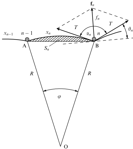
Рис. 5. Сила f_n , действующая на n -й стопор со стороны дислокации, \alpha_n и \theta_n — углы огибания и атаки соответственно, S_n — площадь, замечённая дислокацией перед её остановкой.
