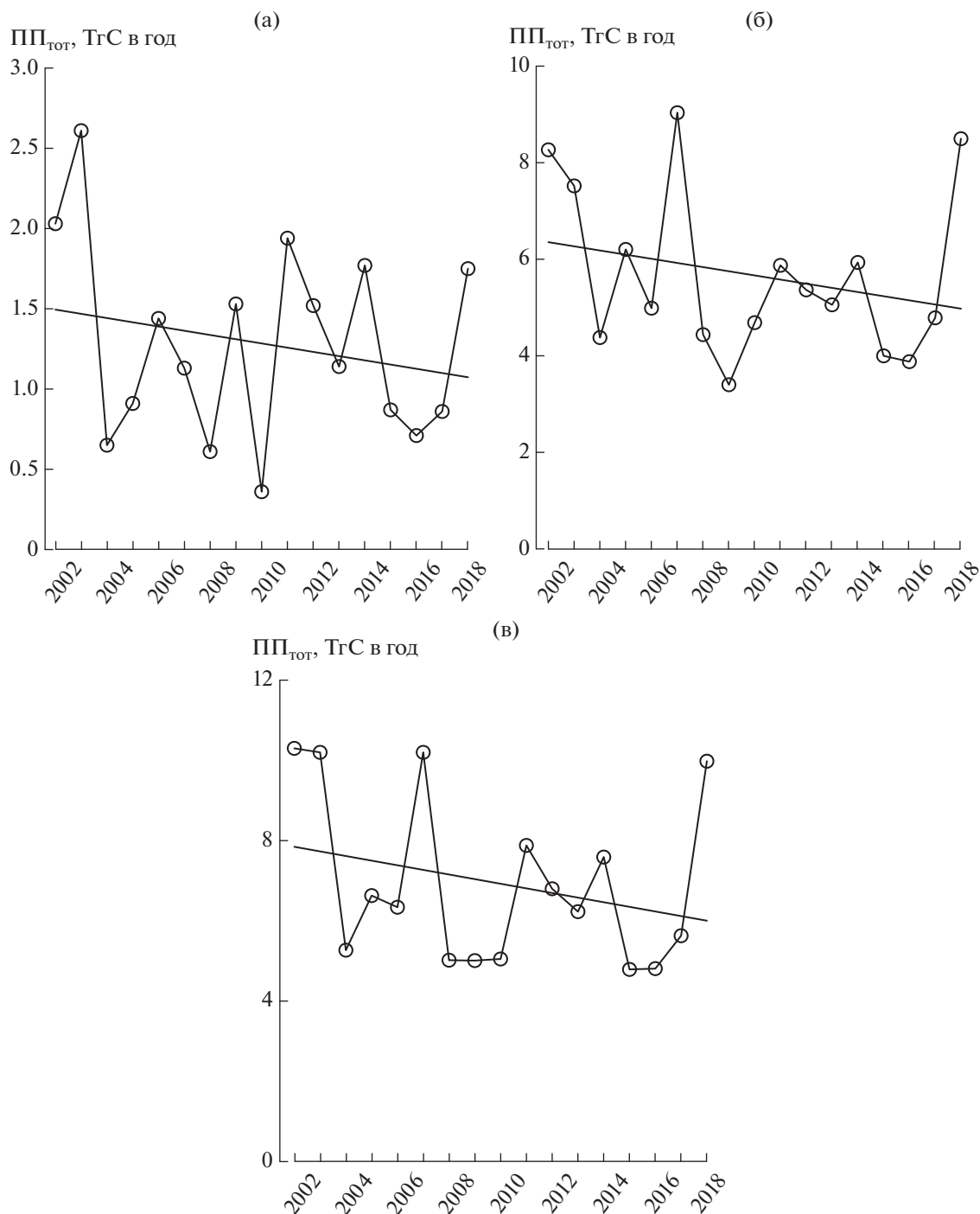
Рис. 5. Межгодовые изменения и линейные тренды первичной продукции ( PP_{\text{тот}} ), в различных районах моря Лаптевых в период с 2002 по 2018 гг. Обозначения районов см. в подписях к рис. 2.
