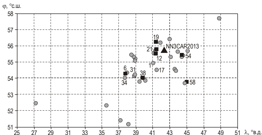
Рис. 2. Местоположение временной малоапертурной группы NN3CAR2013 (черный треугольник) и карьеров с идентифицированными взрывами (серые кружки). Черные квадраты – семь карьеров, использованных для анализа в данном исследовании
