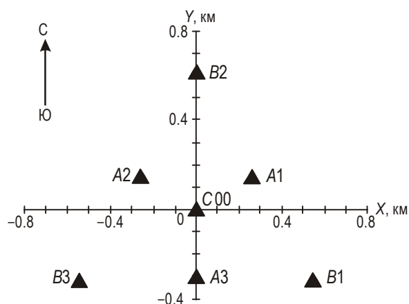
Рис. 1. Конфигурация временной малоапертурной группы NN3CAR2013, установленной в 2013 г. в Нижегородской области
