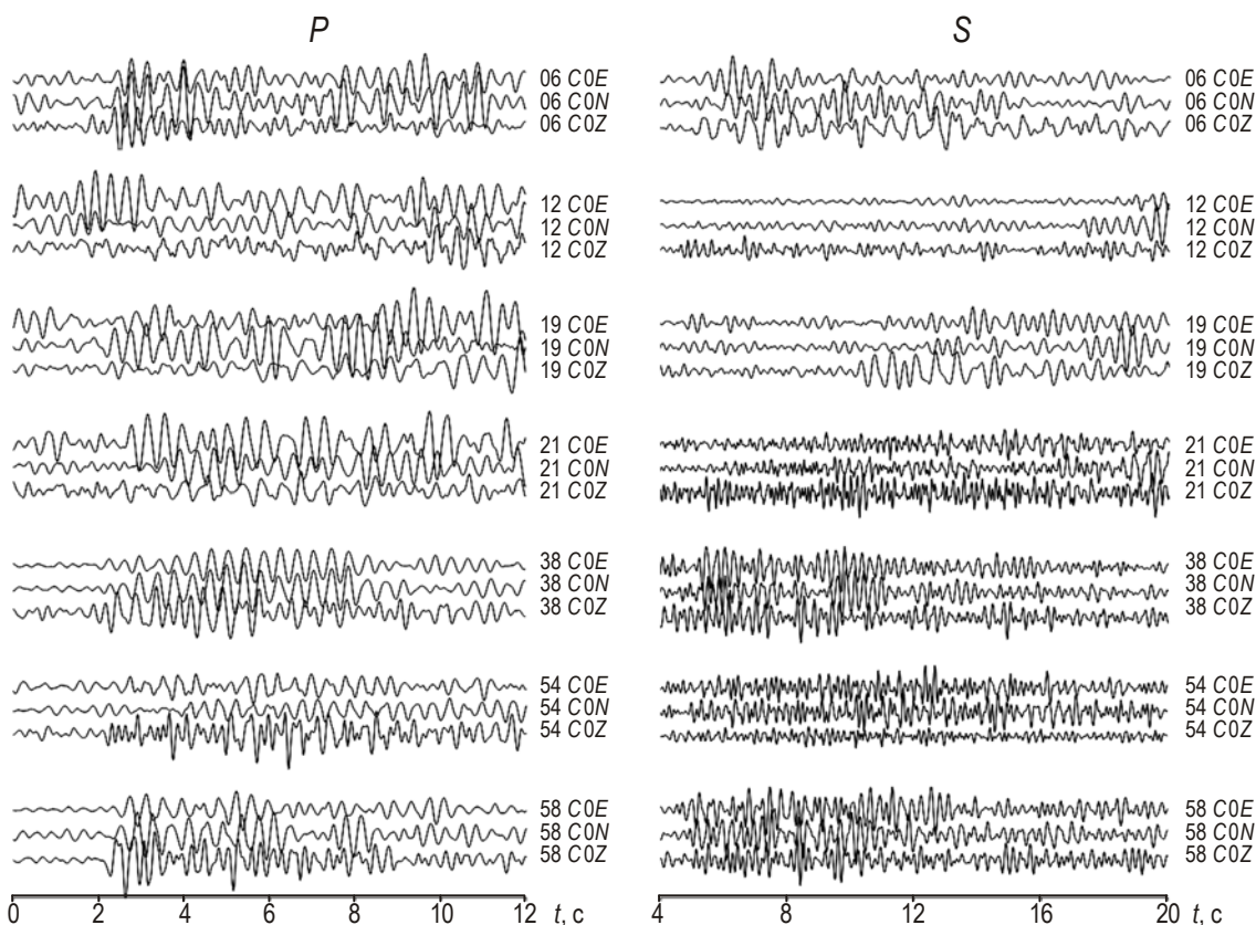
Рис. 3. Примеры шаблонов P - (слева) и S -волн (справа), сформированных по записям трёх компонент на центральной станции (C0E, C0N, C0Z) для карьеров №№ 6, 12, 19, 21, 38, 54, 58 (сверху вниз). Для S -волн показаны записи в интервале 4–20 с
