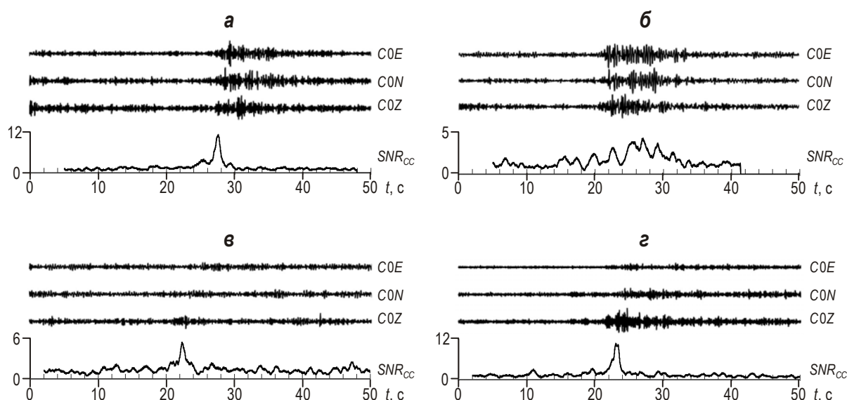
Рис. 4. Примеры обнаружения P -волны от взрывов с использованием метода КВФ. Карьер № 6. Трассы SNR_{CC} получены по 21 каналу
