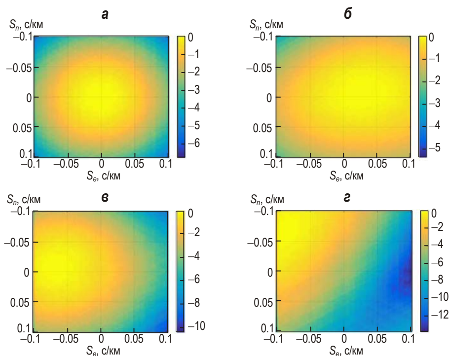
Рис. 6. Результаты FK -анализа, примененного к трассам коэффициента кросскорреляции шаблонов с различными фрагментами записей сигналов от карьера № 38. Пояснения см. в тексте
