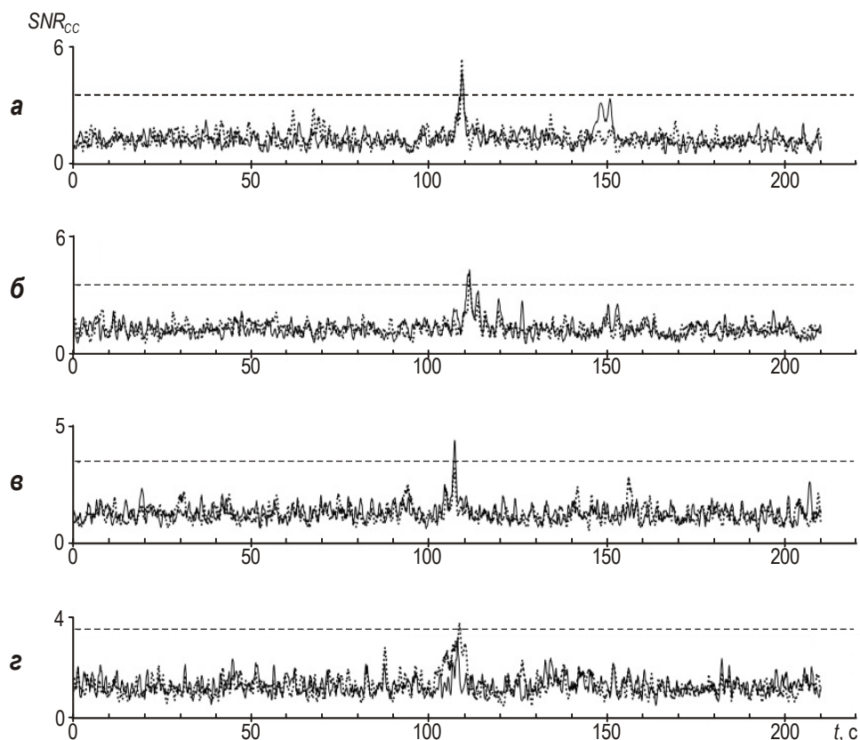
Рис. 5. Примеры обнаружения P -волны от взрывов в карьерах №№ 6 (а, б), 38 (в, г) с использованием метода КВФ. Трассы SNR , полученные по записям только вертикальных каналов – черные кривые, всех трёх каналов 3-С группы – серые. Установленный порог обнаружения SNR_{CC}=3.5 отмечен штриховой линией
