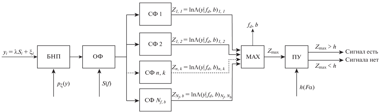
Рис. 1. Структурная схема асимптотически-оптимального обнаружителя для поиска моды Шлихтера в негауссовом шуме: ОФ – обеслаивающий фильтр; СФ – согласованный фильтр; МАХ – выбор максимального значения; ПУ – пороговое устройство.
