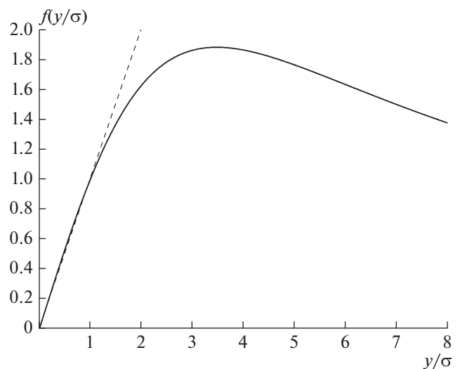
Рис. 2. Вид БНП для сейсмического шума Баксанского деформографа после Чилийского землетрясения (сплошная кривая). Пунктиром показана линейная функция в случае, если бы шум имел гауссовское распределение.
