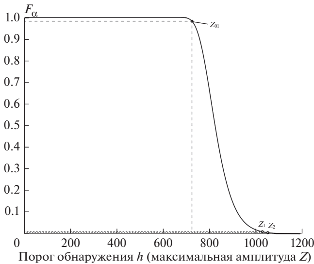
Рис. 6. Зависимость порога обнаружения и вероятности ложной тревоги.
