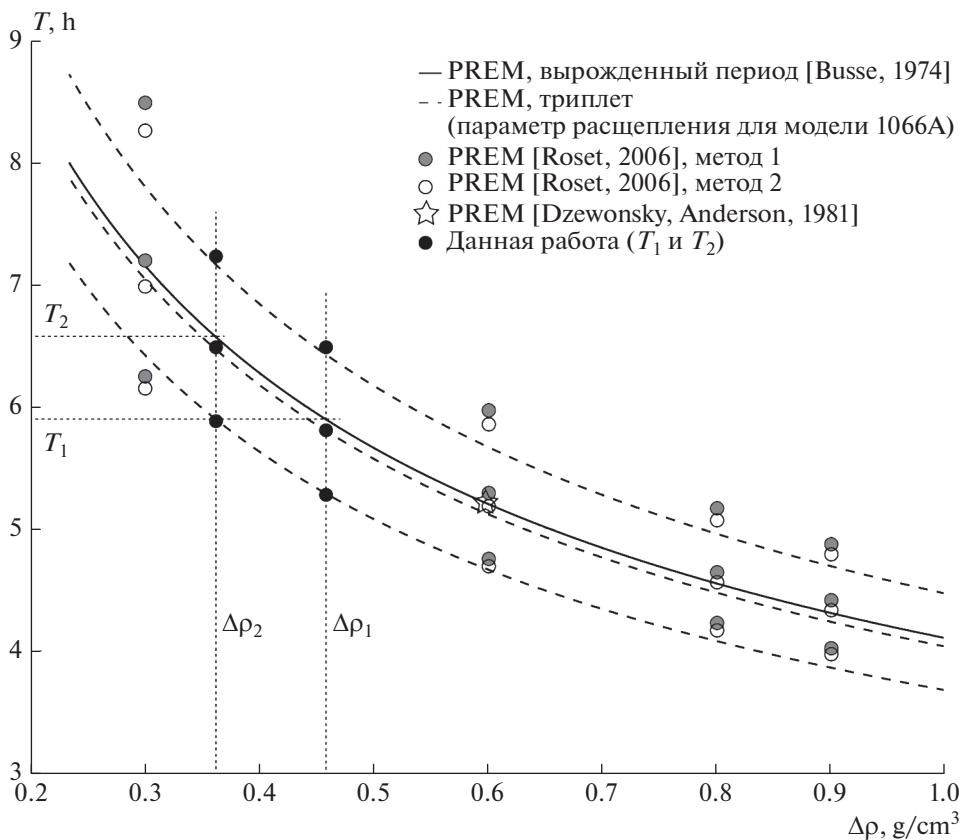
Рис. 7. Зависимость периода моды Шлихтера от скачка плотности между внутренним и внешним ядром Земли по различным источникам и результатам данной работы.
