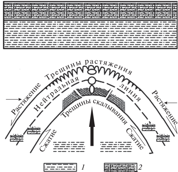
Рис. 3. Начальная фаза образования глиняного диавира: 1 – глины, обладающие свойствами неньютоновской жидкости; 2 – песчаник.
