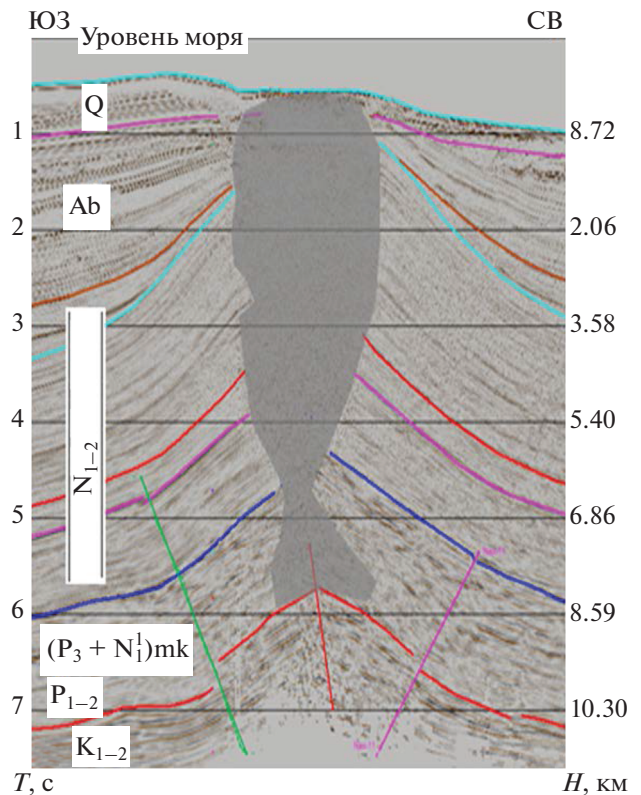
Рис. 4. Сечение эруптивного канала грязевого вулкана Нахчыван по данным трехмерной сейсморазведки.
