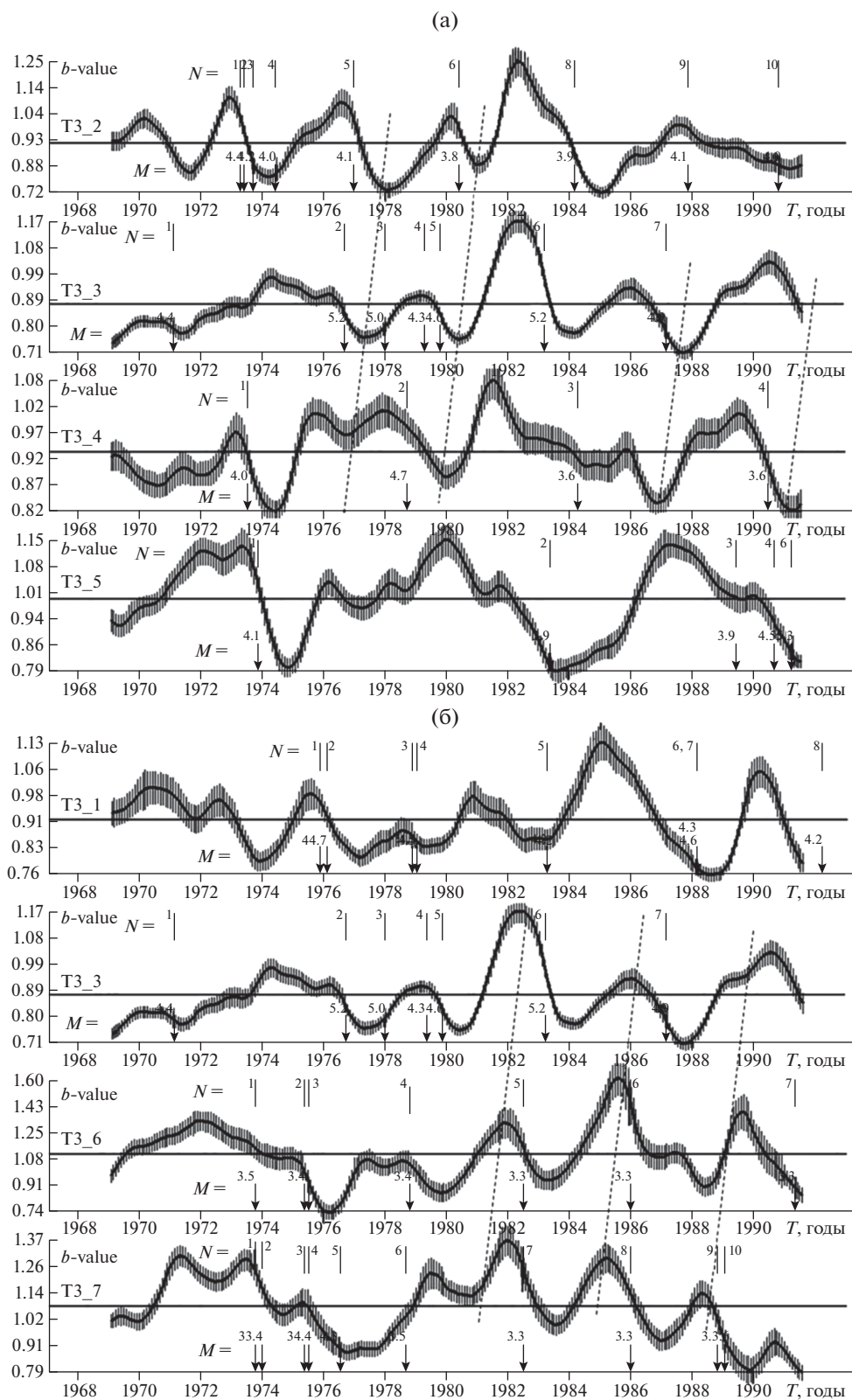
Рис. 7. (а) — Временные вариации b по данным землетрясений из ЛР (рис. 6), расположенных по простиранию геотектонических структур. Вертикальными стрелками отмечены моменты возникновения землетрясений с магнитудой M \geq 4.0 , произошедшие в пределах каждого ЛР. Цифры у стрелок соответствуют номерам землетрясений, приведенным в табл. 4. На кривых 70% доверительный интервал отмечен вертикальными отрезками. Пунктирными линиями обозначены возможные признаки перемещения фронта деформационных волн; (б) — временные вариации b -value по данным землетрясений из ЛР (рис. 6), расположенных вкрест простирания геотектонических структур. Условные обозначение те же, что и на рис. 7а.
