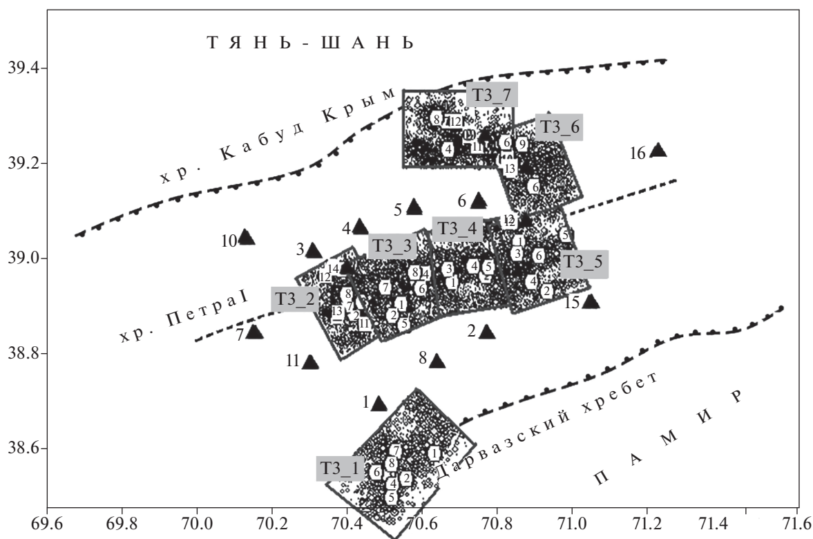
Рис. 6. Схема расположения локальных районов (ЛР) выборки данных землетрясений, расположенных по латеральному простиранию геотектонических структур. Условные обозначения те же, что и на рис. 1. Полые круги с номерами – эпицентры землетрясений с M \geq МПЗ внутри ЛР.
