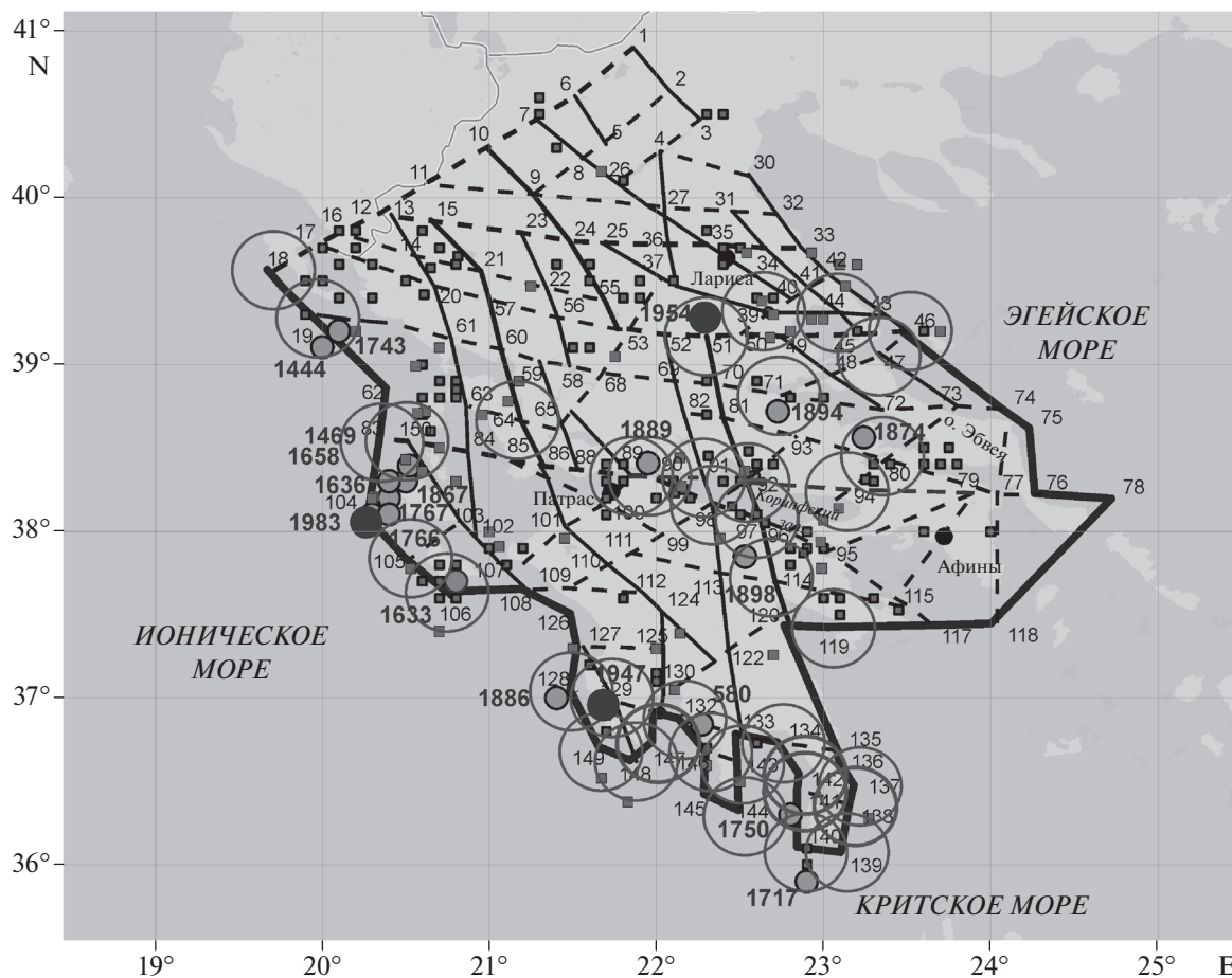
Рис. 2. Схема морфоструктурного районирования Эллинид и пересечения линейментов, отнесенные к классу В для M_w \geq 7.0 : Кругами отмечены высокосейсмические пересечения для M_w \geq 7.0 . Остальные обозначения те же, что и на рис. 1.
