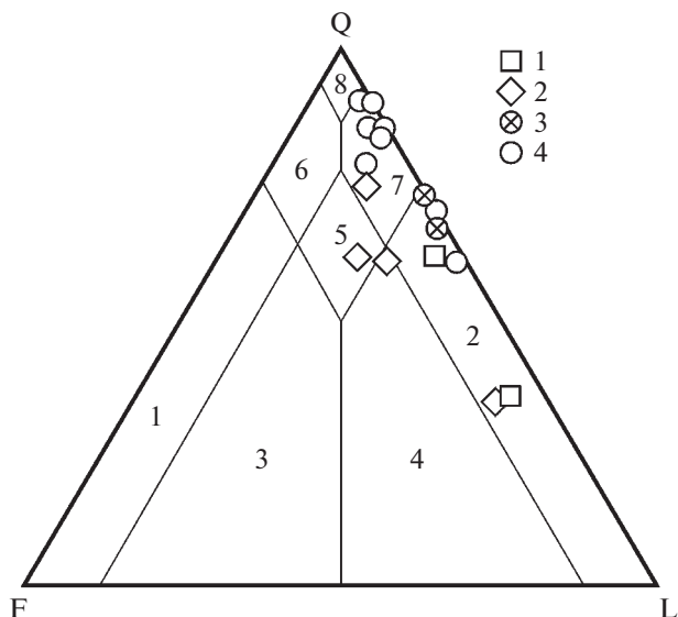
Рис. 5. Классификация песчаных разновидностей неопротерозойских и верхнепалеозойских отложений (McBride, 1963).
