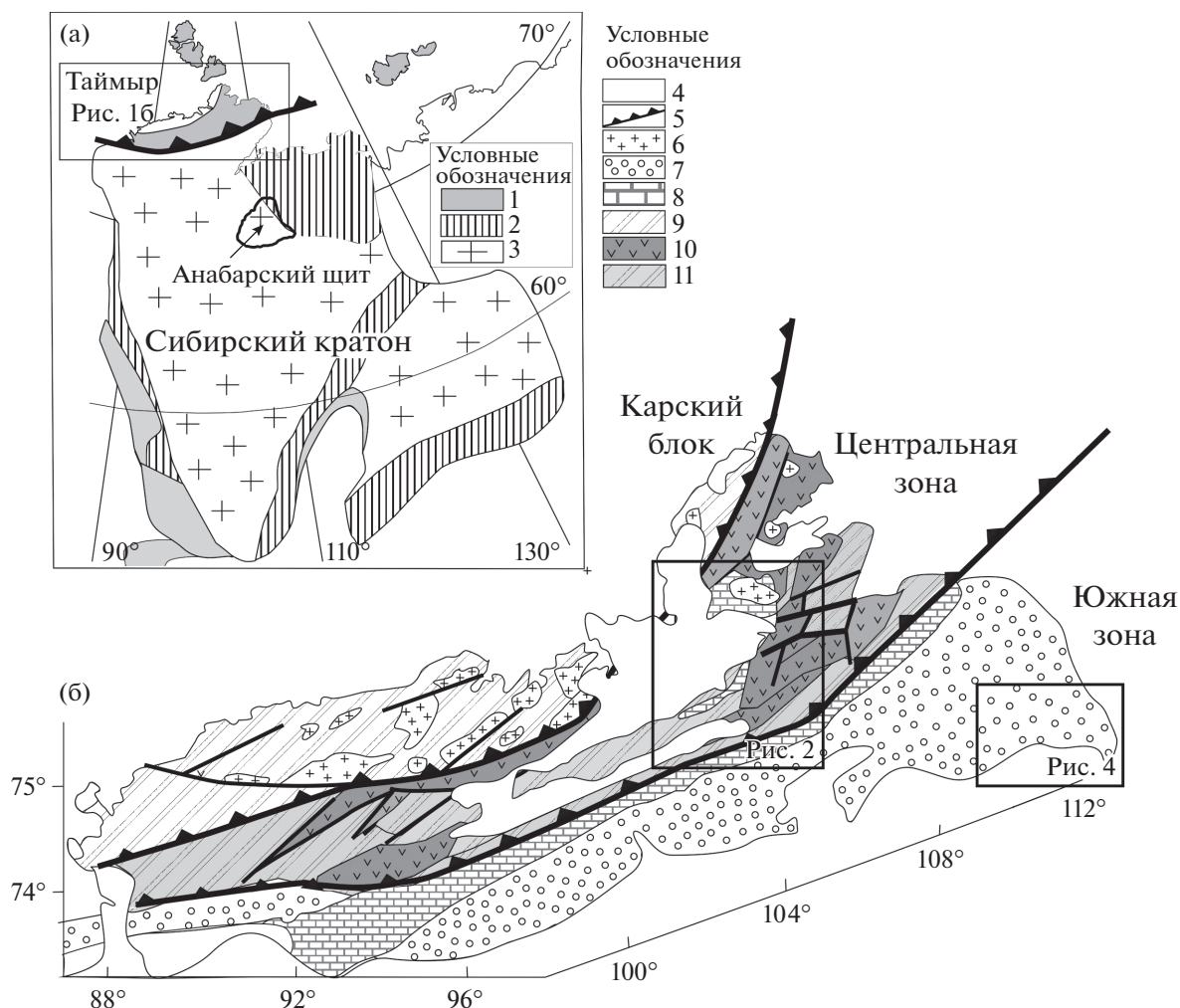
Рис. 1. (а) Основные тектонические единицы фундамента Сибирского кратона с обрамлением (по Розен, 2003) и (б) строение Таймырского складчато-надвигового пояса (по Верниковский, 1996; Vernikovskiy, Vernikovskaya, 2001). 1 – неопротерозойские складчатые пояса; 2 – палеопротерозойские складчатые пояса; 3 – архейская континентальная кора; 4 – мезозойско-кайнозойский чехол; 5 – главные надвиги; 6 – граниты с возрастом 300–250 млн лет; 7 – верхнепалеозойский терригенный комплекс; 8 – палеозойские известняки и сланцы; 9 – турбидиты неопротерозойского и раннекембрийского возраста; 10 – неопротерозойские офиолиты и островодужные комплексы; 11 – неопротерозойские терригенные и карбонатные осадочные комплексы.
