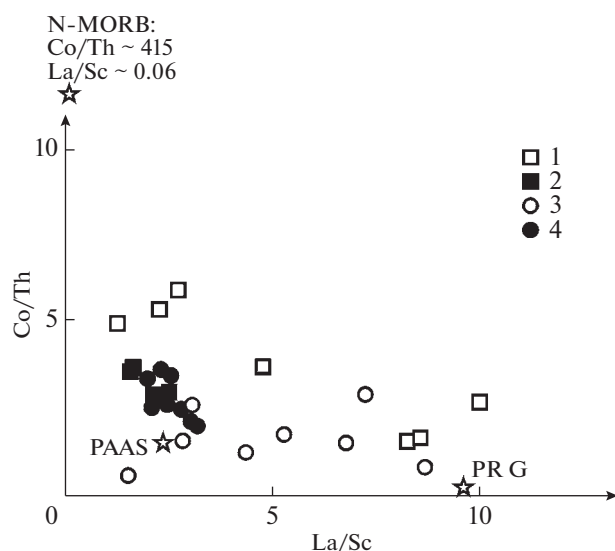
Рис. 8. Диаграмма соотношения Co/Th и La/Sc в терригенных породах неопротерозоя и верхнего палеозоя восточного Таймыра, позволяющая реконструировать состав пород в источнике сноса.
