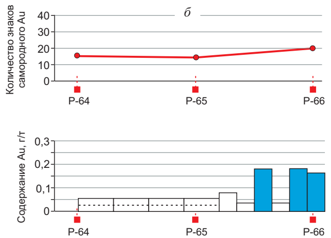
Рис. 8. ОРТО-САЛА-ВЕРХНЕКУРАНАХСКОЕ РУДНОЕ ПОЛЕ. СОТНОШЕНИЕ РАСПРЕДЕЛЕНИЯ ЭЛЮВИАЛЬНОГО ШЛИХОВОГО ЗОЛОТА ИЗ РАСЧИСТОК (зона разборного плотика) И СОДЕРЖАНИЙ ЗОЛОТА ПО ДАННЫМ ПРОБИРНОГО АНАЛИЗА В БК-100 (а) И БК-101 (б)
