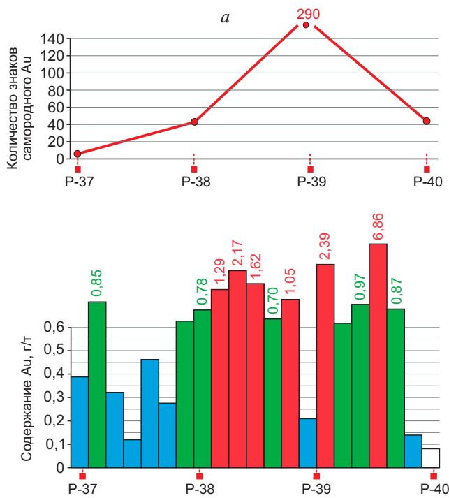
Рис. 8. ОРТО-САЛА-ВЕРХНЕКУРАНАХСКОЕ РУДНОЕ ПОЛЕ. СОТНОШЕНИЕ РАСПРЕДЕЛЕНИЯ ЭЛЮВИАЛЬНОГО ШЛИХОВОГО ЗОЛОТА ИЗ РАСЧИСТОК (зона разборного плотика) И СОДЕРЖАНИЙ ЗОЛОТА ПО ДАННЫМ ПРОБИРНОГО АНАЛИЗА В БК-100 (а) И БК-101 (б)
