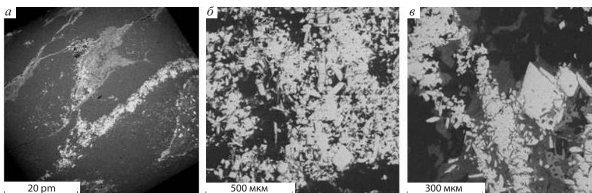
Рис. 4. РУДНАЯ МИНЕРАЛИЗАЦИЯ ЗАПАДНОГО УЧАСТКА РУДОПРОЯВЛЕНИЯ РАЯЛАМПИ:
